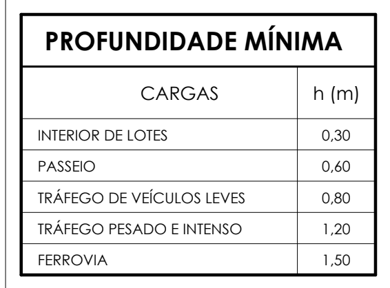
DETALHE DE VALA PARA TUBULAÇÃO ENTERRADA
