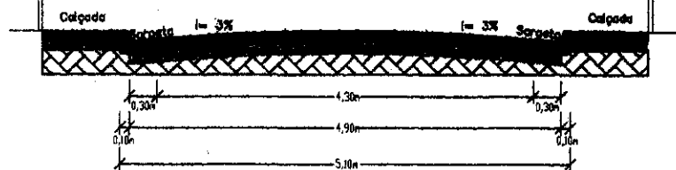
Perfil Transversal Seção Tipo
