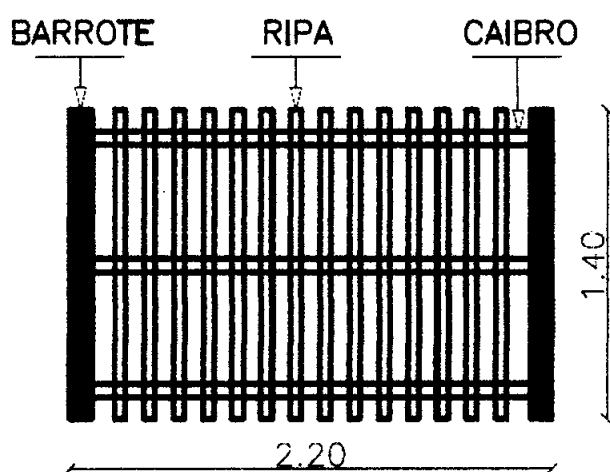
DETALHE DO PORTÃO DE MADEIRA
