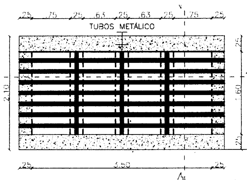
DETALHE LOCALIZAÇÃO DOS TUBOS METÁLICO (GRADE)
