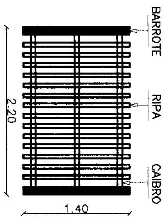
DETALHE DO PORTÃO DE MADEIRA
