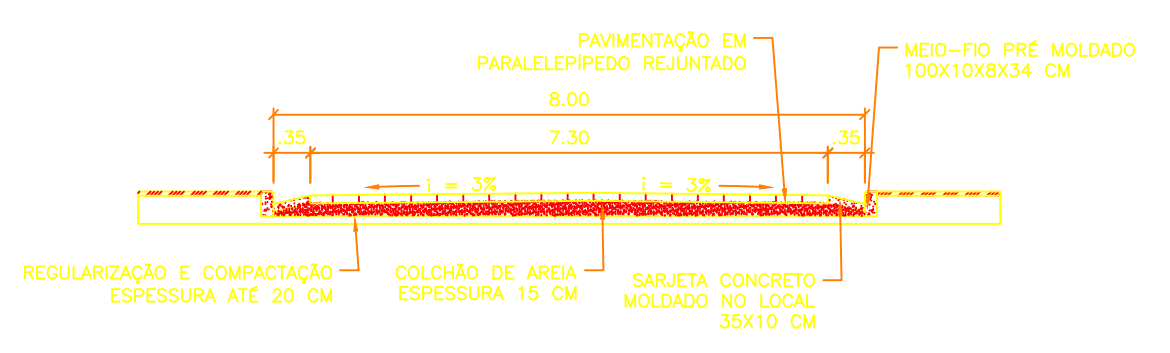
02 SEÇÃO TRANSVERSAL ESCALA 1:75
