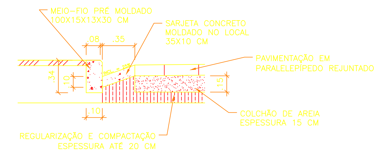
03 DETALHE DO MEIO-FIO E SARJETA ESCALA 1:25
