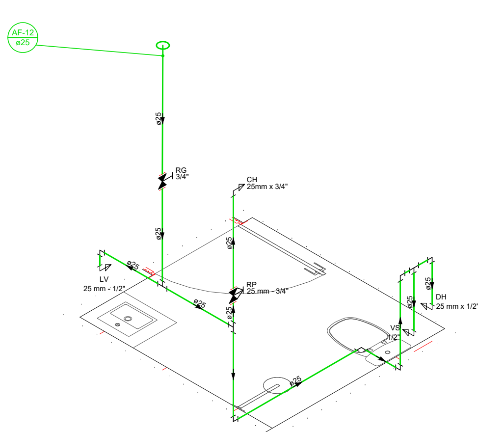
DETALHE HID-16 1:25
