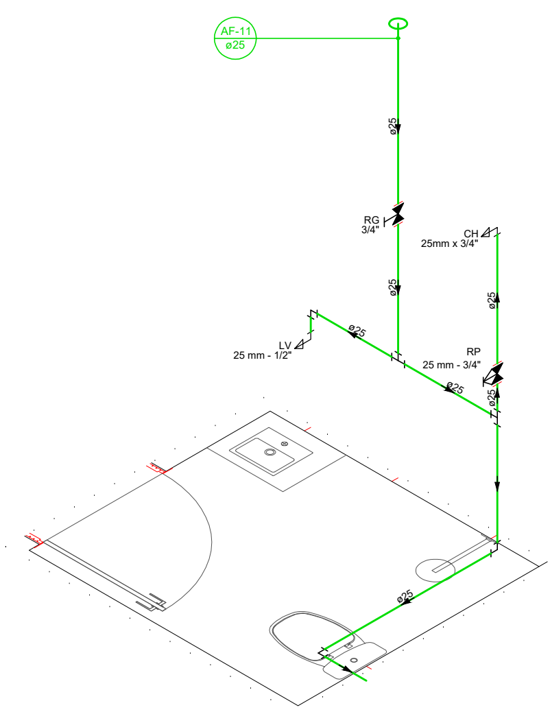
DETALHE HID-15 1:25
