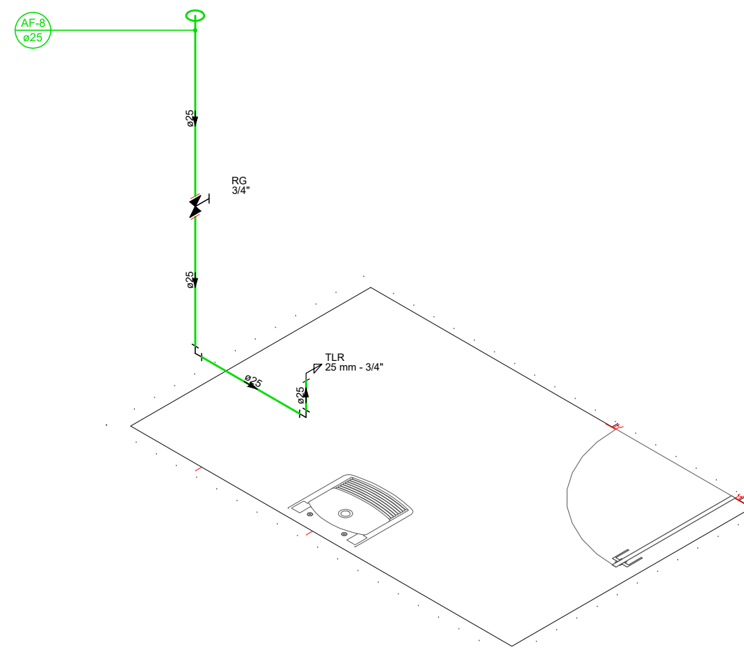
DETALHE HID-12 1:25
