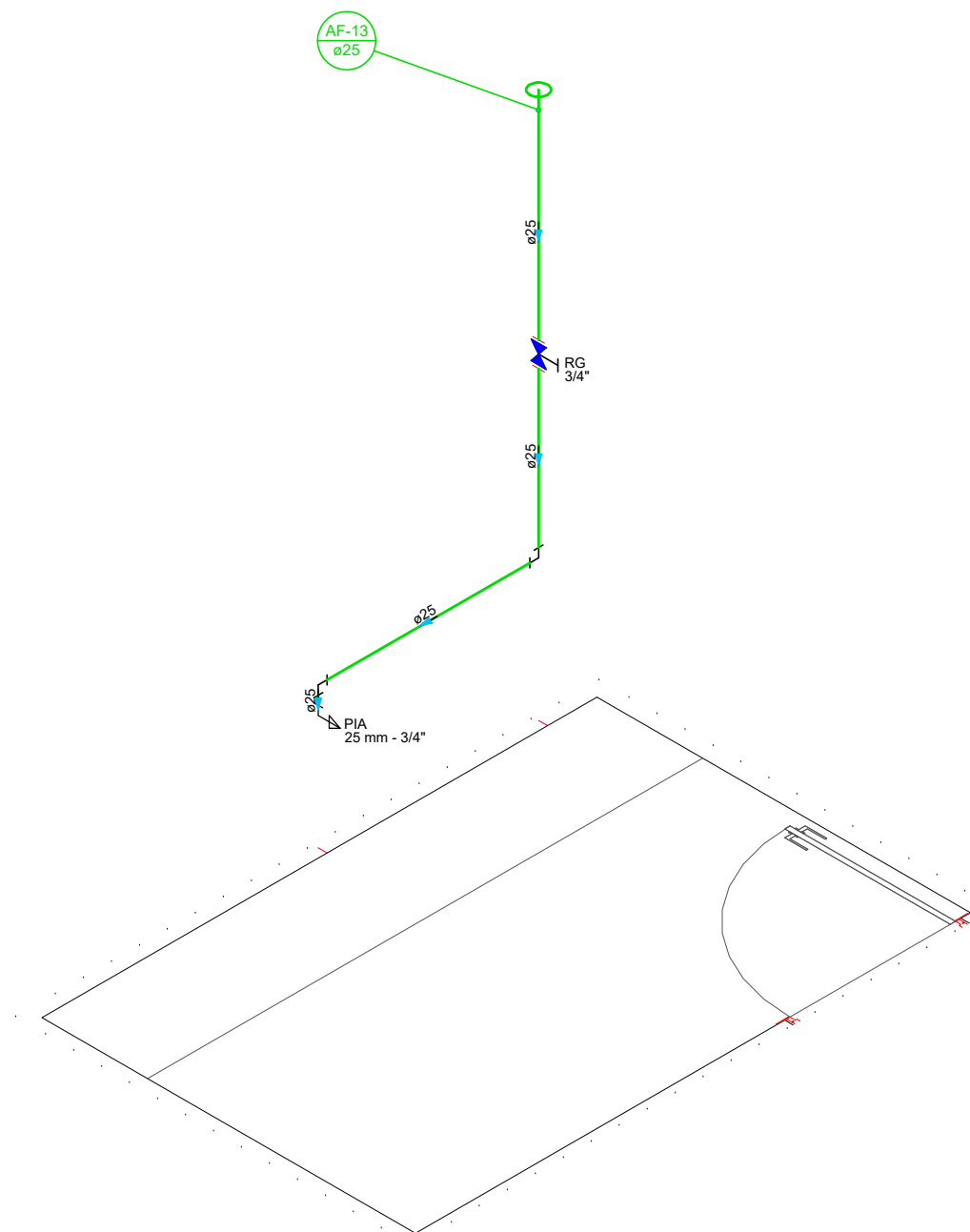
DETALHE HID-6 1:25
