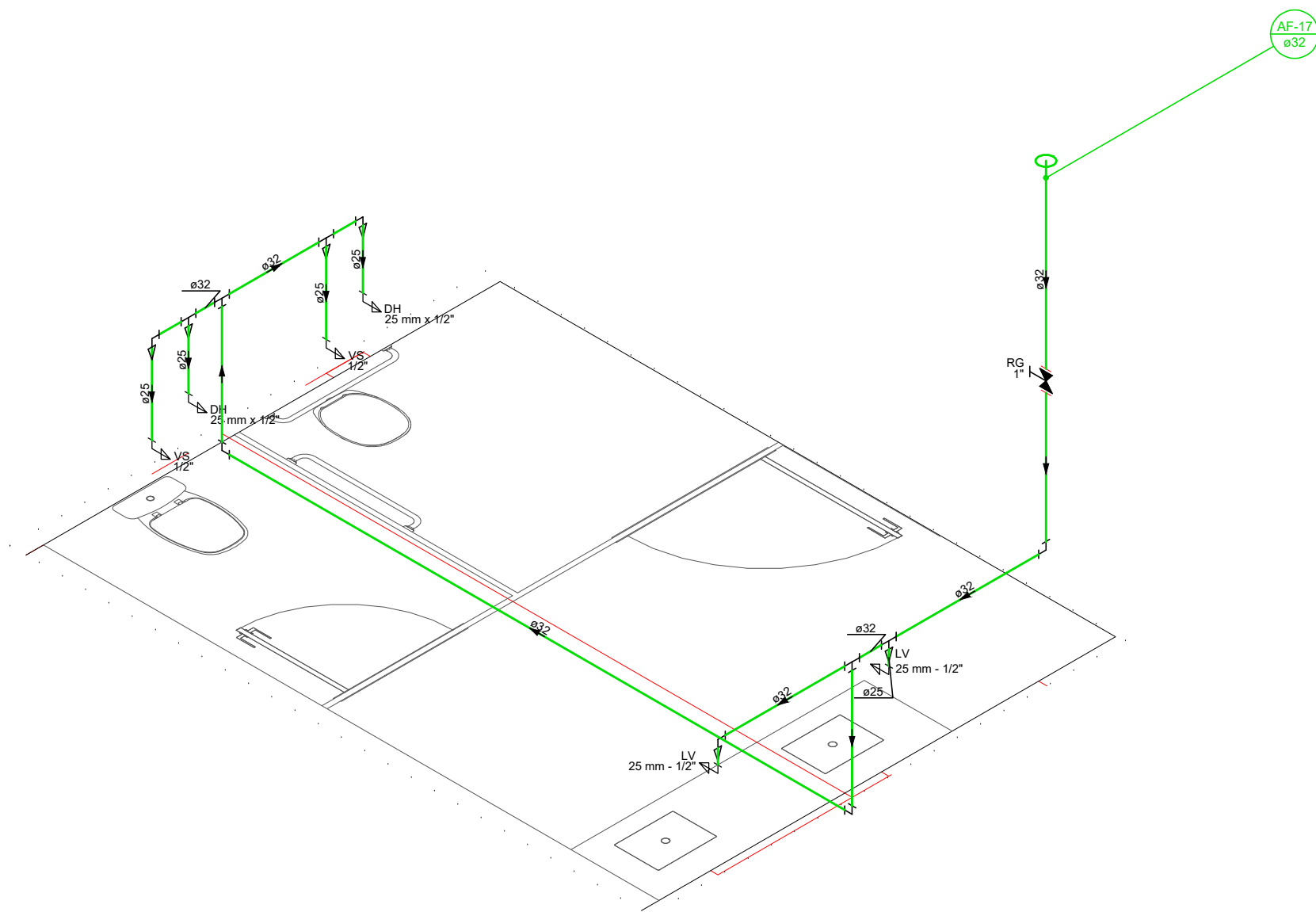
DETALHE HID-14 1:25
