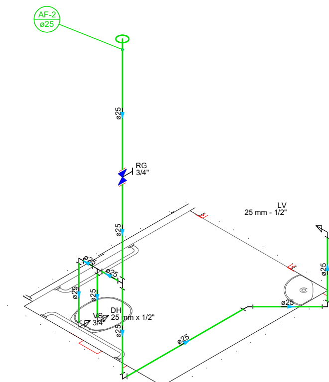
DETALHE HID-3 1:25
