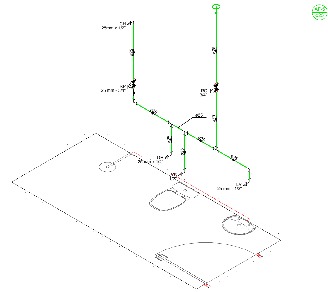
DETALHE HID-11 1:25
