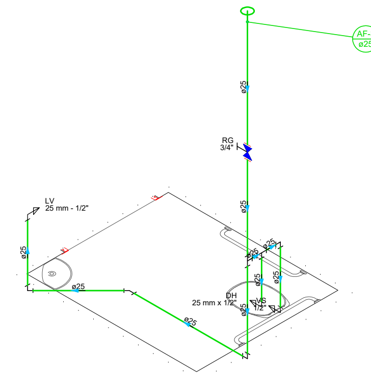
DETALHE HID-4 1:25
