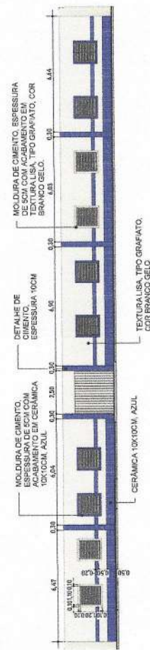
2 FACHADA SENHORINHA Escala - 1:100
