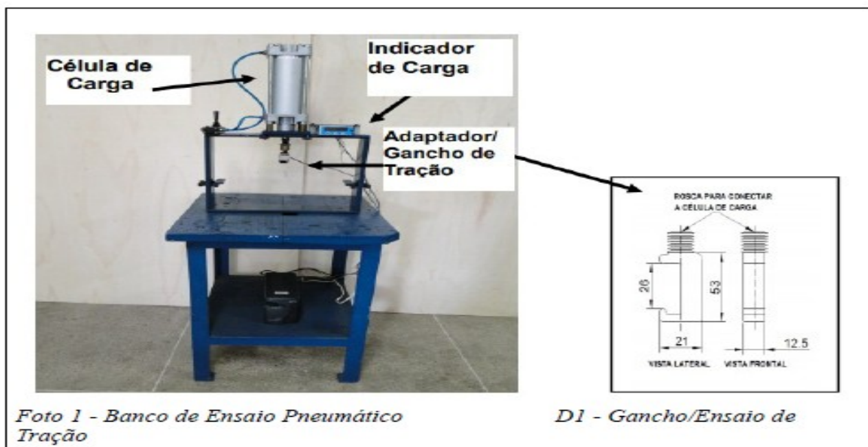
Foto 1 - Banco de Ensaio Pneumático
