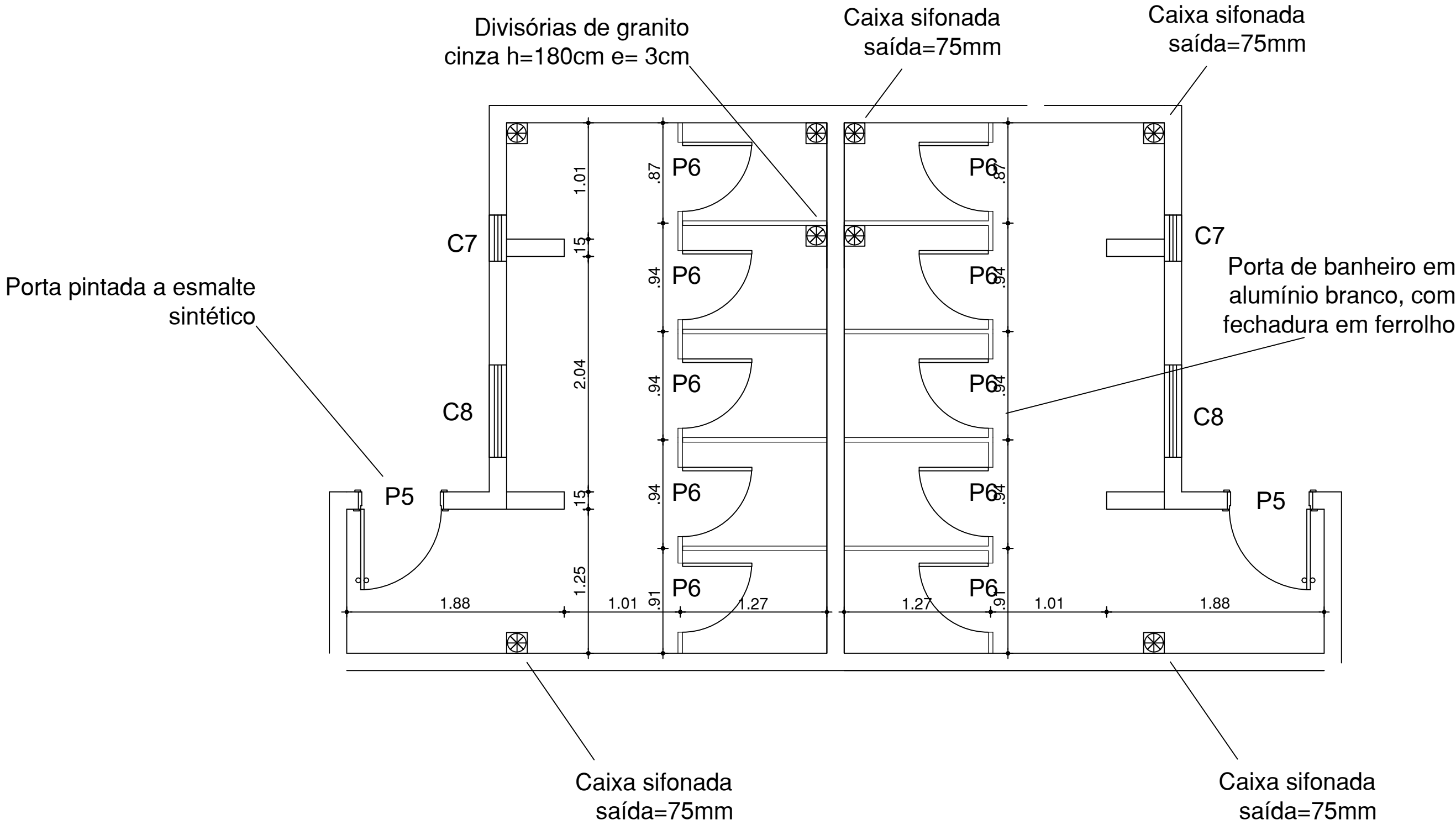
02 | ALVENARIAS E DIVISÓRIAS WC's ESCALA : 1/50
