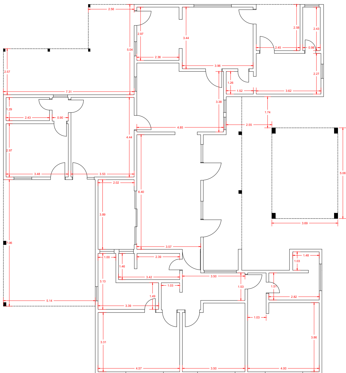
PLANTA BAIXA - MEDIDAS INTERNAS ESC. SEM ESCALA
