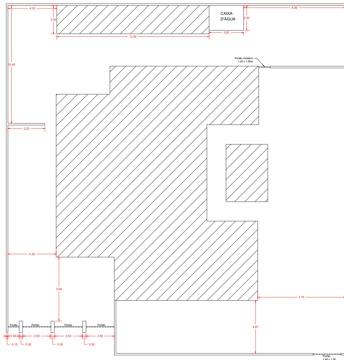
PLANTA BAIXA - MEDIDAS EXTERNAS ESC. SEM ESCALA
