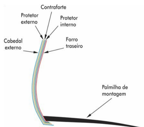
FIGURA: Desenhos das camadas de materiais do calcanhar. (Figura meramente ilustrativa)
