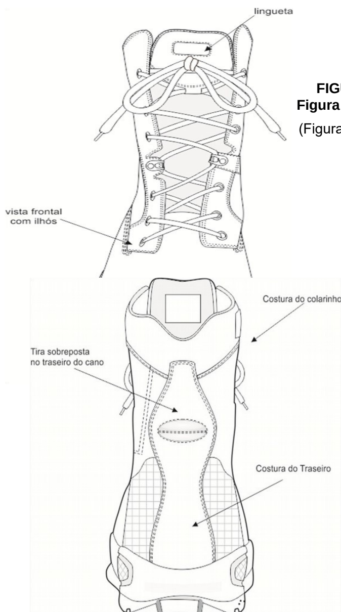
FIGURA: Vista traseira - Figura Meramente Ilustrativa (Figura meramente ilustrativa)
