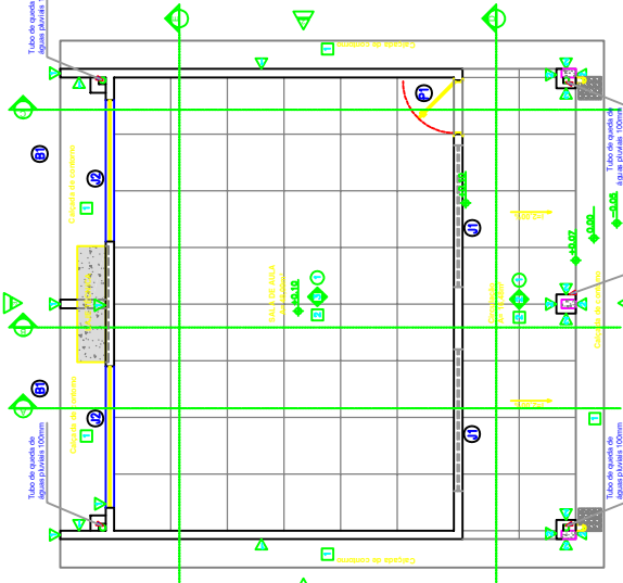
02 | PL. DE LEGENDAS ESCALA 1:50
