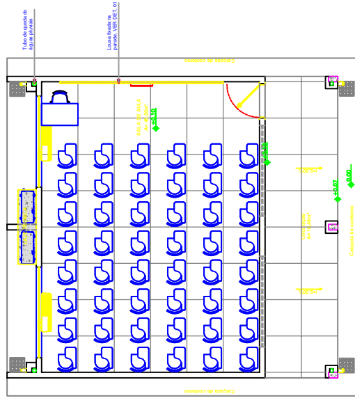
05 | PL. DE LAYOUT ESCALA 1:50
