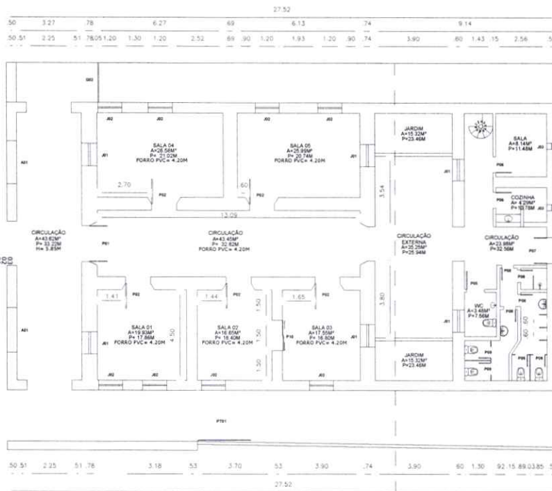
01 PLANTA BAIXA 1/125
