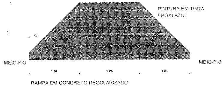
01. PL. RAMPA ACESSÍVEL 1/30
