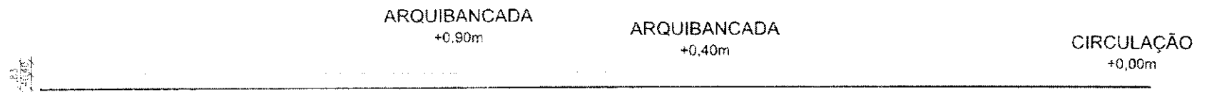
01 CORTE C - ARQUIBANCADA 1/100
