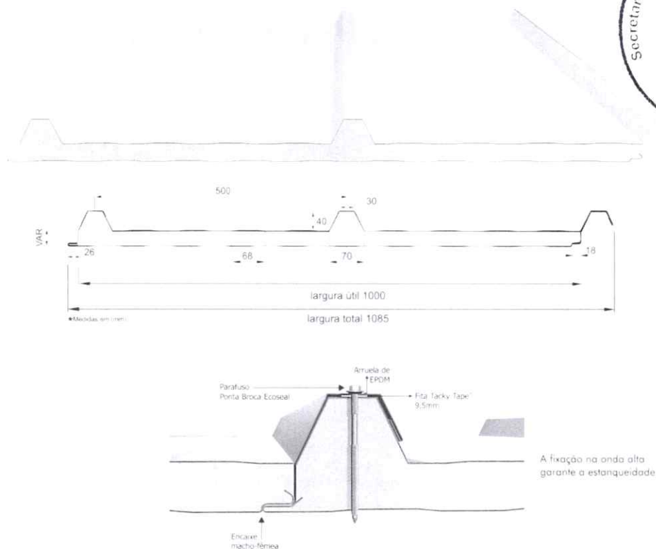
Figura 10 – imagem telha termoacústica
