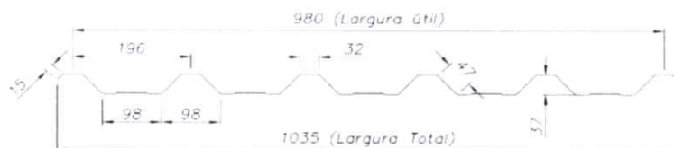
Figura 11 – imagem telha metálica trapezoidal TP40-980
