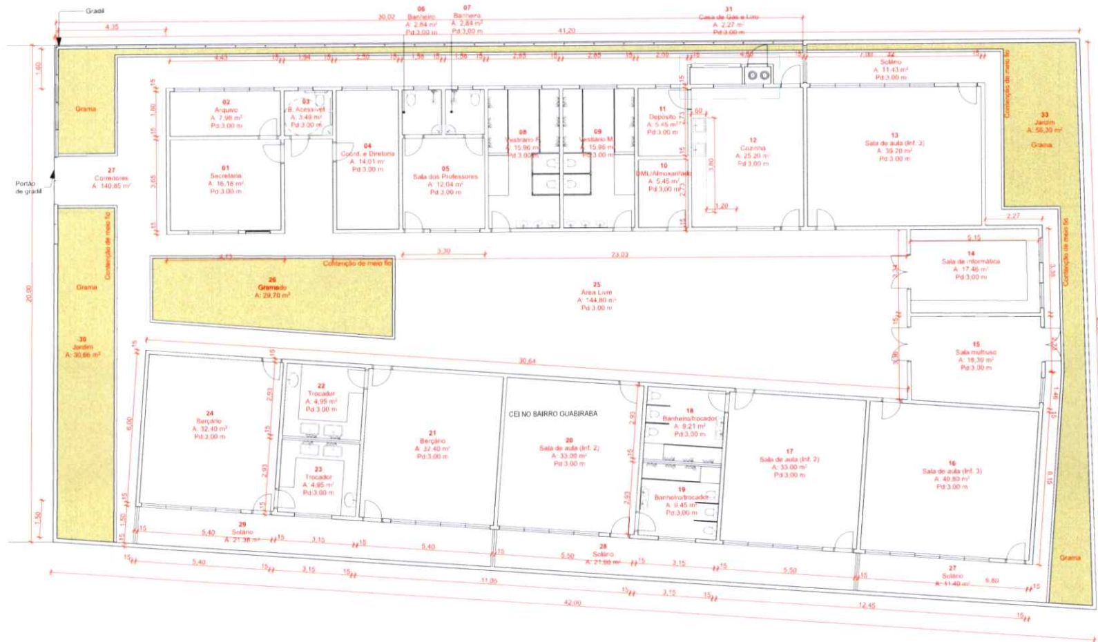
1 | Planta baixa geral 1:100
