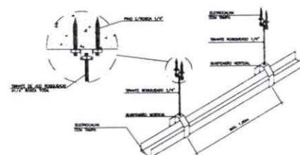
DETALHE DE FIXAÇÃO DAS ELETROCALHAS SEM ESCALA
