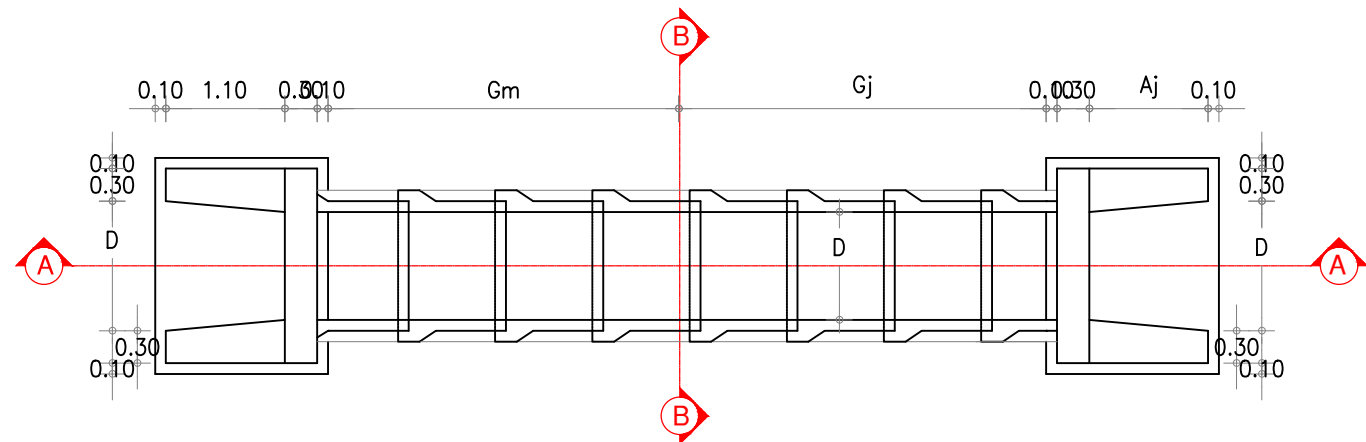
PLANTA BAIXA
