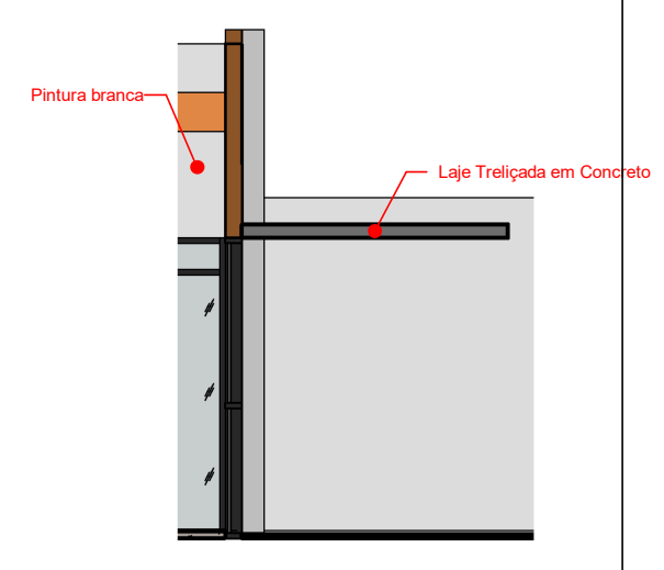
4 a-a 1 : 75
