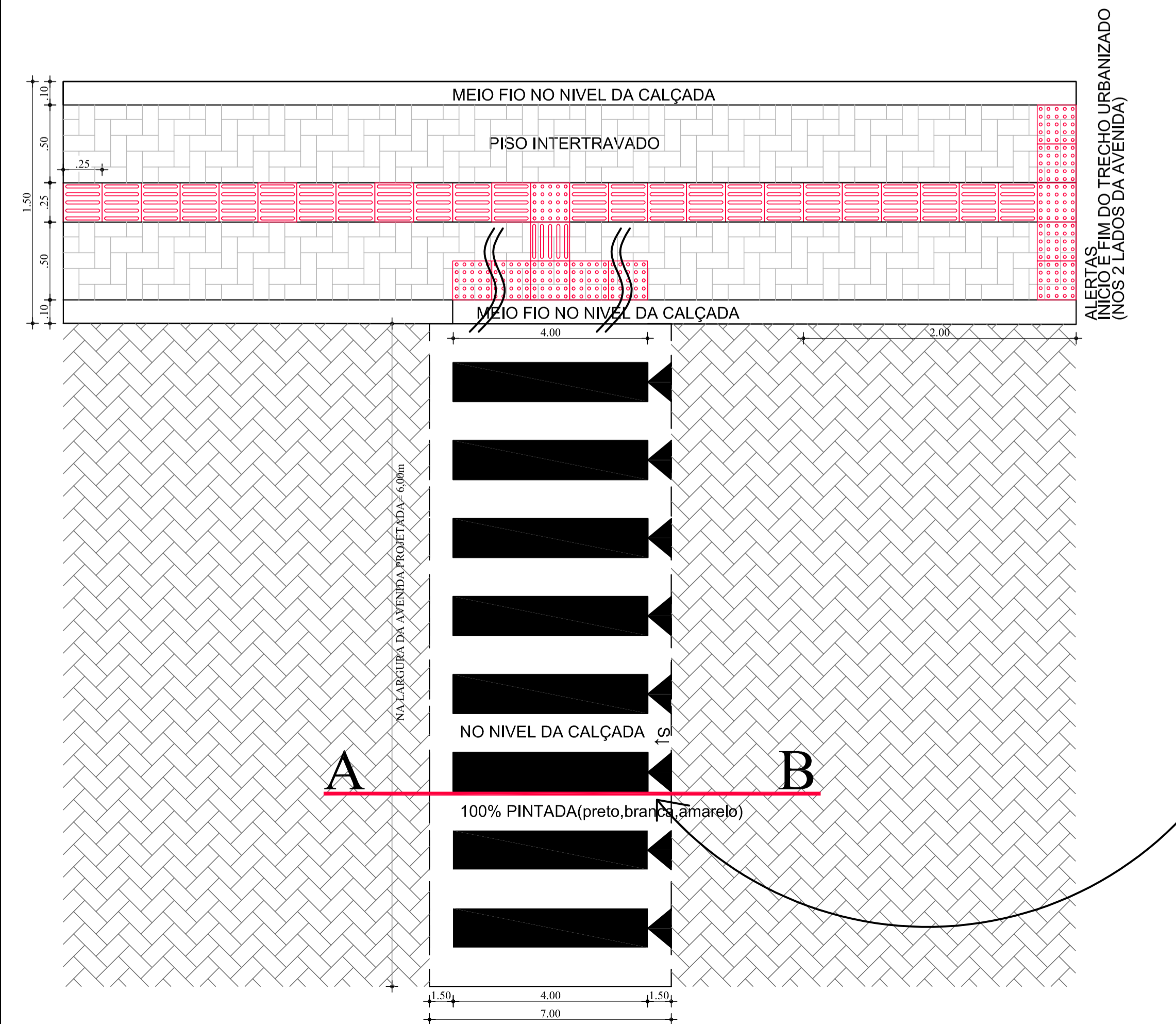
03 PASSARELAS ELEVADAS EM CONCRETO ESCALAS = SEM
