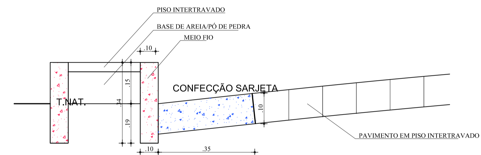
06 DETALHE SARGETA ESCALAS = SEM
