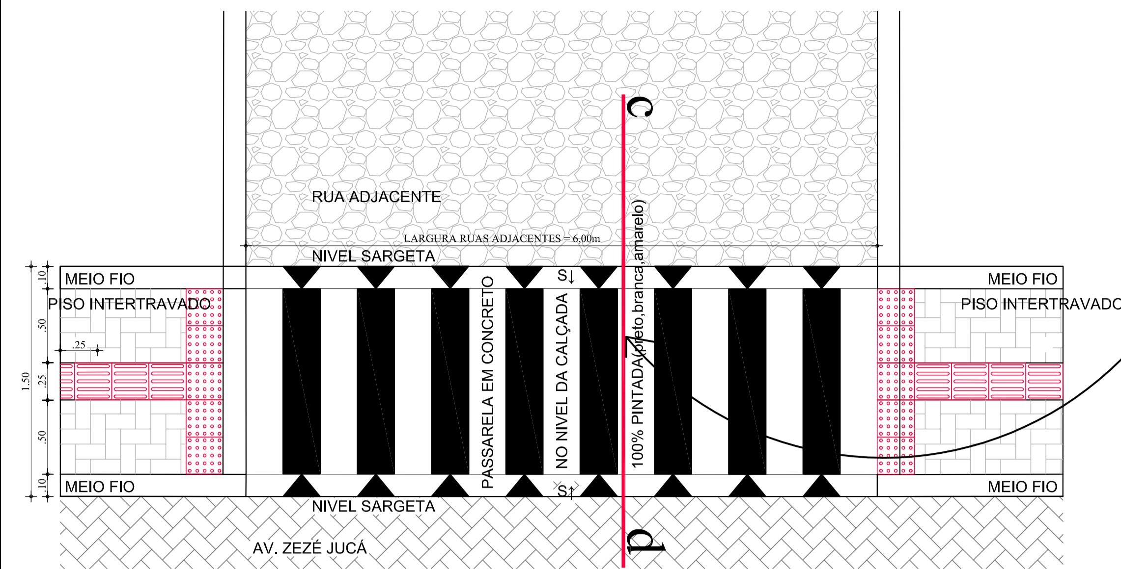
01 CRUZAMENTOS DA AVENIDA PROJETADA COM AS RUAS ADJACENTES (ESQUINAS) ESCALAS = SEM
