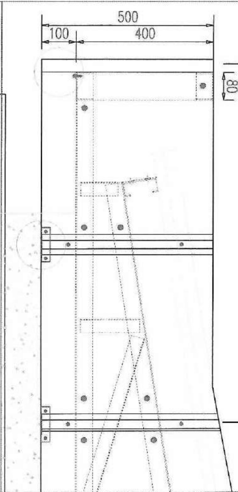
8" - DETALHE TIPO PARA OS TRAVEÇOS DE GIZO
