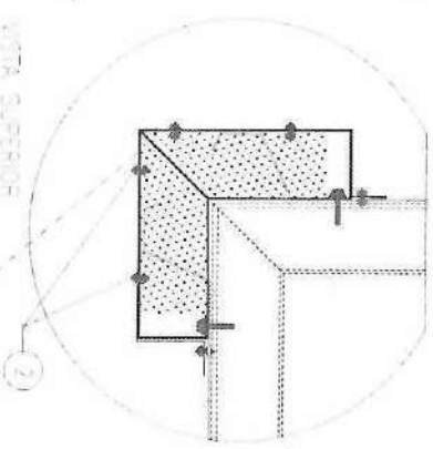
7" - DETALHE TIPO PARA CANTOS
