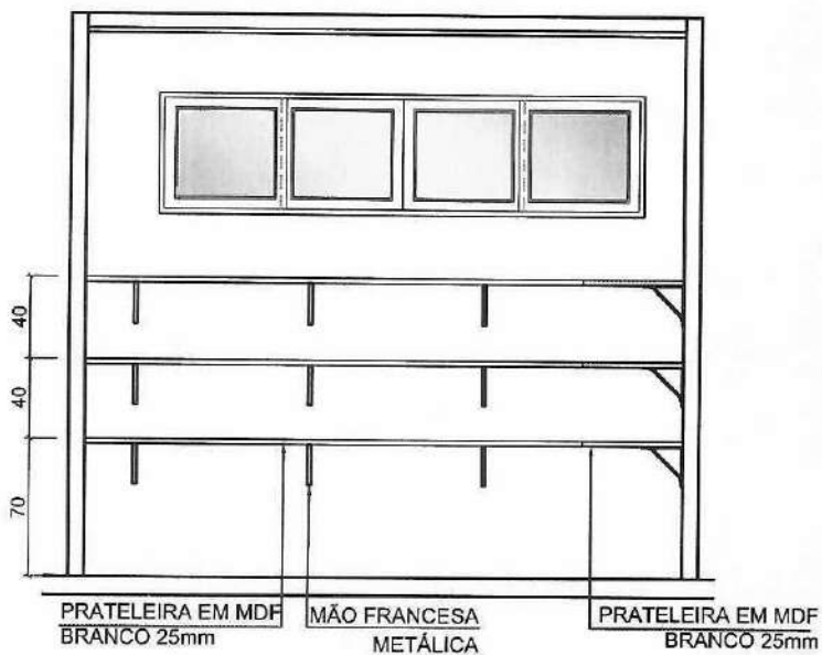
02 ELEVÇÃO A ESCALA 1:40
