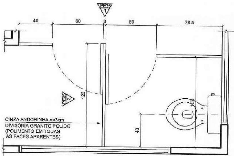
01 PLANTA ESCALA 1:25
