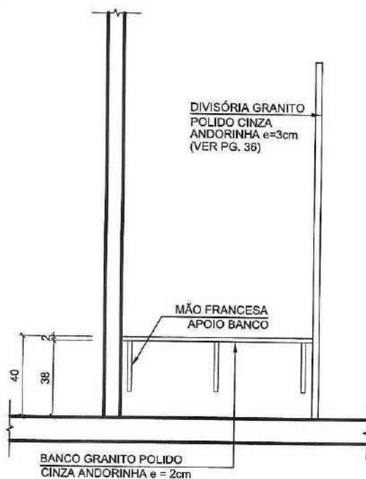
03 B21 - ELEVÇÃO ESCALA 1:25
