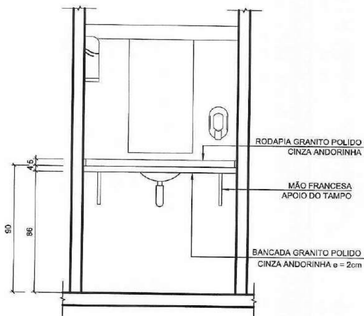
04 B10 - ELEVÇÃO ESCALA 1:25
