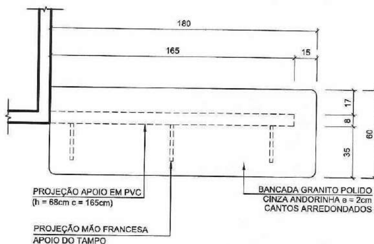
01 PLANTA ESCALA 1:25
