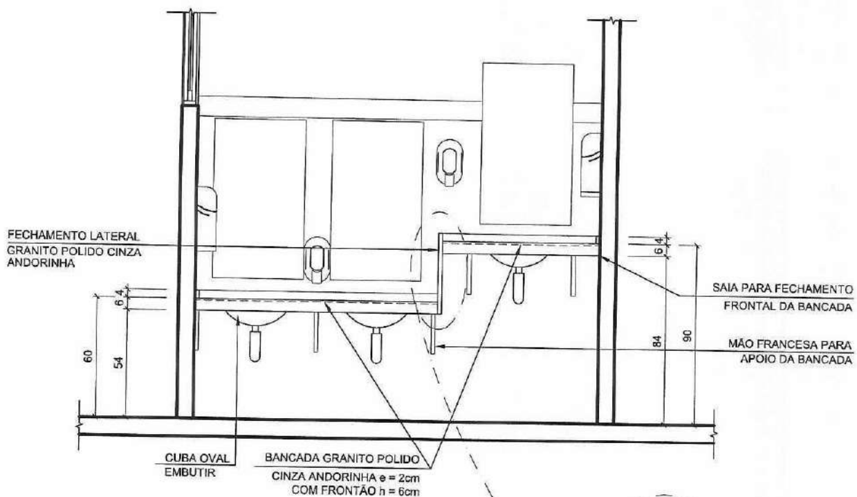
02 ELEVÇÃO ESCALA 1:25
