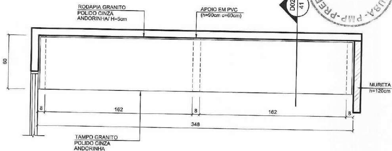
01 PLANTA ESCALA 1:25
