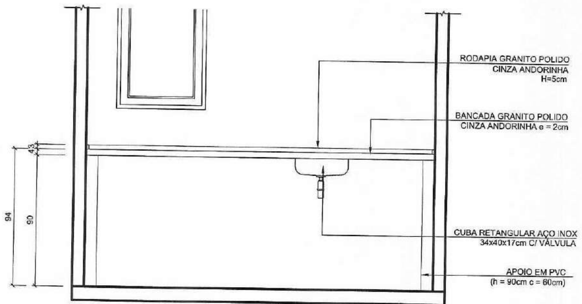
02 ELEVÇÃO ESCALA 1:25
