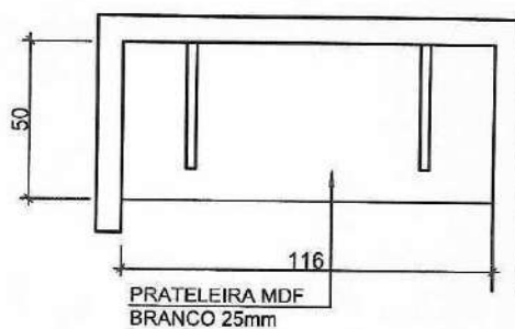
01 PLANTA ESCALA 1:25
