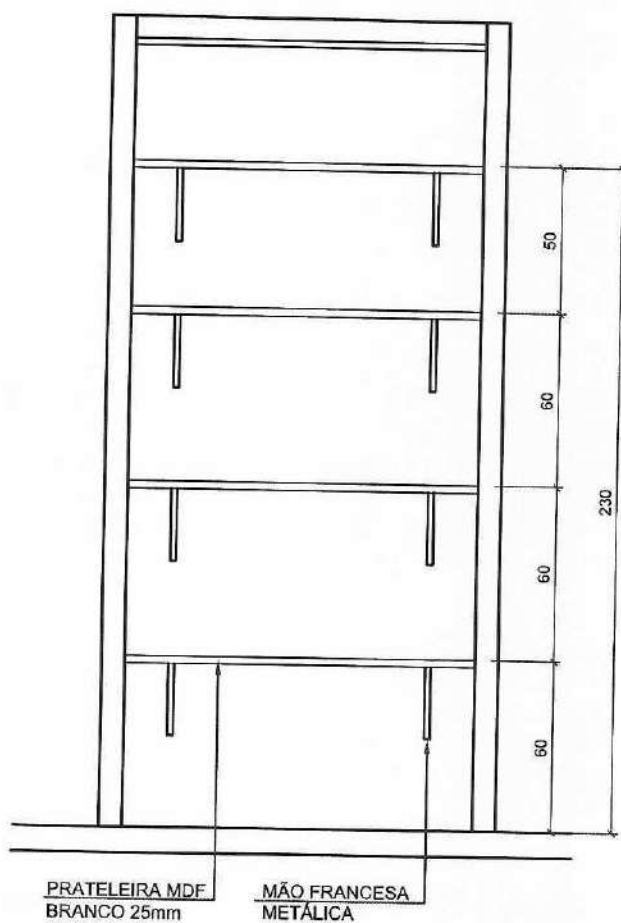
02 ELEVAÇÃO ESCALA 1:25
