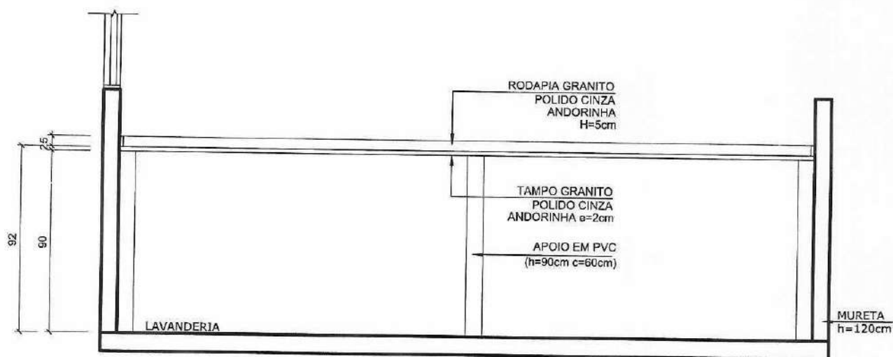
02 ELEVÇÃO ESCALA 1:25
