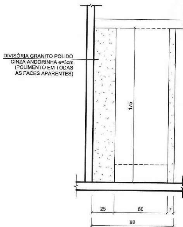
02 CORTE CC ESCALA 1:25
