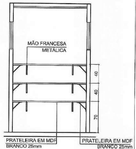
03 ELEVÇÃO B ESCALA 1:40
