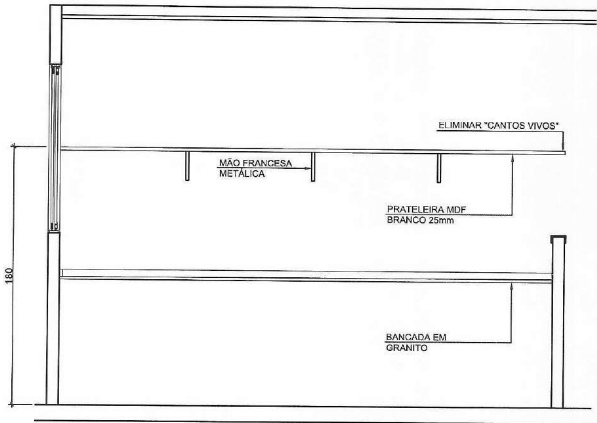
02 ELEVÇÃO ESCALA 1:25
