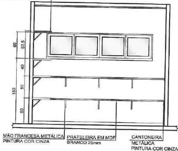
02 ELEVAÇÃO A ESCALA 1:50
