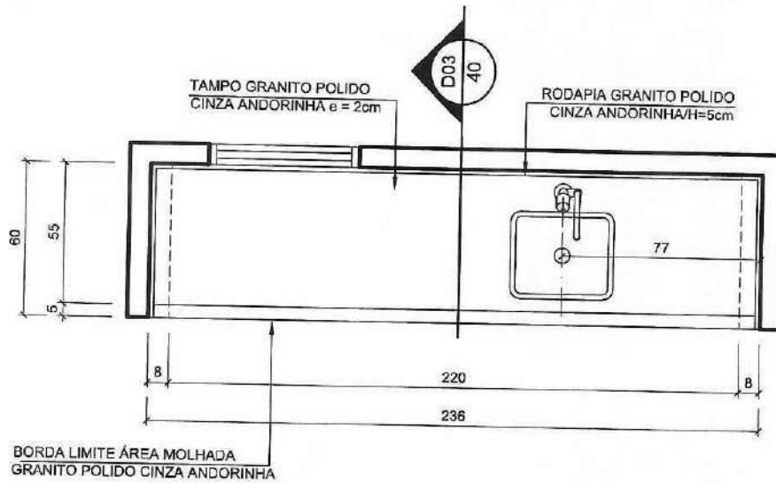
01 PLANTA ESCALA 1:25
