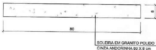
02 DETALHE SOLEIRA 2 ESCALA 1:10
