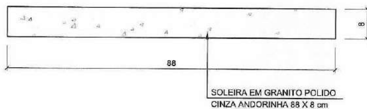
03 DETALHE SOLEIRA 3 ESCALA 1:10
