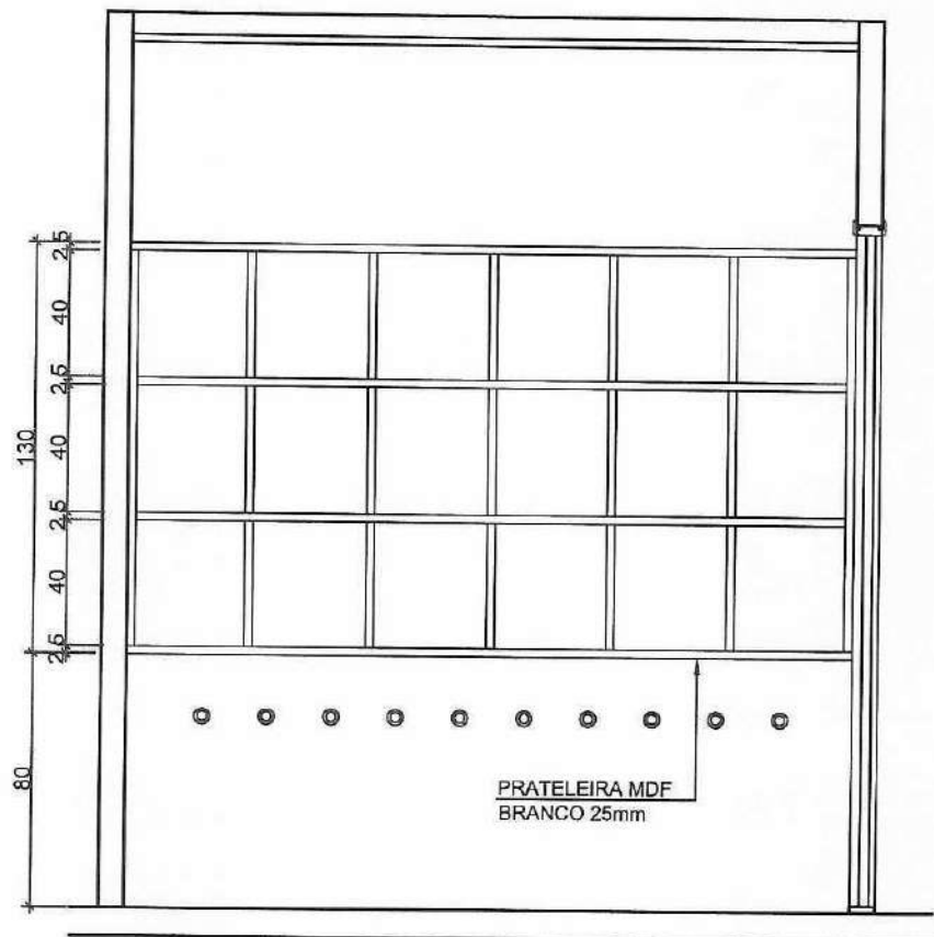
02 ELEVÇÃO ESCALA 1:25
