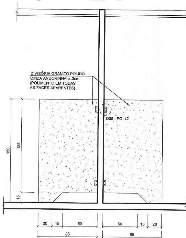
ELEVÇÃO ESCALA 1:25 02
