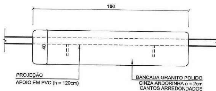
01 PLANTA ESCALA 1:25
