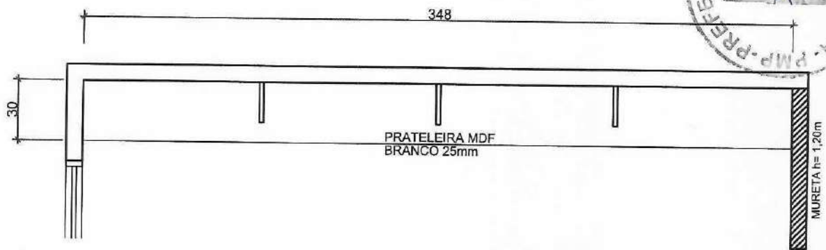
01 PLANTA ESCALA 1:25
