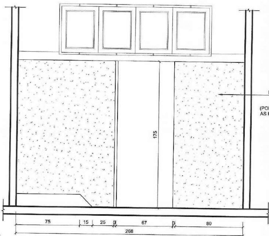
02 CORTE AA ESCALA 1:25
