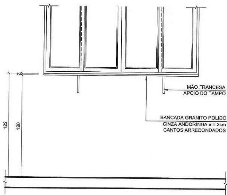
02 ELEVÇÃO ESCALA 1:25
