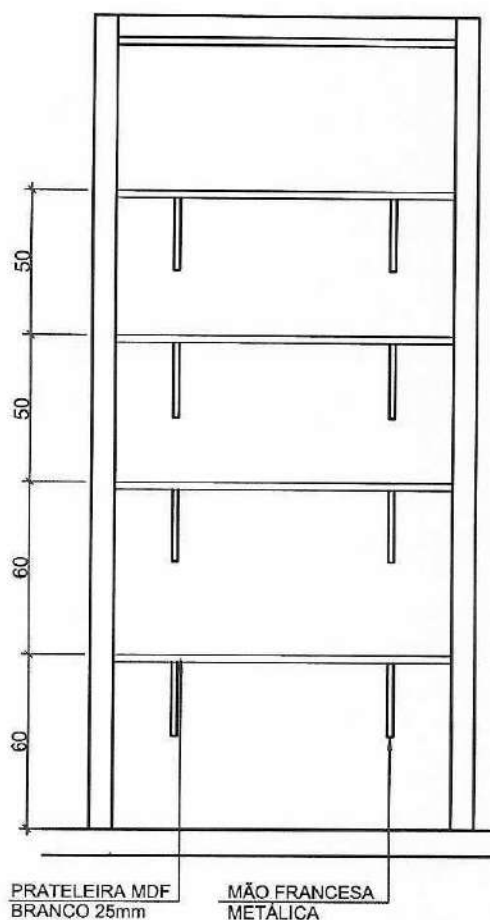
02 ELEVÇÃO ESCALA 1:25
