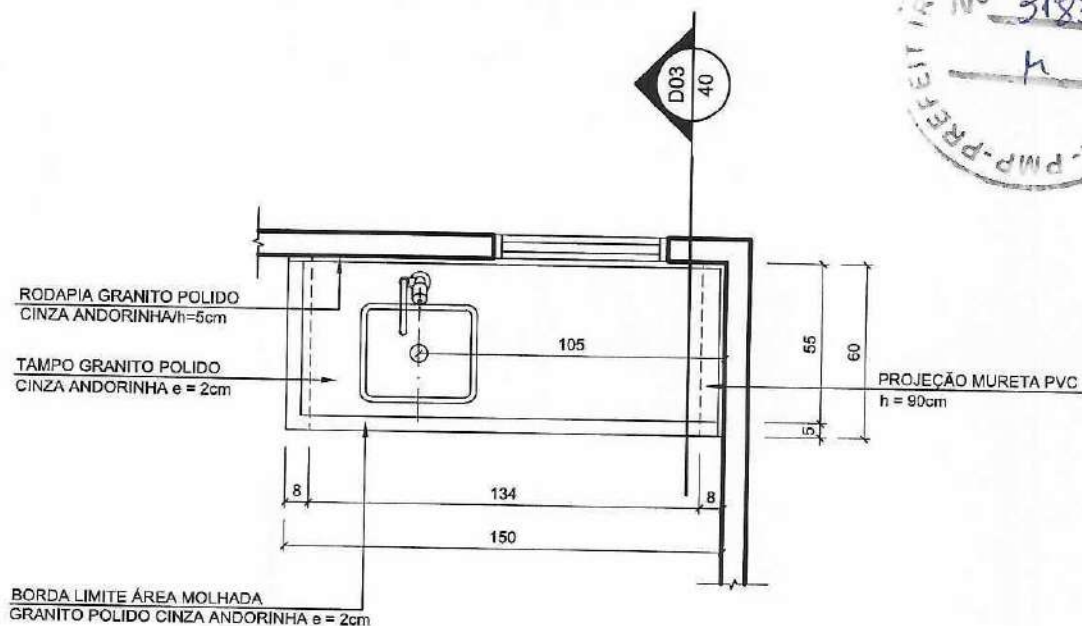
01 PLANTA ESCALA 1:25
