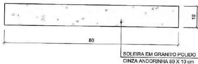
01 DETALHE SOLEIRA 1 ESCALA 1:10
