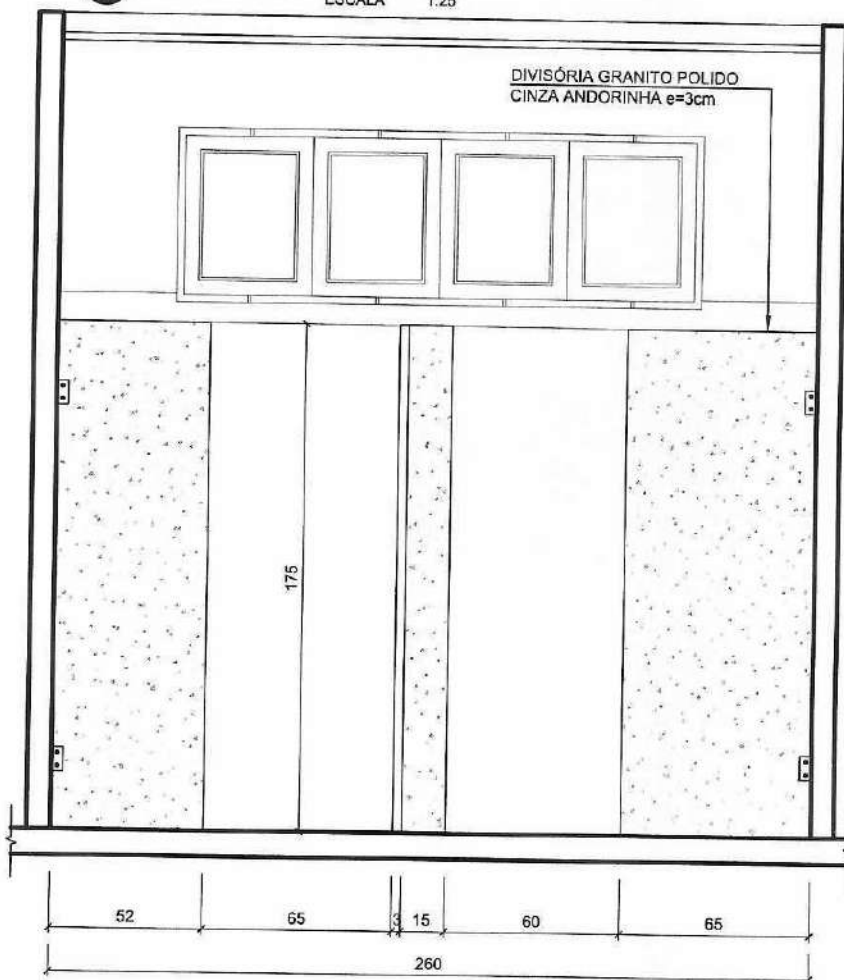
02 CORTE AA ESCALA 1:25
