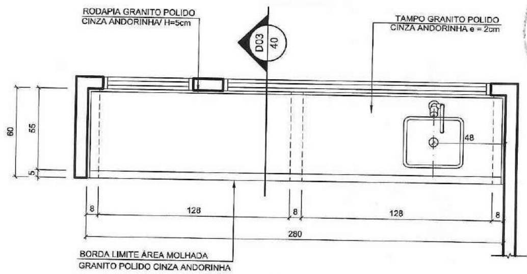
01 PLANTA ESCALA 1:25
