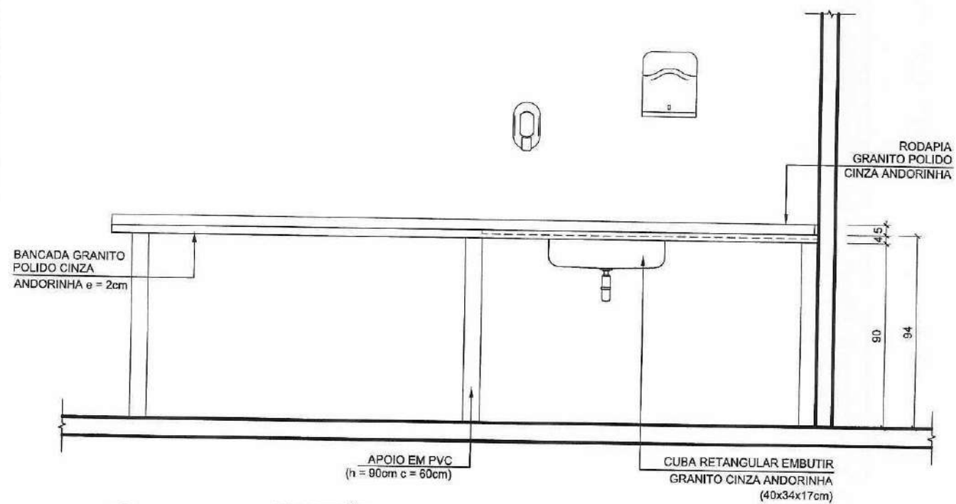
02 ELEVÇÃO ESCALA 1:25
