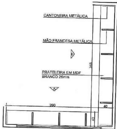
01 PLANTA ESCALA 1:50
