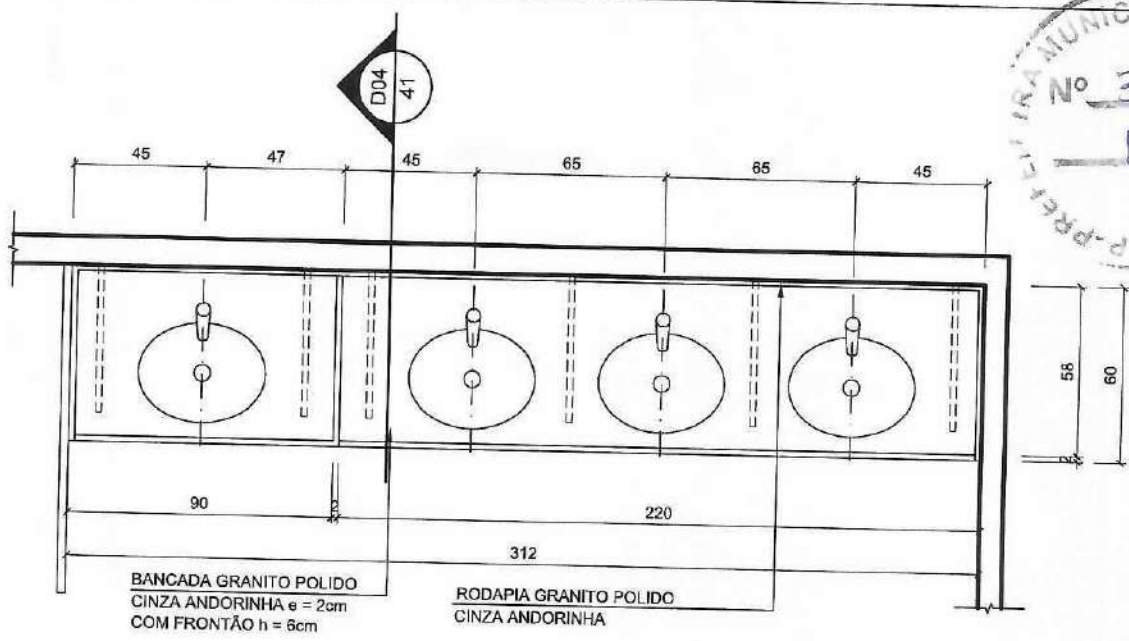
01 PLANTA ESCALA 1:25
