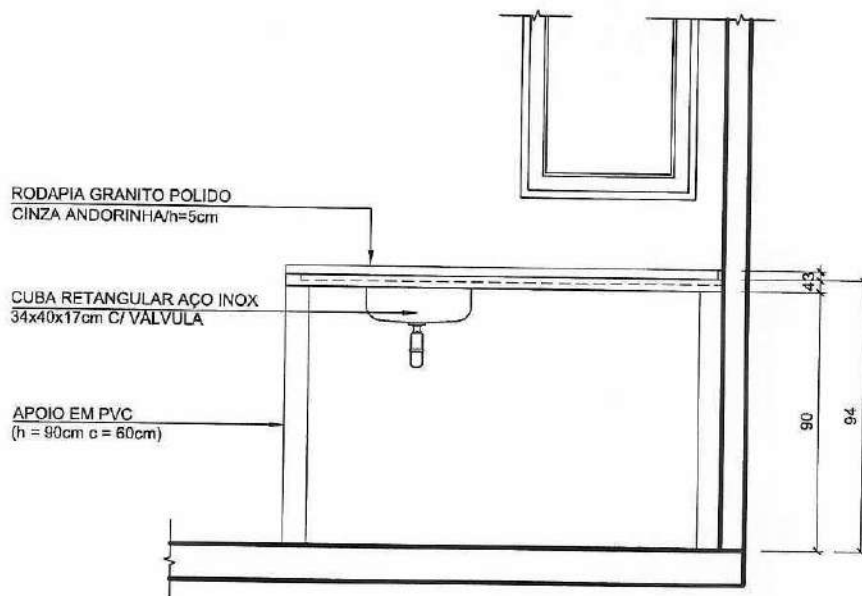
02 ELEVÇÃO ESCALA 1:25
