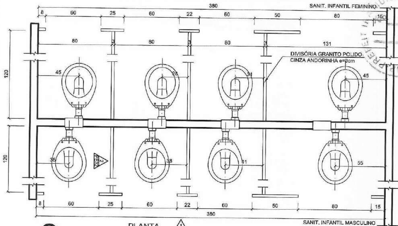
01 PLANTA ESCALA 1:25
