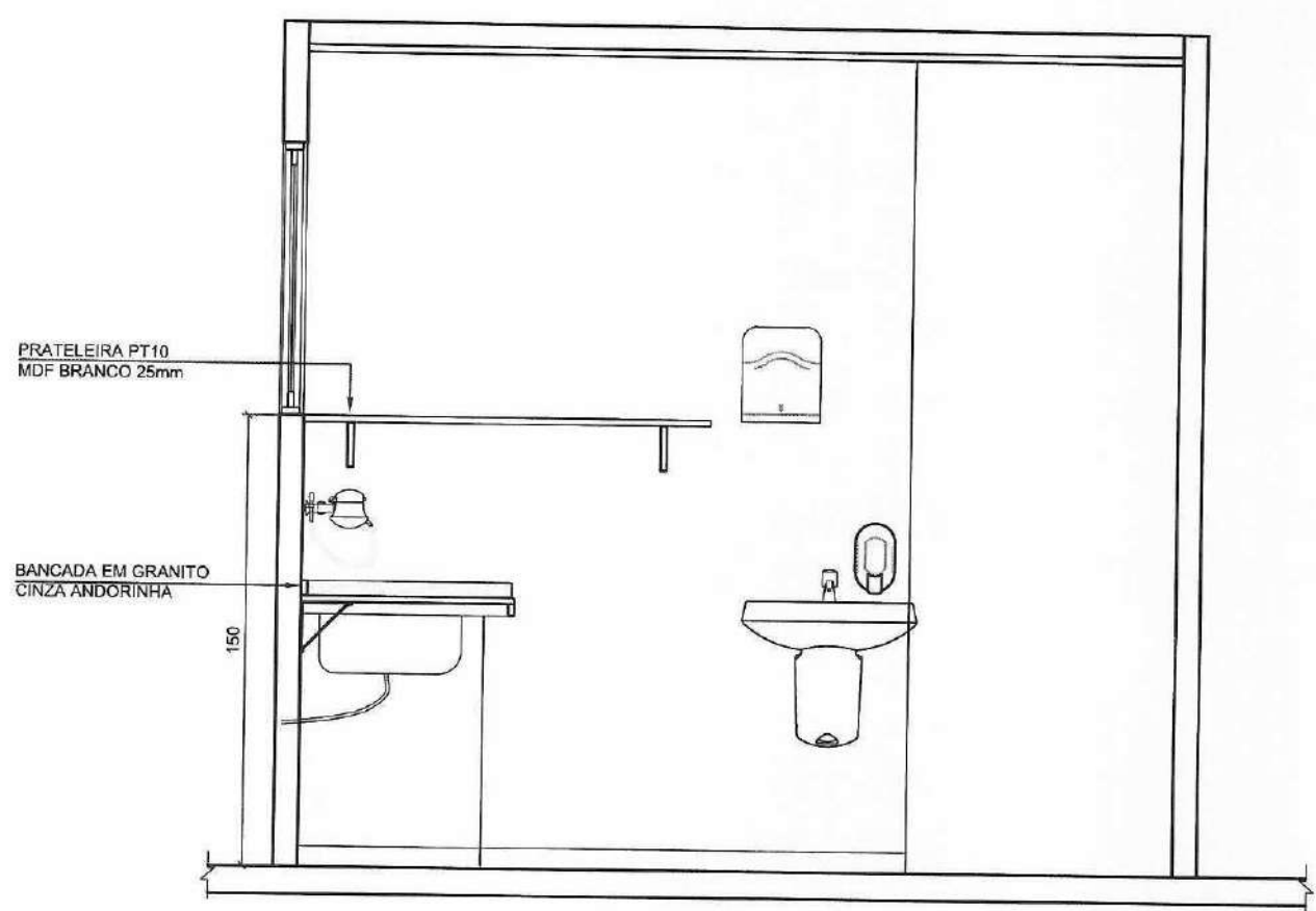
02 ELEVÇÃO ESCALA 1:25
