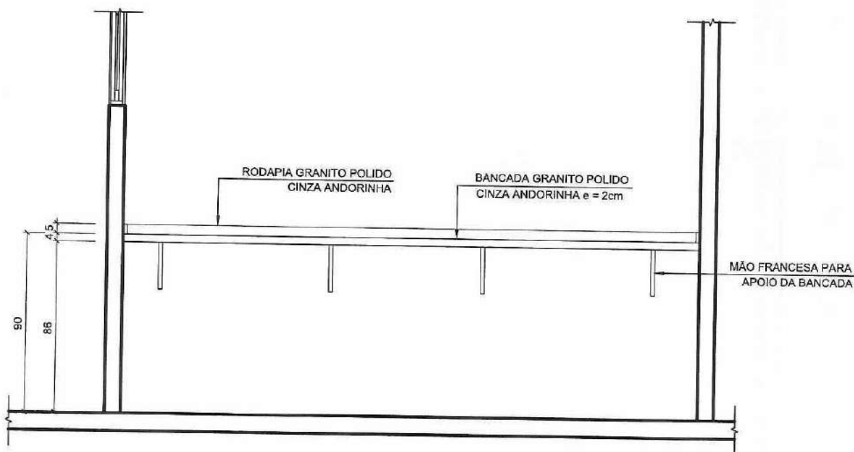
02 ELEVÇÃO ESCALA 1:25
