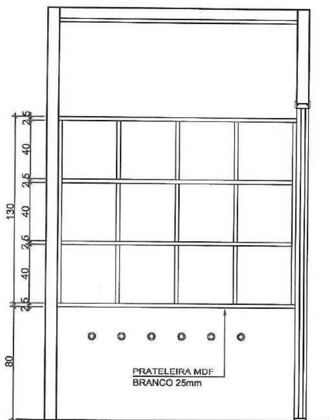
02 ELEVÇÃO ESCALA 1:25
