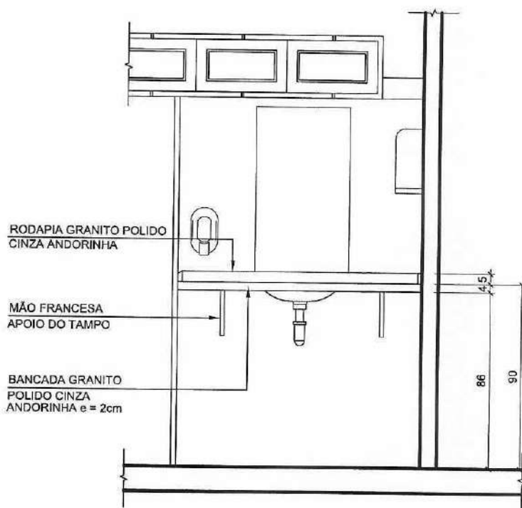
02 ELEVACÃO ESCALA 1:25
