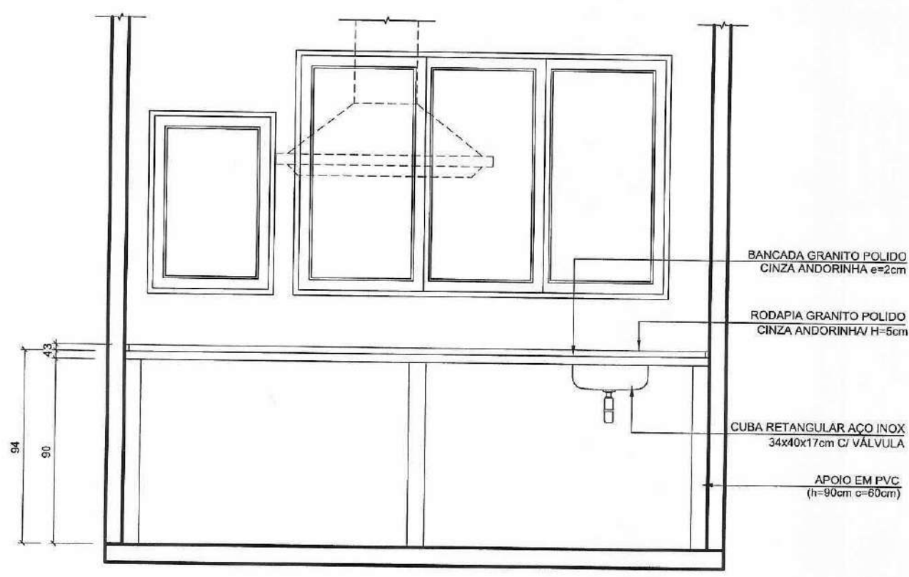
02 ELEVÇÃO ESCALA 1:25
