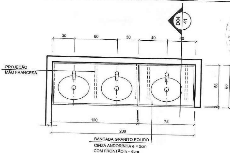
01 PLANTA ESCALA 1:25
