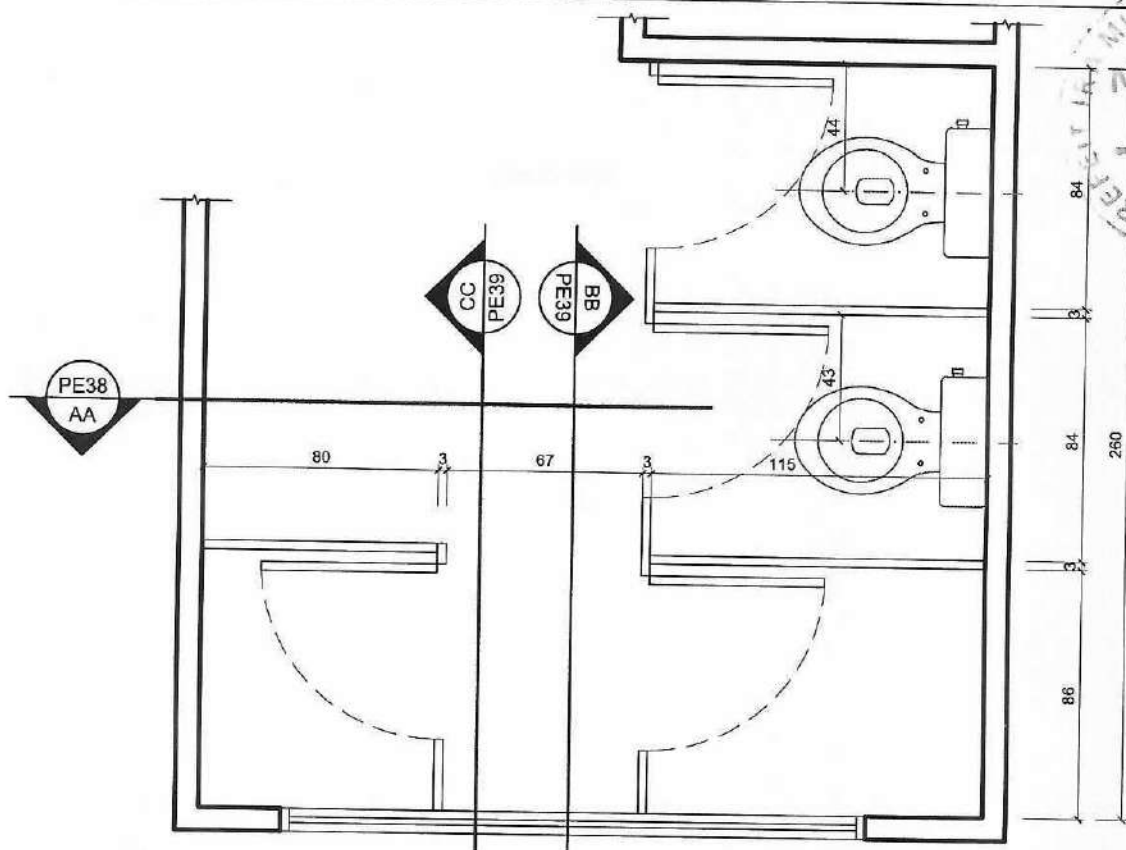
01 PLANTA ESCALA 1:25
