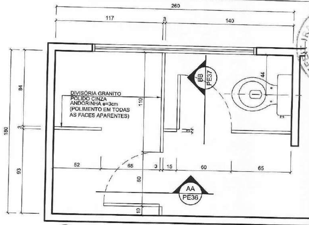
01 PLANTA ESCALA 1:25
