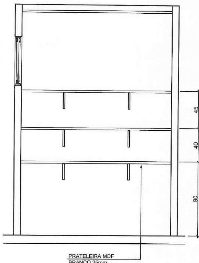
02 ELEVAÇÃO ESCALA 1:25
