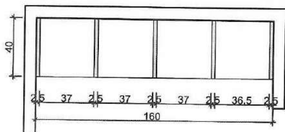
01 PLANTA ESCALA 1:25
