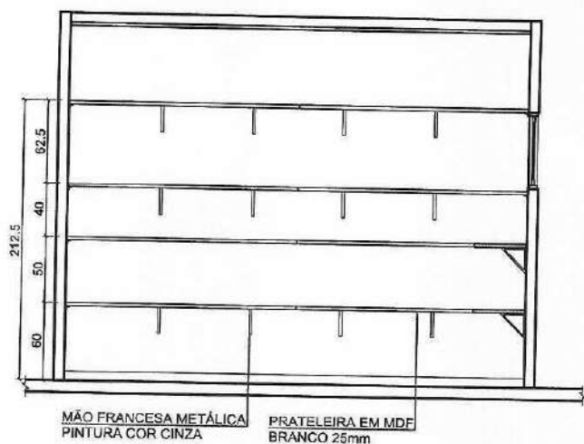
03 ELEVAÇÃO B ESCALA 1:50
