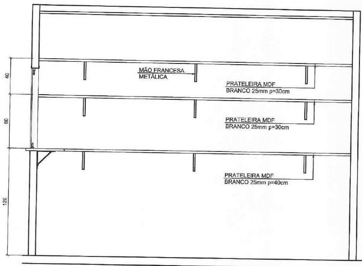
ELEVÇÃO
