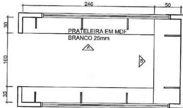
01 PLANTA ESCALA 1:40
