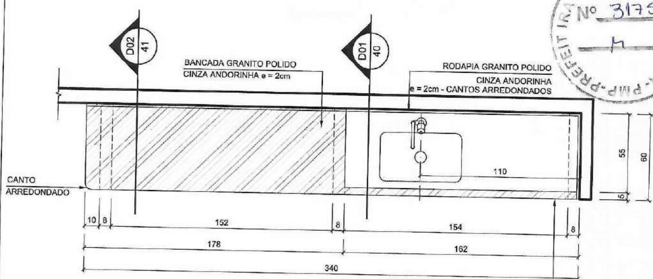
01 PLANTA ESCALA 1:25
