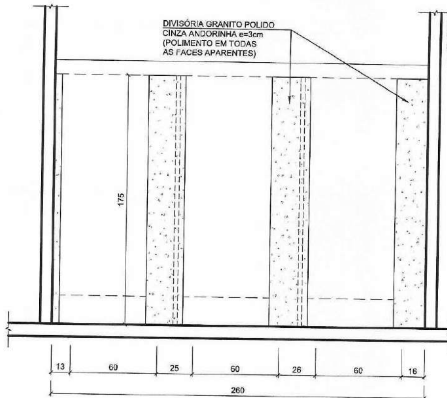
01 CORTE BB ESCALA 1:25
