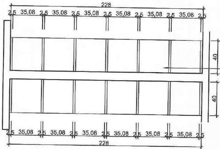
01 PLANTA ESCALA 1:25
