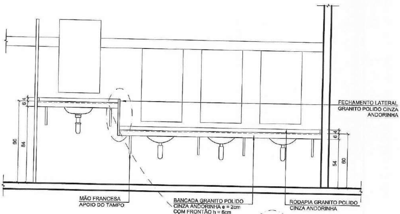
02 ELEVÇÃO ESCALA 1:25
