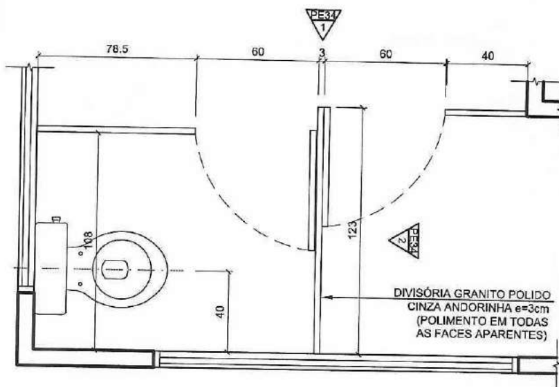
01 PLANTA ESCALA 1:25
