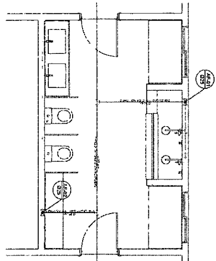
Planta 1
