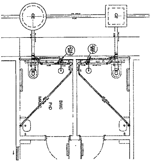
Detalhe S4 escala 1,25
