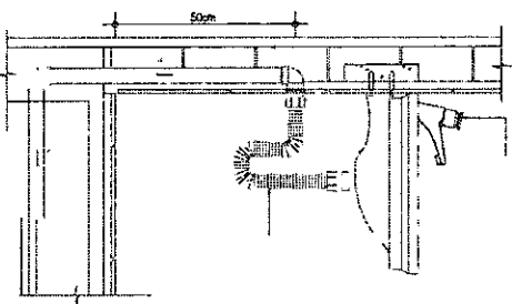
Detalhe de instalação
