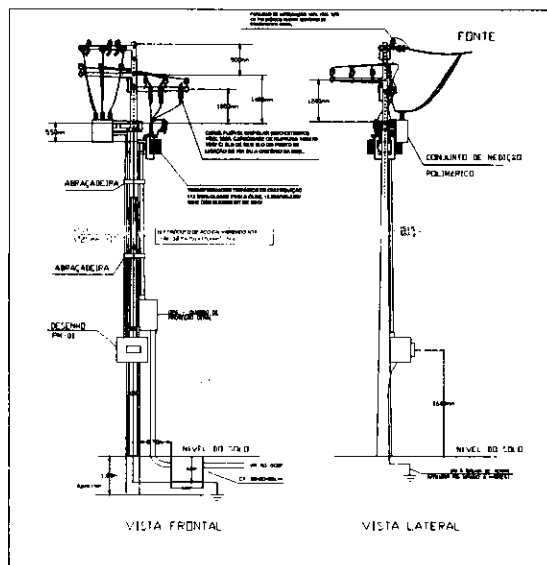
DETALHE 01 - CONJ. DE MEDIÇÃO E TRAFÓ DE 112,5 KVA ESCALA S/E
