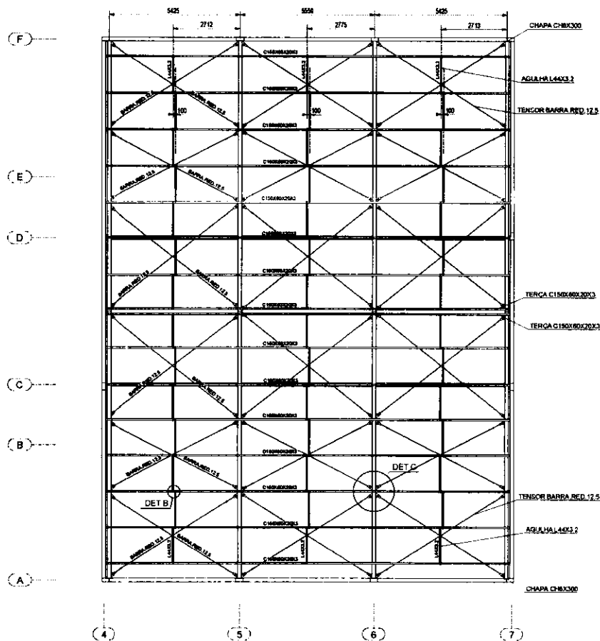
01 VISTA SUPERIOR DO BLOCO B ESCALA 1:50
