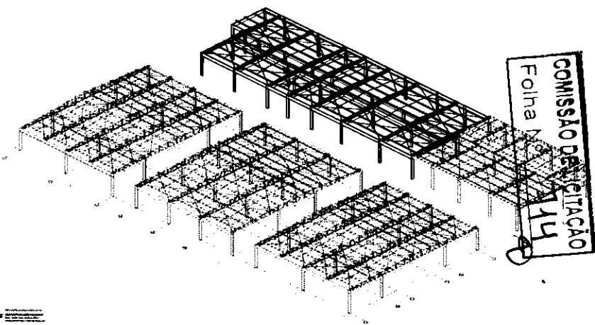
02 VISTA 3D DA COBERTURA METÁLICA ESCALA 1:30
