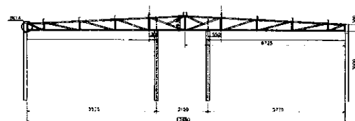
03 VISTA FRONTAL DO BLOCO E ESCALA 1:50
