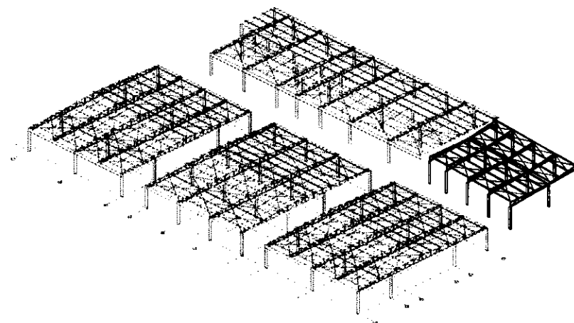
02 VISTA 3D DA COBERTURA METÁLICA ESCALA 1:50
