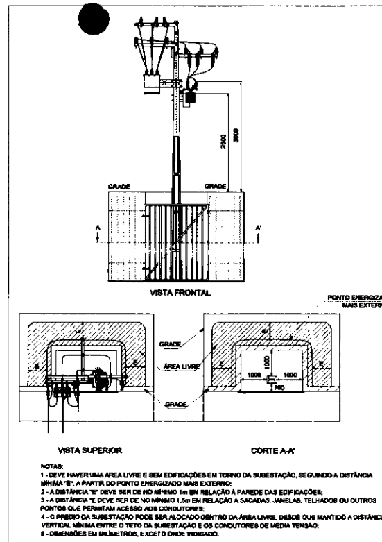
DETALHE 07 - RECUB. ESTRUTURA ÚNICA ESCALA S/E
