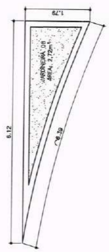
10.04 DETALHE - JARDINEIRA 08 ESCALA 1/50
