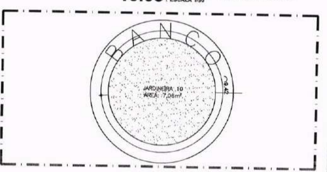
10.05 DETALHE - JARDINEIRA 10 ESCALA 1/50
