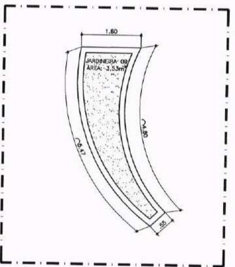
10.03 DETALHE - JARDINEIRAS 09 ESCALA 1/50
