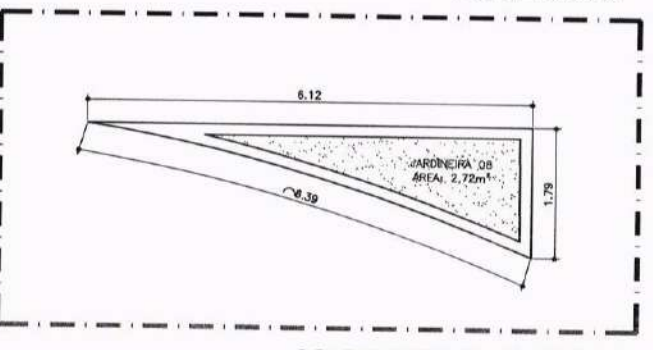
10.04 DETALHE - JARDINEIRA 08 ESCALA 1/50
