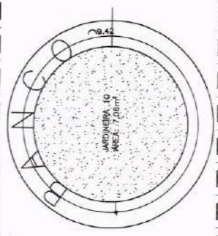
10.05 DETALHE - JARDINEIRA 10 ESCALA 1/50
