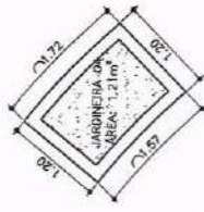
10.00 DETALHE - JARDINEIRAS 01 A 04 ESCALA 1/50
