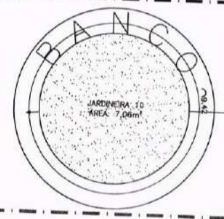
10.05 DETALHE - JARDINEIRA 10 ESCALA 1/50
