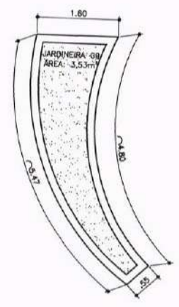
10.03 DETALHE - JARDINEIRAS 09 ESCALA 1/50
