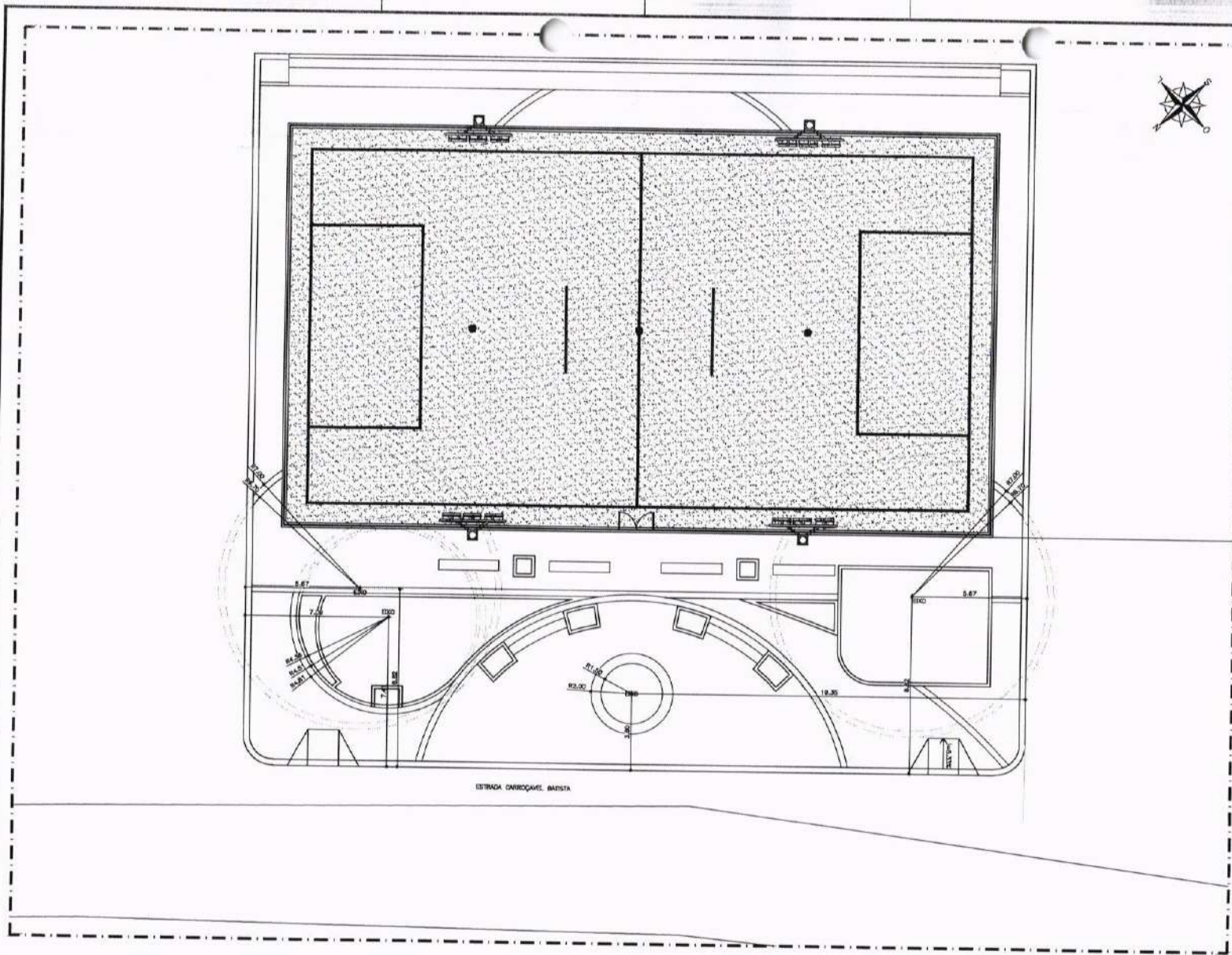
04.00 PLANTA BAIXA - IMPLANTAÇÃO 02 ESCALA 1:100
