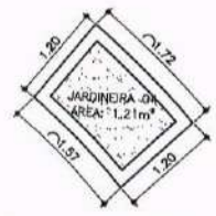
10.00 DETALHE - JARDINEIRAS 01 A 04 ESCALA 1/50
