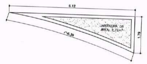
10.04 DETALHE - JARDINEIRA 08 ESCALA 1/50
