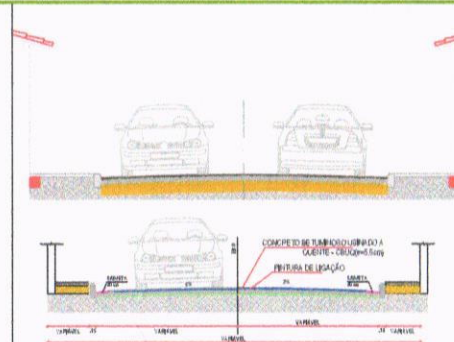
02 SEÇÃO TIPO ESCALA — 1 : 8/ESC
