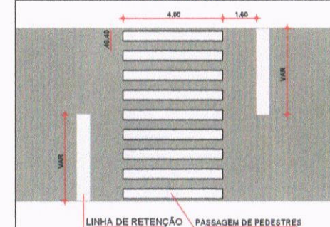
03 DET. FAIXA DE PEDESTRE ESCALA — 1 : 20
