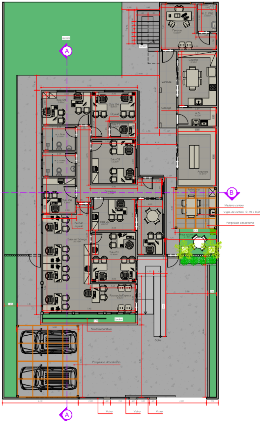
EXE Planta de layout - Pav. térreo ESC. 1:100
