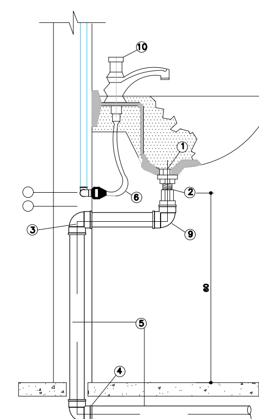
13 Detalhe - H5 Projeto Hidráulico - Terraço Escala: 1/25
