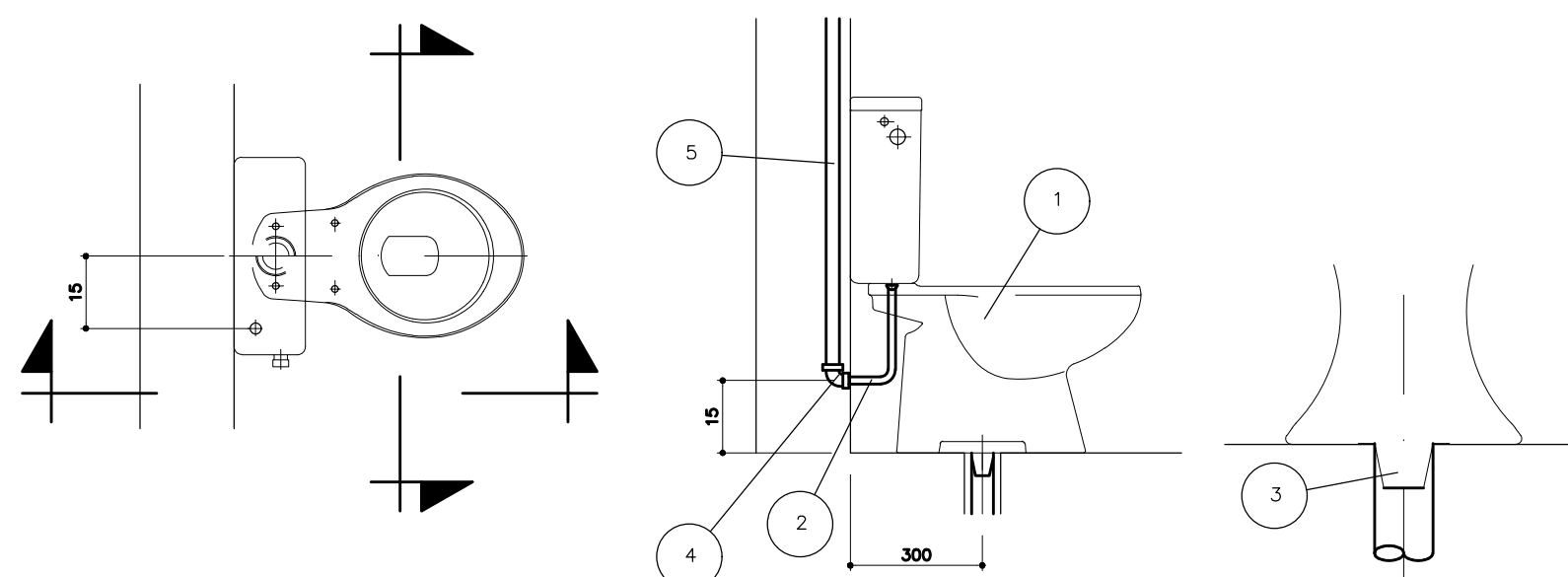
14 Vaso com caixa acoplada Projeto Hidráulico - Terraço Sem escala
