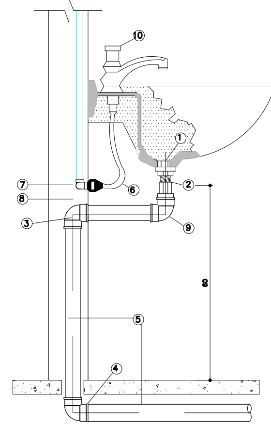
15 Detalhe Lavatório Projeto Hidráulico – Térreo Sem Escala
