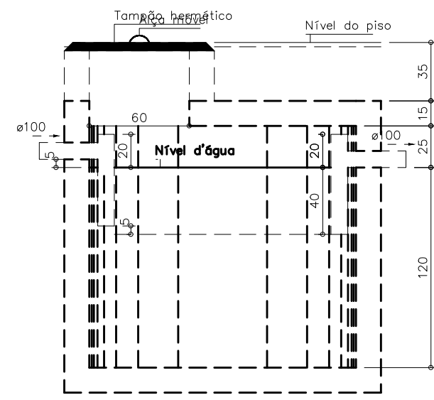
13 Tanque Séptico – Corte Projeto Sanitário – Térreo Escala: 1/25
