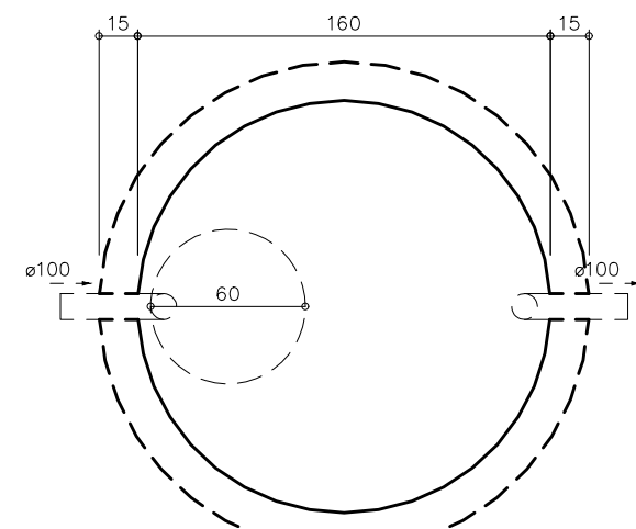
14 Tanque Séptico – Planta Baixa Projeto Sanitário – Térreo Escala: 1/25
