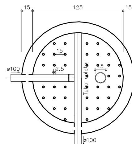
20 Filtro Anaeróbio – Corte 1 Projeto Sanitário – Térreo Escala: 1/25
