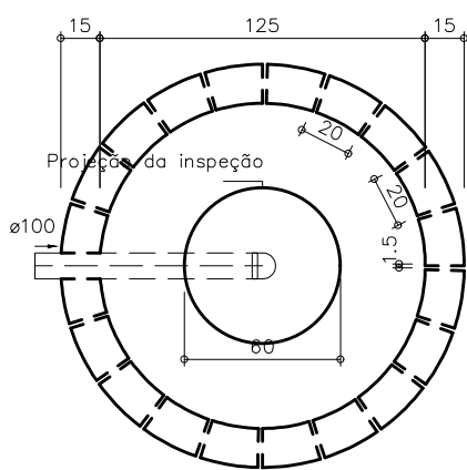
17 Sumidouro – Planta Baixa Projeto Sanitário – Térreo Escala: 1/25
