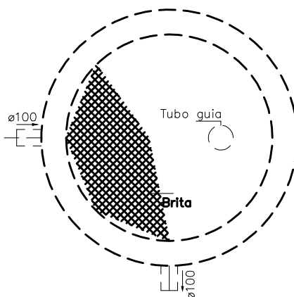
18 Filtro Anaeróbio – Planta Projeto Sanitário – Térreo Escala: 1/25
