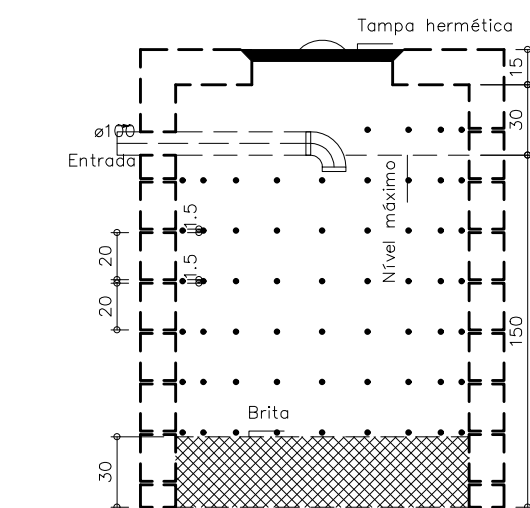
16 Sumidouro – Corte Projeto Sanitário – Térreo Escala: 1/25
