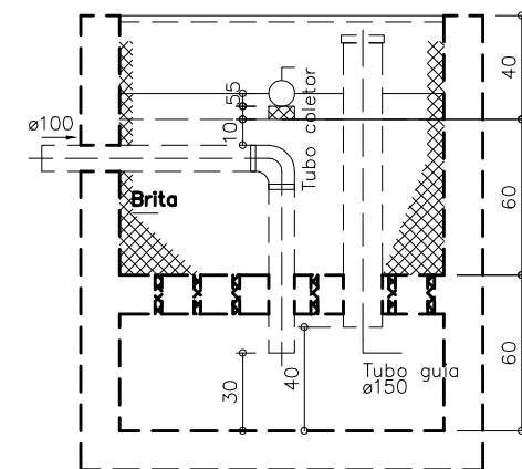
19 Filtro Anaeróbio – Corte 1 Projeto Sanitário – Térreo Escala: 1/25
