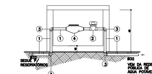
08 Hidrômetro Projeto Hidráulico - Térreo Sem Escala
