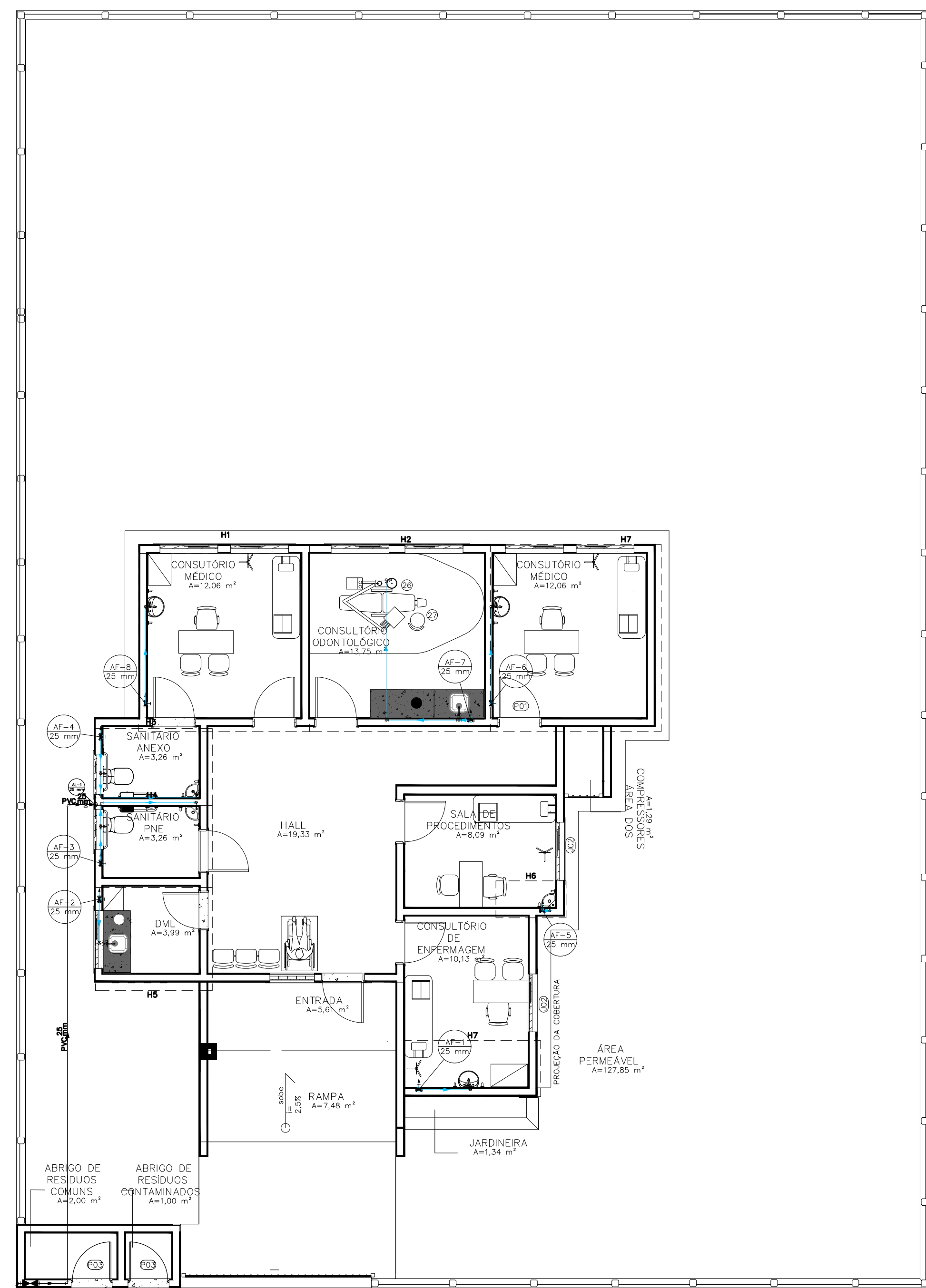
01 Planta Baixa - Térreo Projeto Hidráulico - Térreo Escala: 1/50
