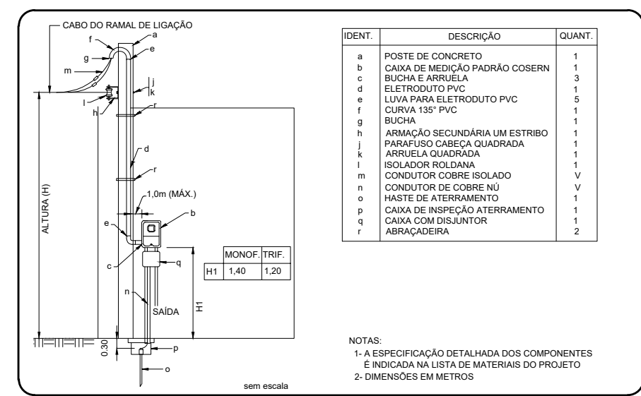
AÉREA COM ARMAÇÃO EM POSTE - MEDIÇÃO EM PAREDE - SAÍDA EMBUTIDA
