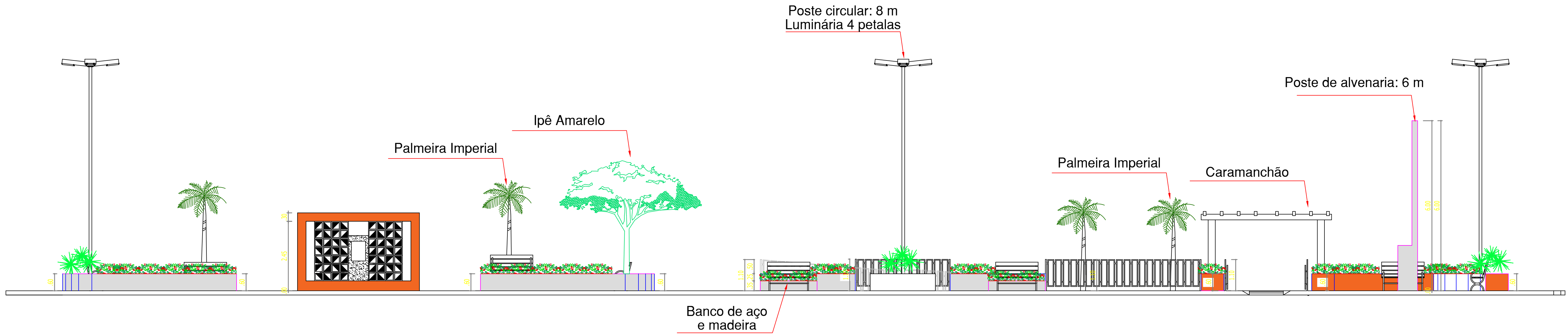
VISTA 02 Escala: 1/75
