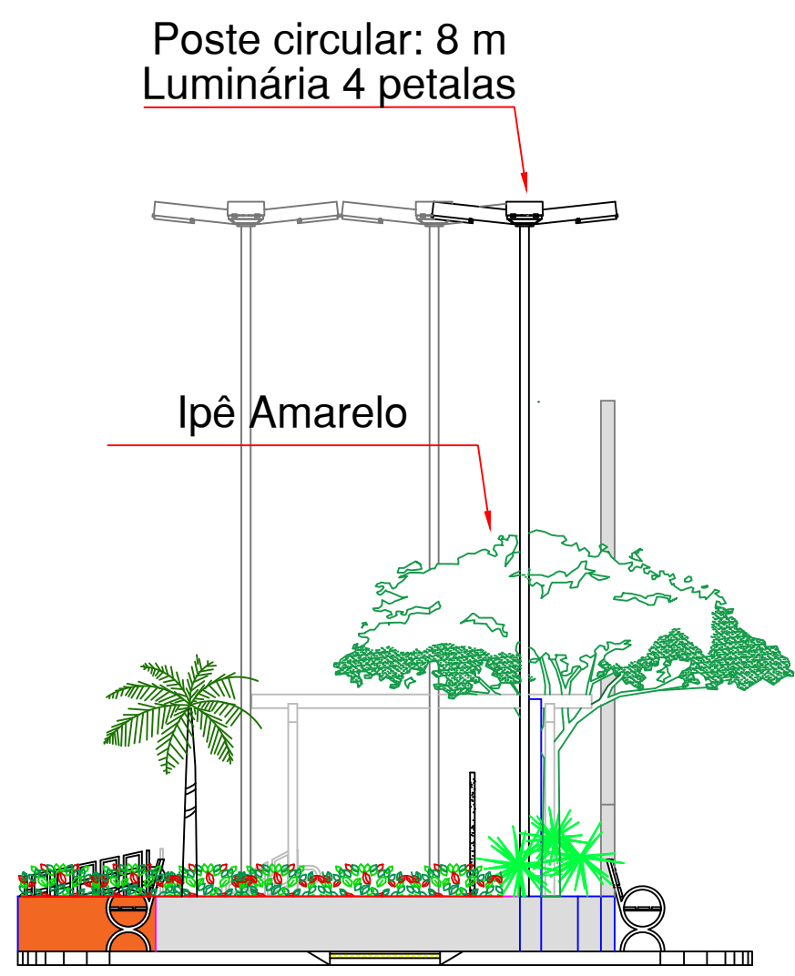
VISTA LATERAL 01 Escala: 1/75
