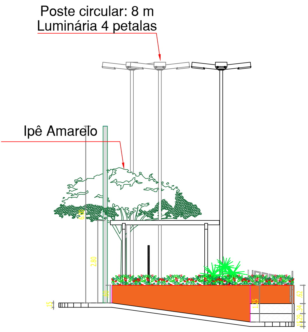
VISTA LATERAL 02 Escala: 1/75
