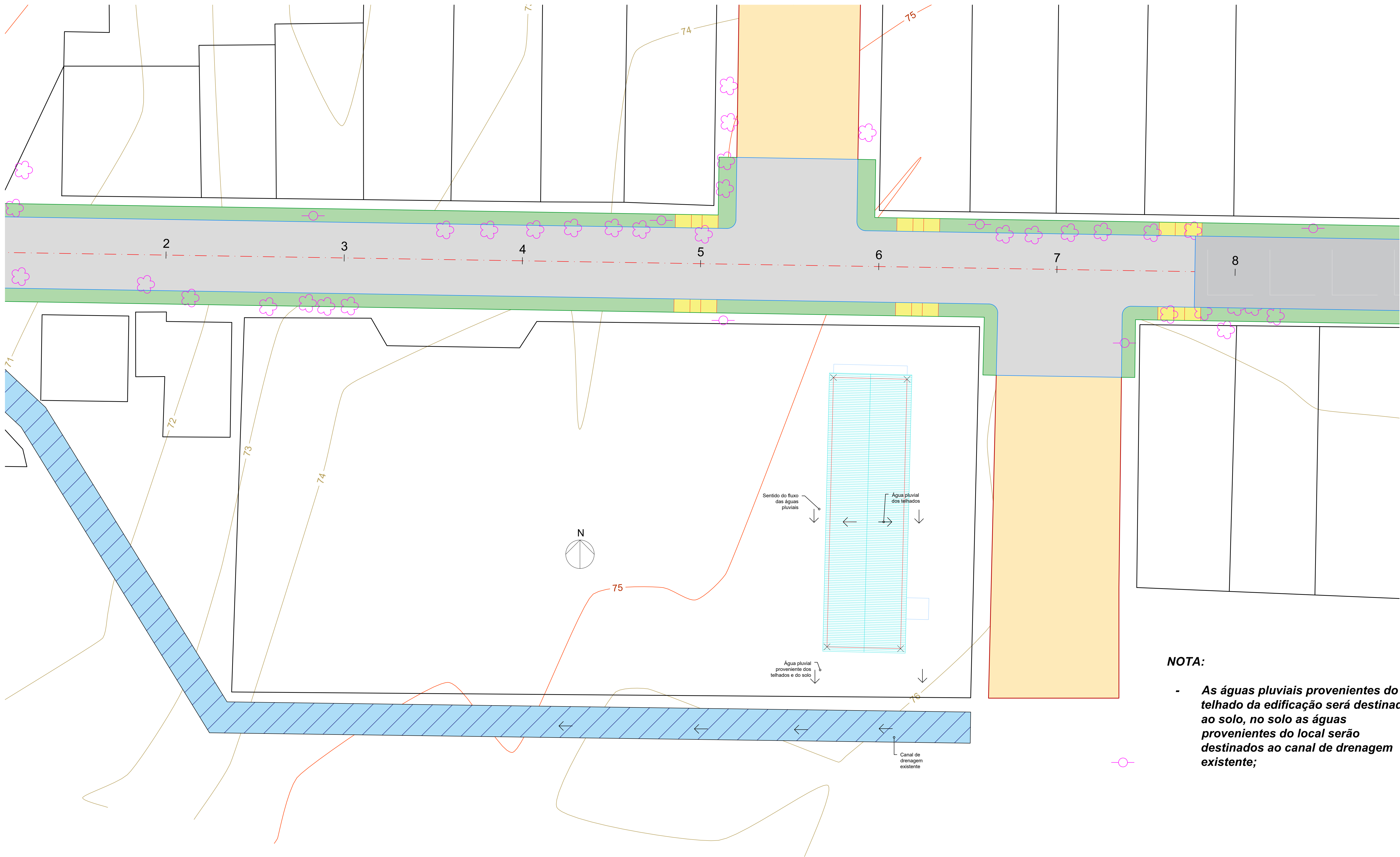
1 Planta de águas pluviais Esc.: 1:200
