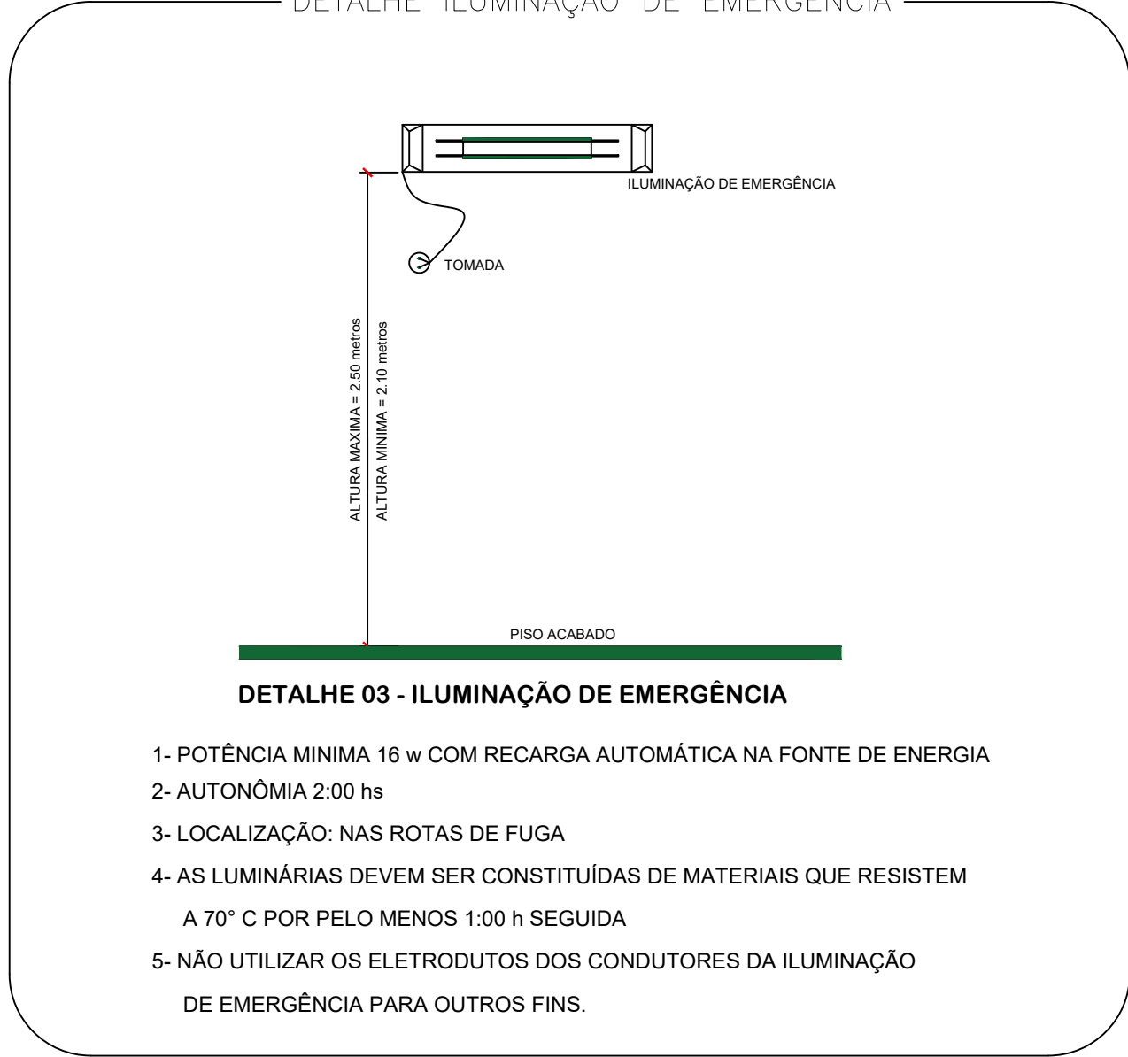
DETALHE ILUMINAÇÃO DE EMERGÊNCIA
