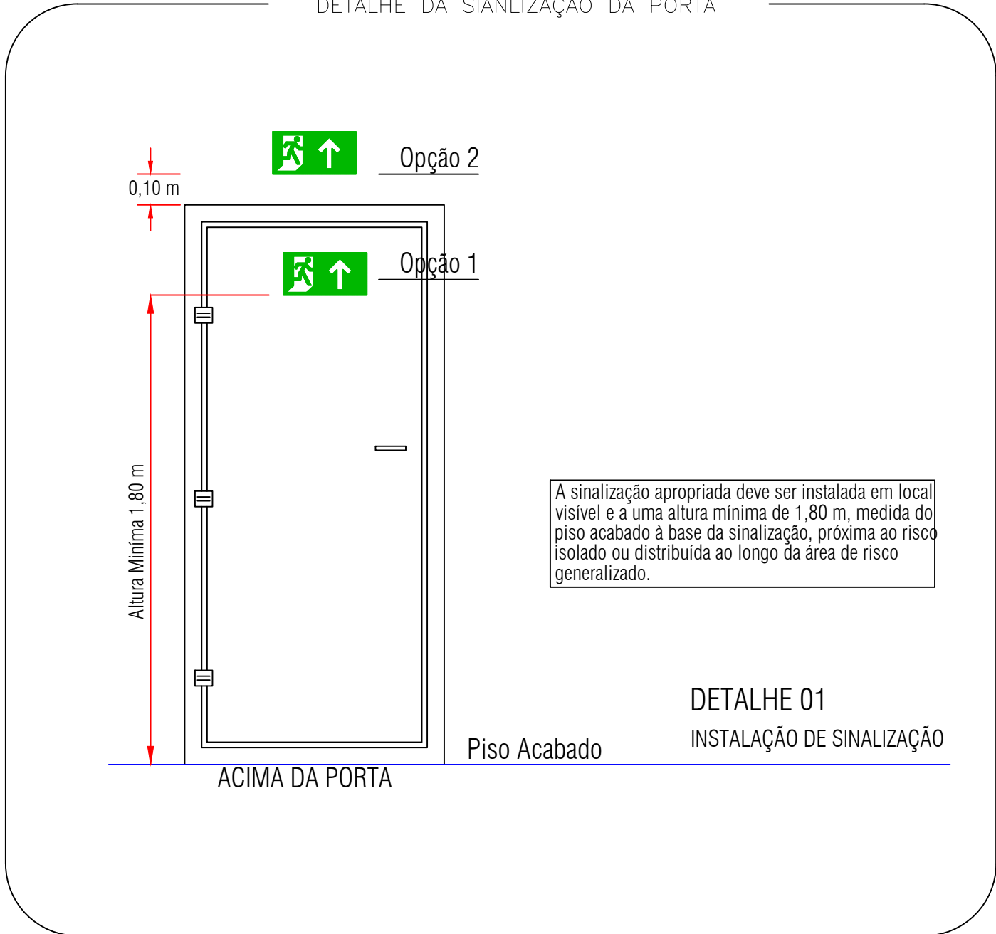
DETALHE DA SIANLIZAÇÃO DA PORTA
