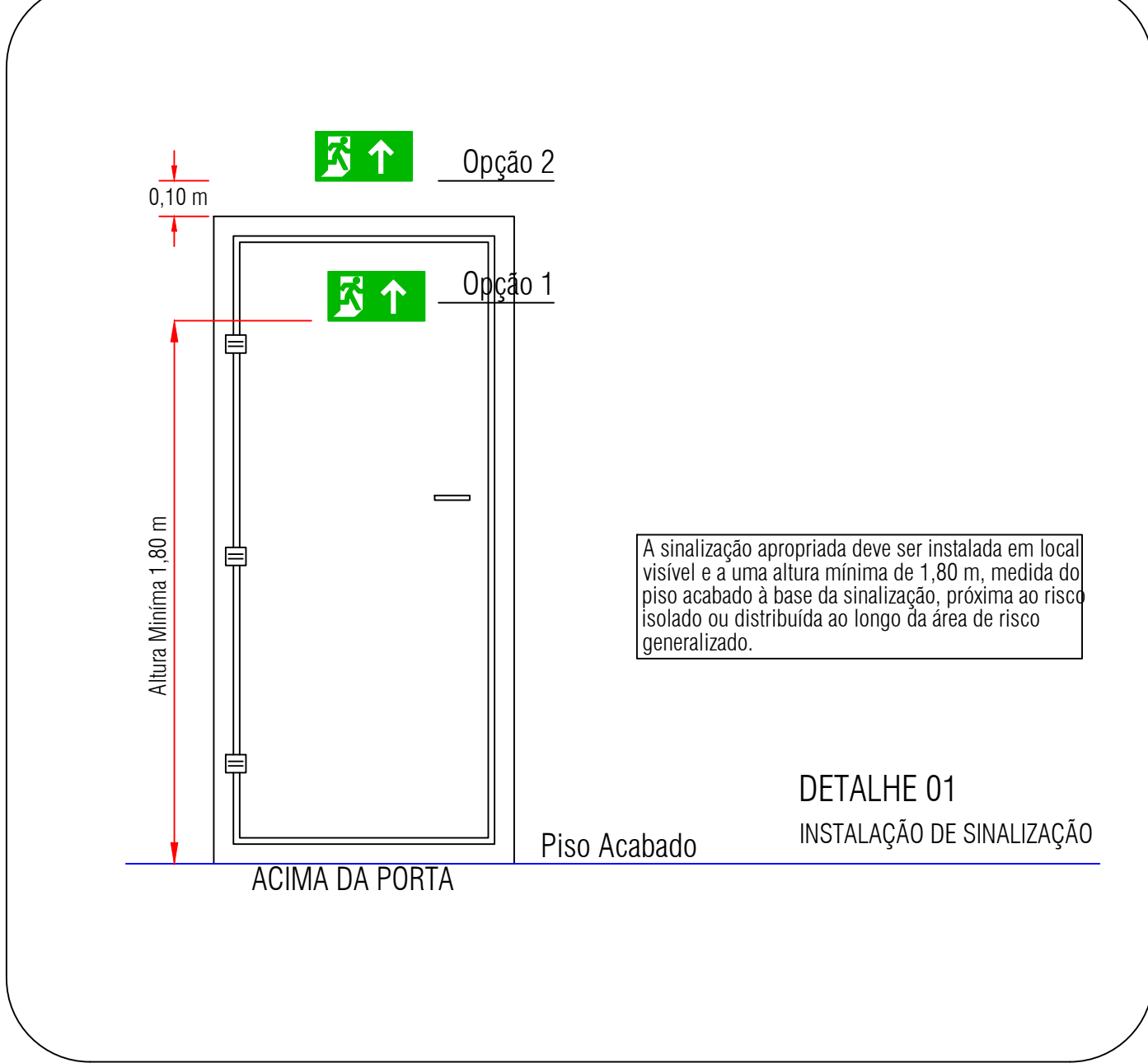
DETALHE DA SIANLIZAÇÃO DA PORTA
