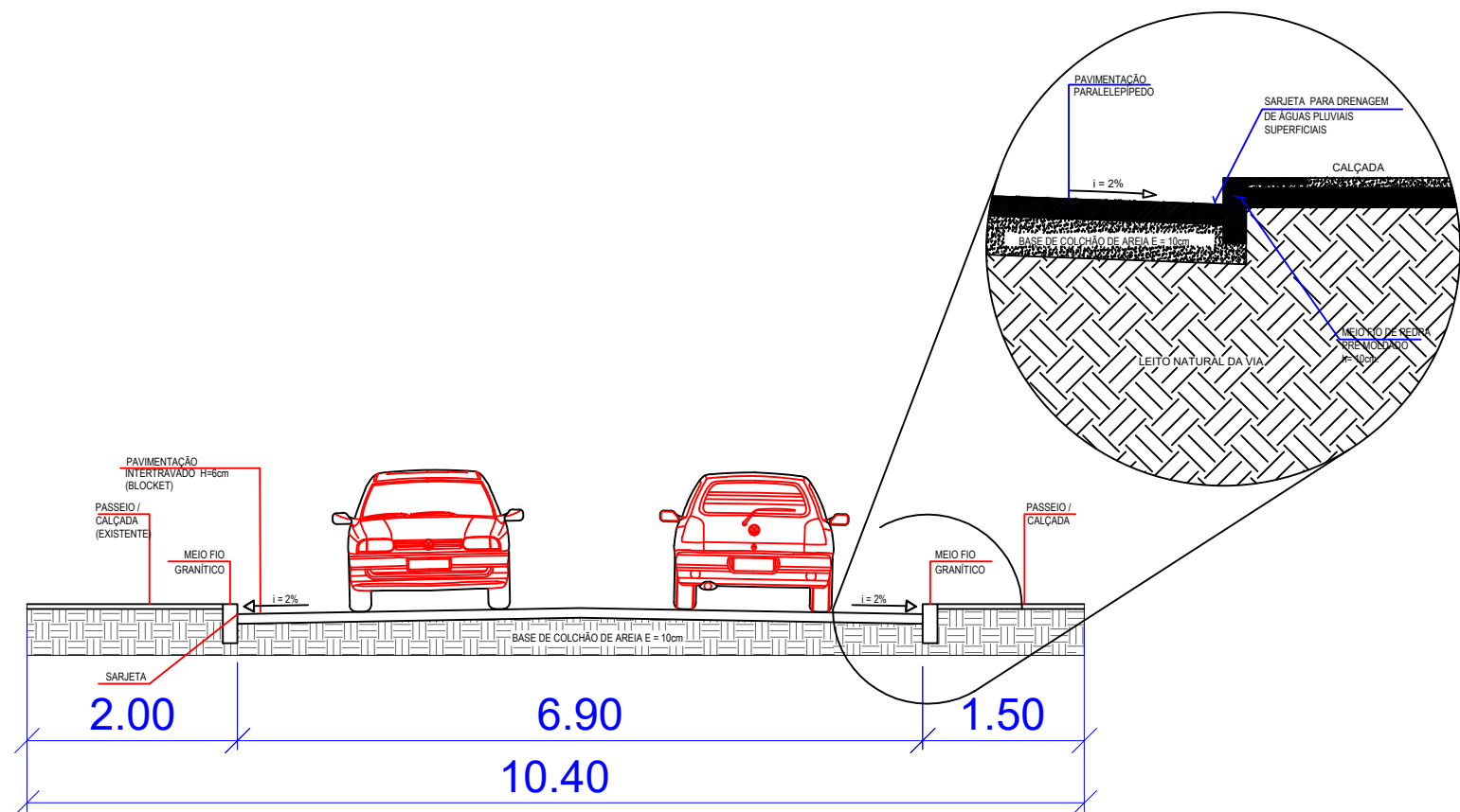
SECÇÃO TRANSVERSAL Escala 1/50
