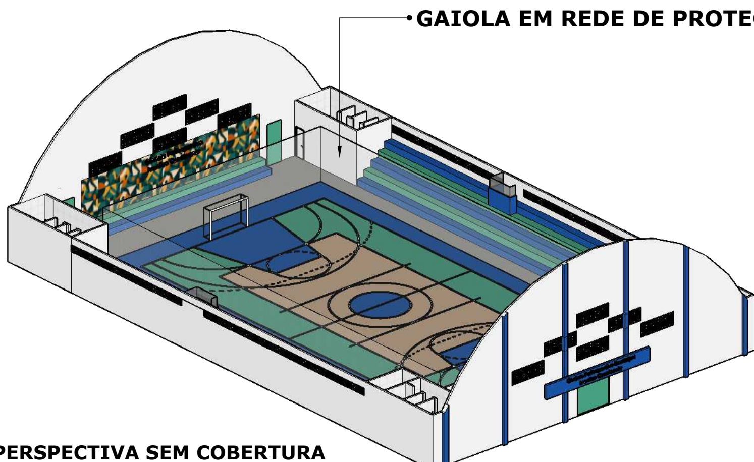
PERSPECTIVA SEM COBERTURA ESC.:1/75
