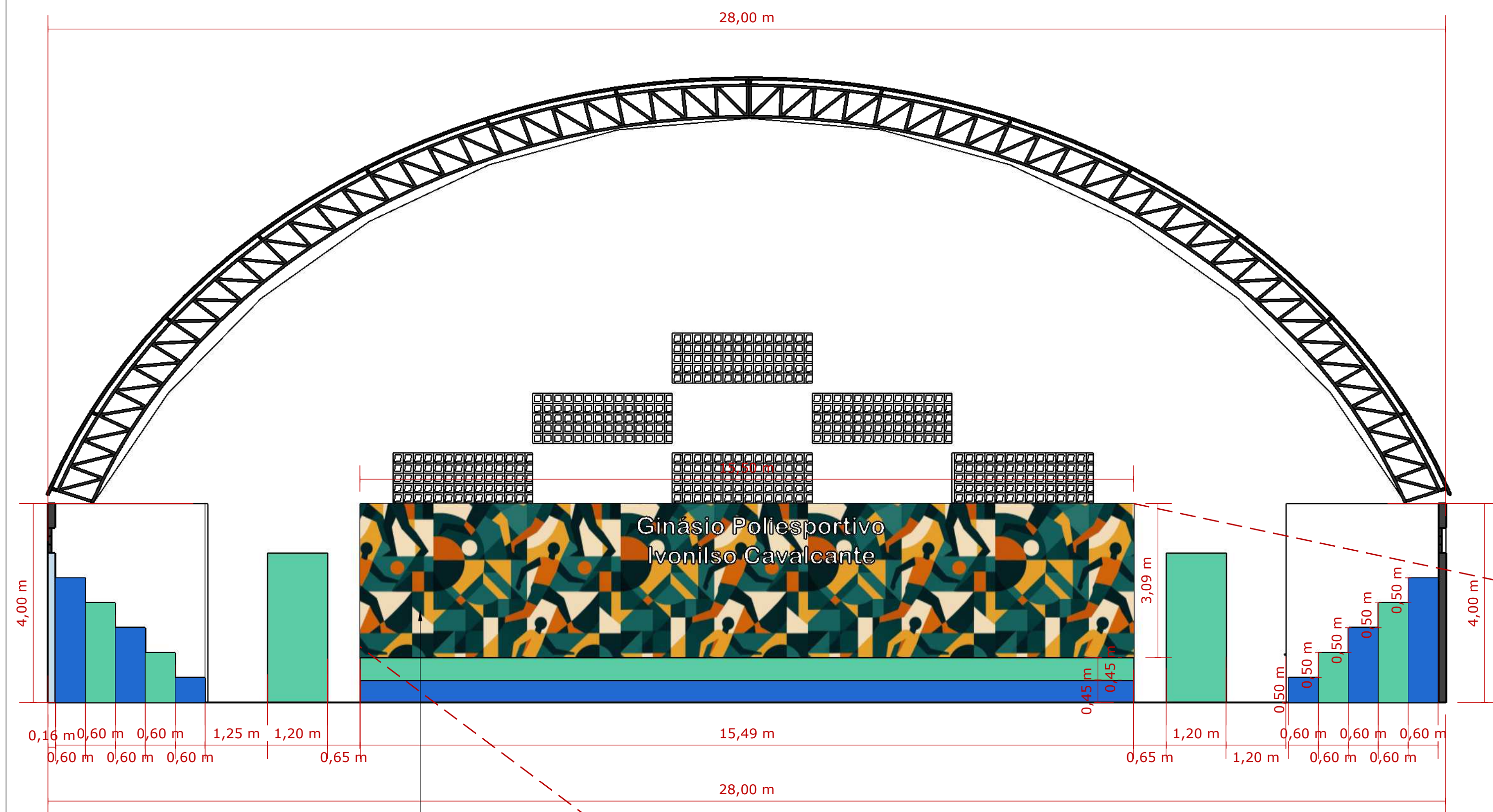
CORTE 03 ESC.:1/75
