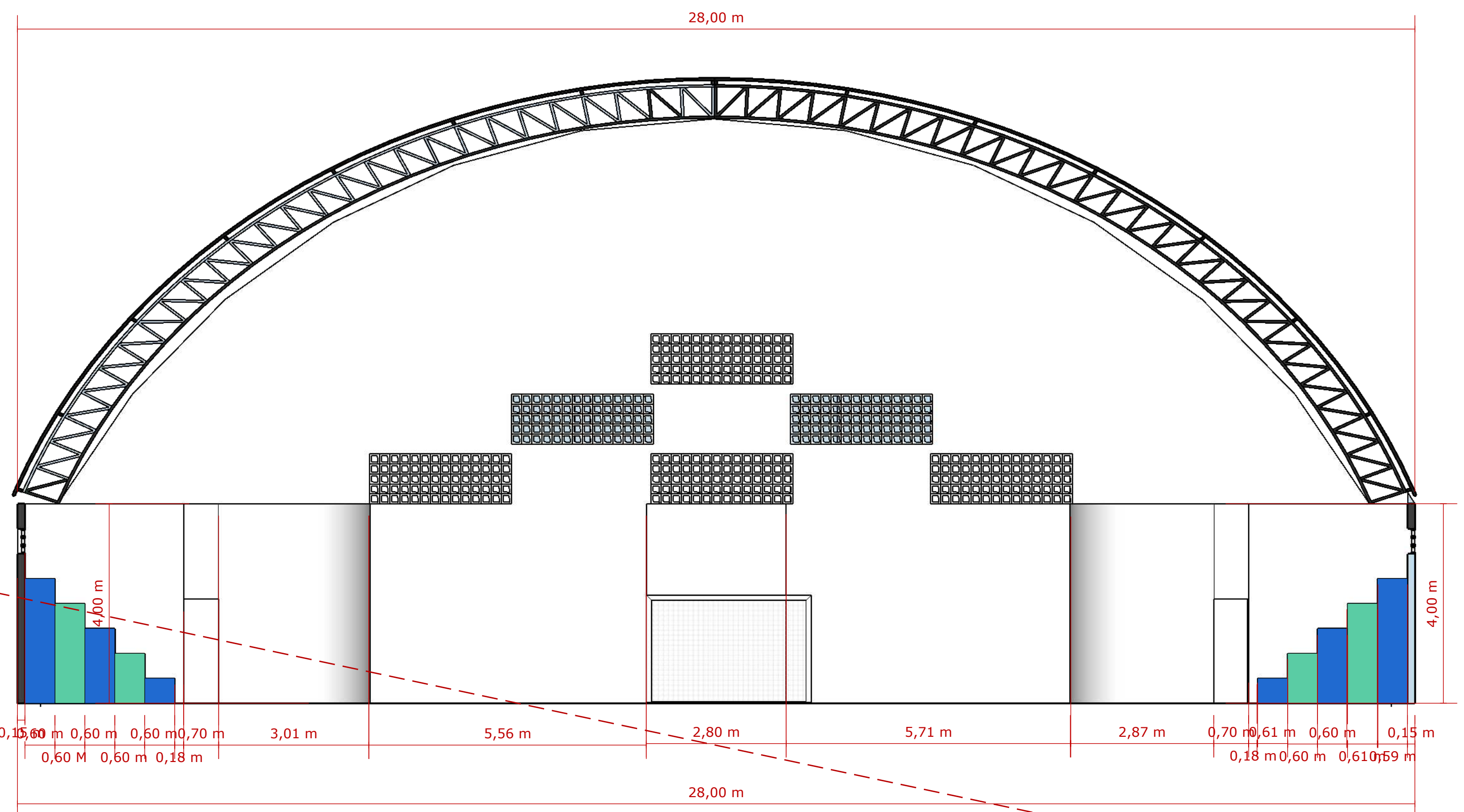
CORTE 04 ESC.:1/75
