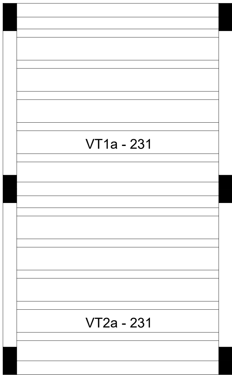
Planta de vigotas pré-moldadas escala 1:50
