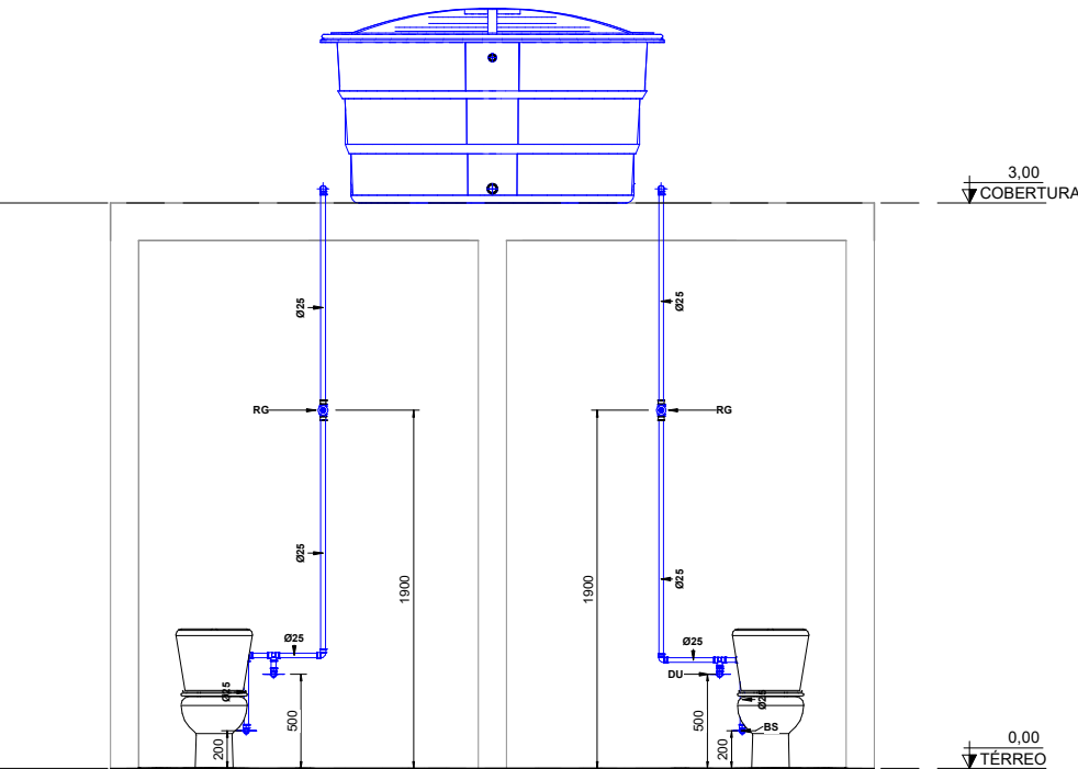
CORTE A-A
