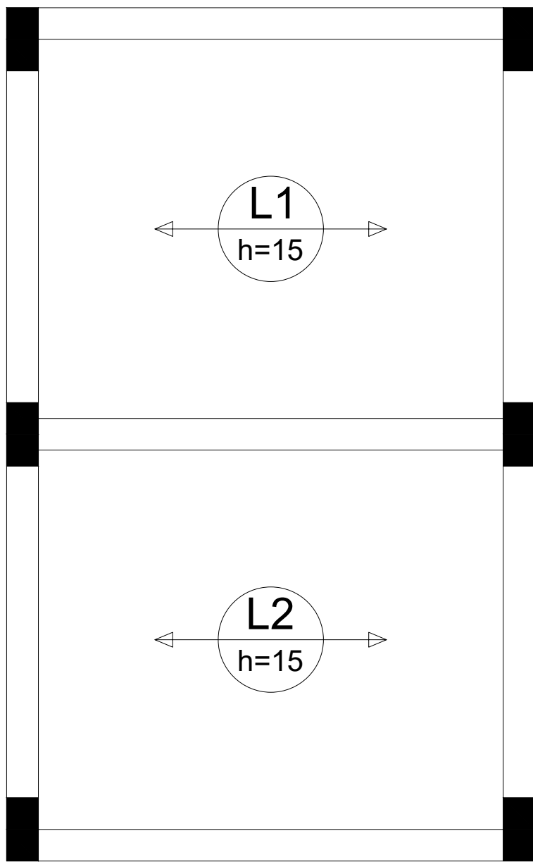
Armação positiva das lajes do pavimento reservatorio (Eixo X) escala 1:50
