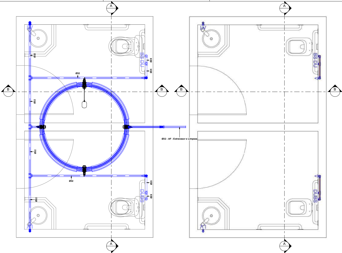
PLANTA DO TÉRREO
