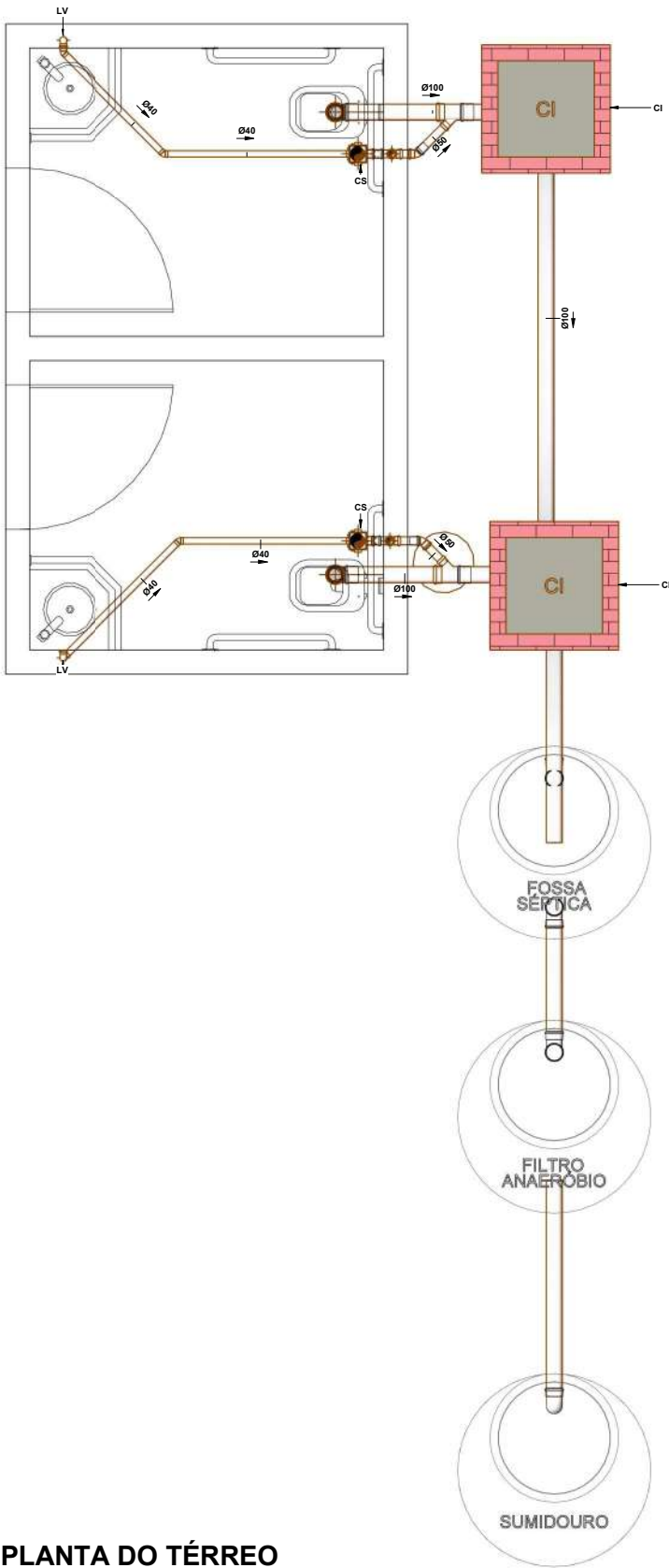
PLANTA DO TÉRREO 1 : 20
