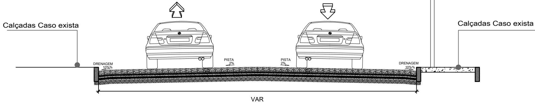
CORTE TRANSVERSAL - RUA LUIZ BATISTA SEM ESCALA
