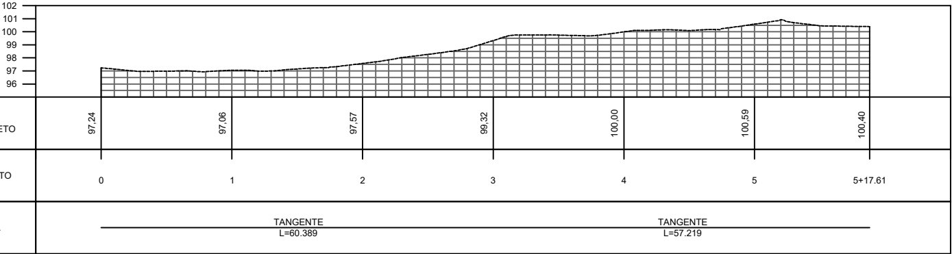
PERFIL RUA KERGINALDO FERREIRA - PARTE 1
