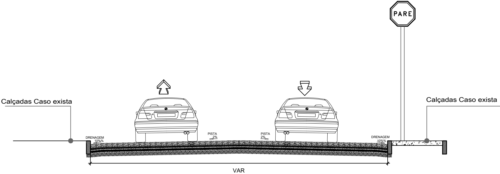
CORTE TRANSVERSAL - LUIZ FERREIRA SOBRINHO SEM ESCALA
