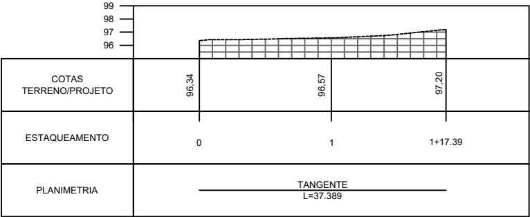
PERFIL KERGINALDO FERREIRA - PARTE 2
