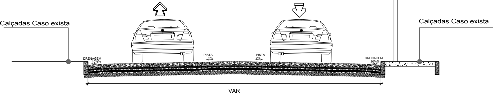
CORTE TRANSVERSAL - RUA FRANCISCO BATISTA SEM ESCALA
