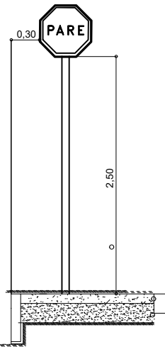
DETALHE DA PLACA DE SINALIZAÇÃO SEM ESCALA
