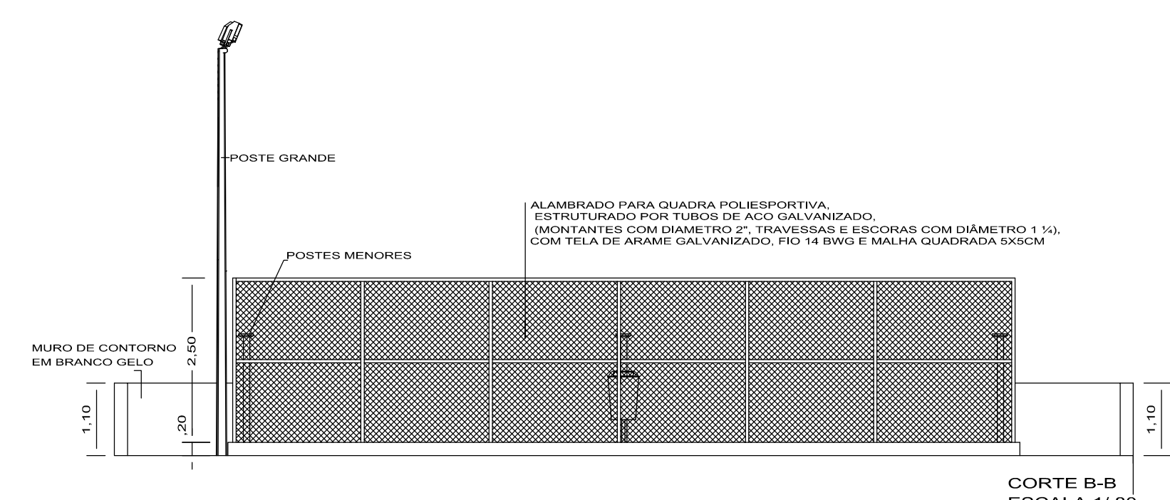
CORTE B-B ESCALA 1/ 80
