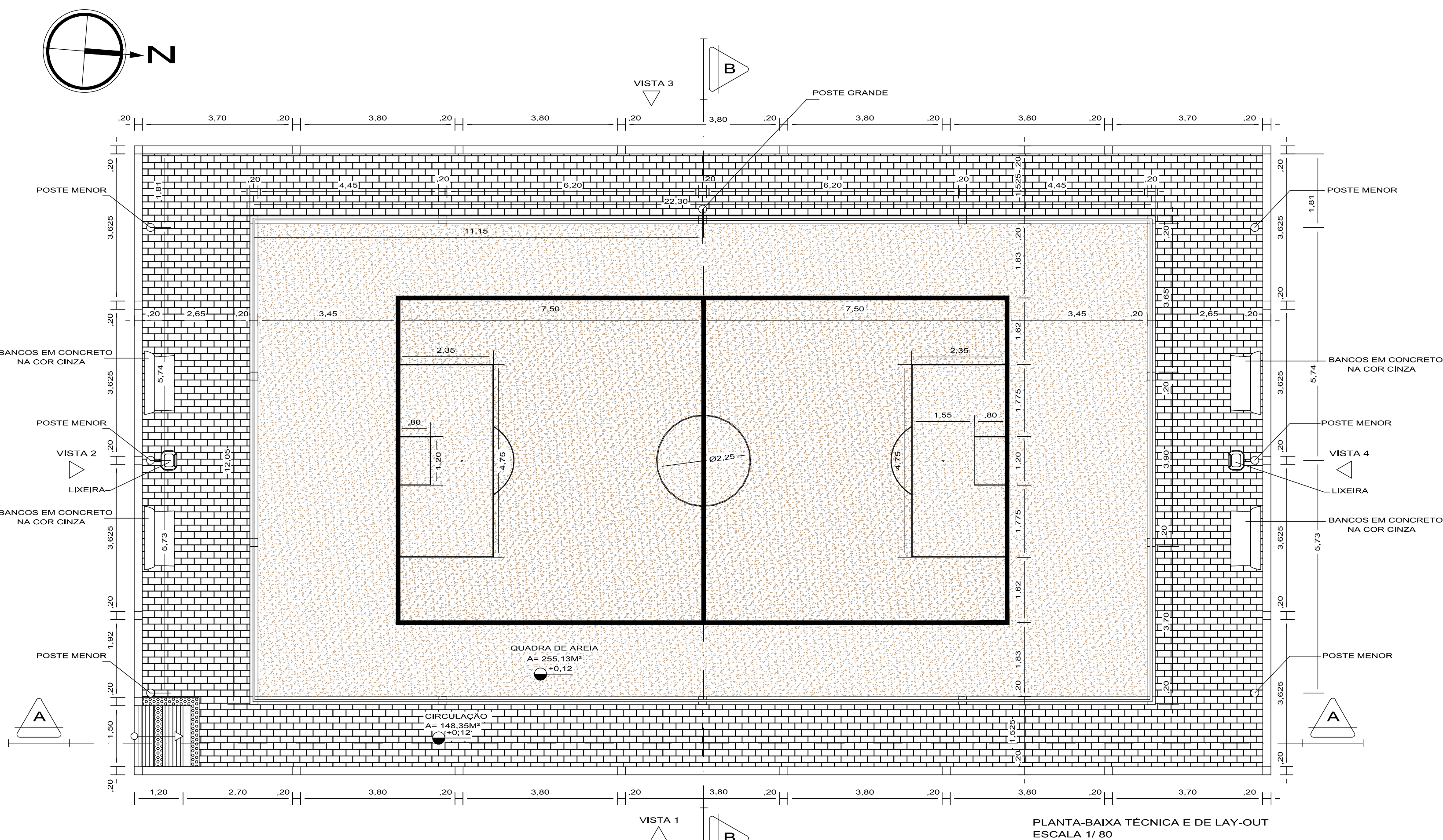
PLANTA-BAIXA T CNICA E DE LAY-OUT ESCALA 1/ 80
