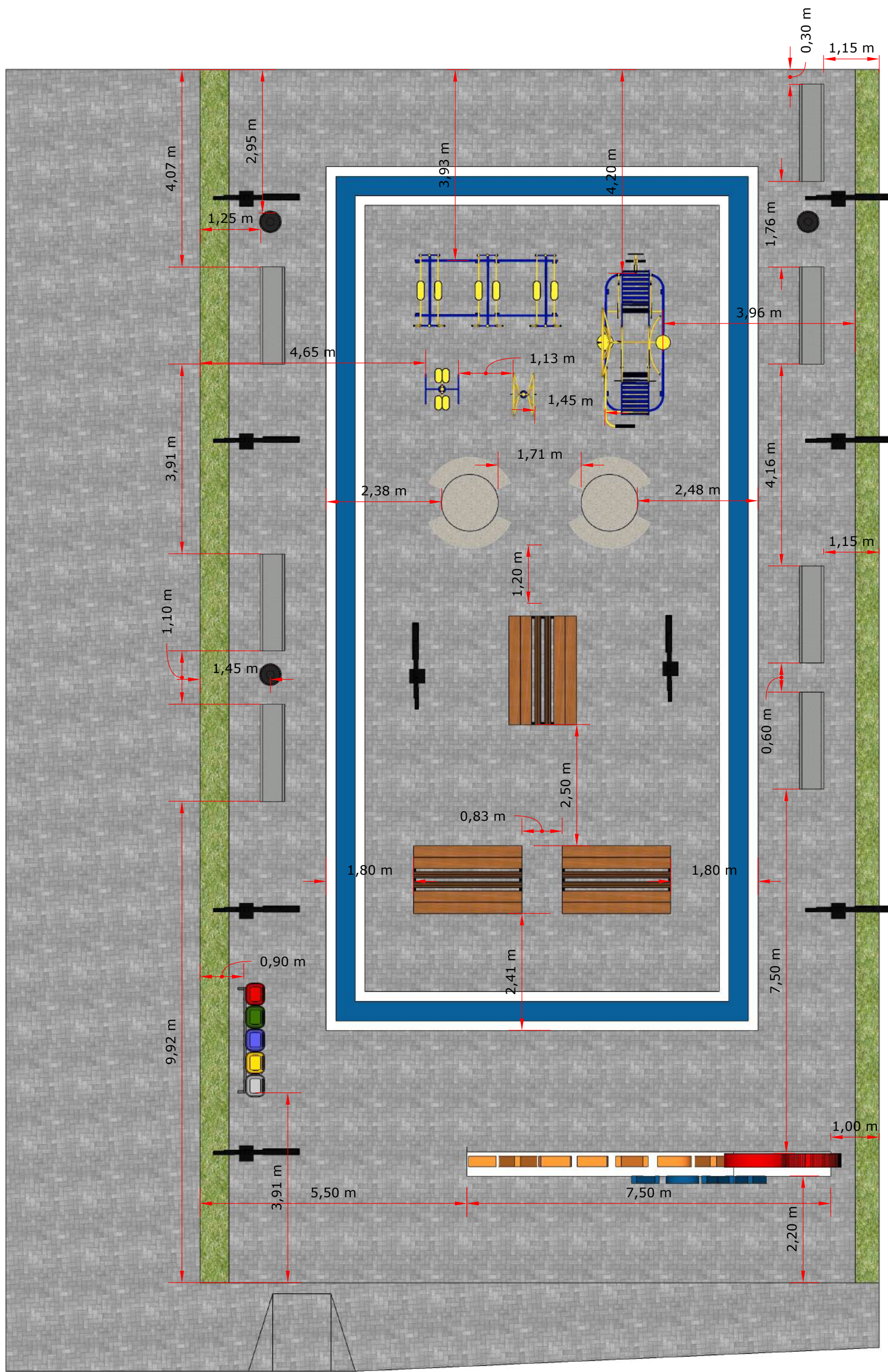
01 PLANTA BAIXA - MOBILIÁRIO URBANO ESCALA... 1/75
