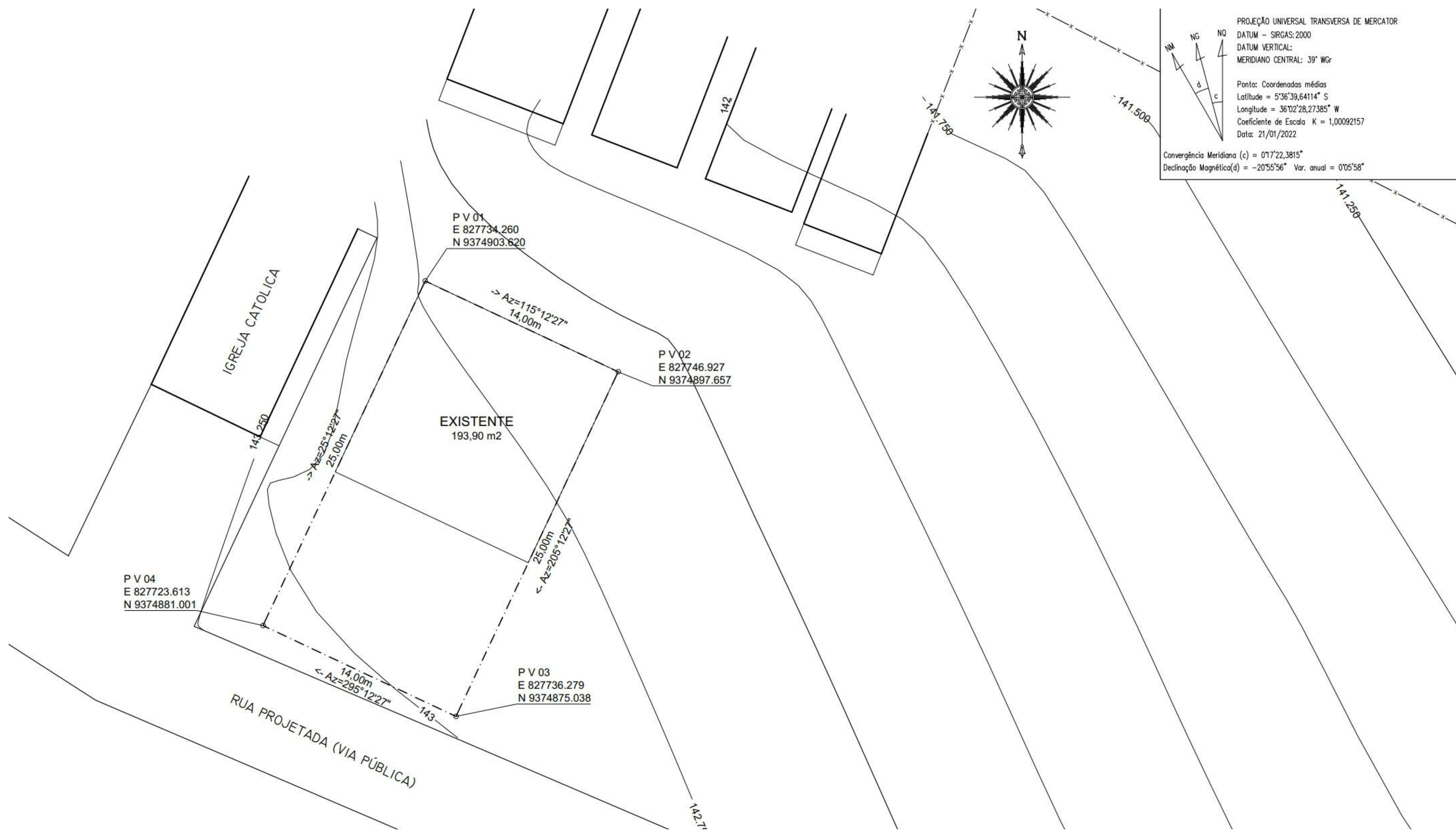
02 LEVANTAMENTO TOPOGRÁFICO SEM ESCALA
