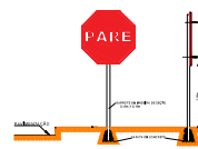
DETALHE DA PLACA "PARE" - R1 SEM ESCALA
