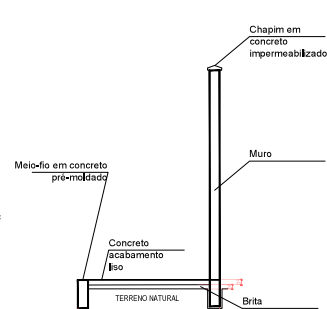
CORTE CALÇADA SEM ESCALA
