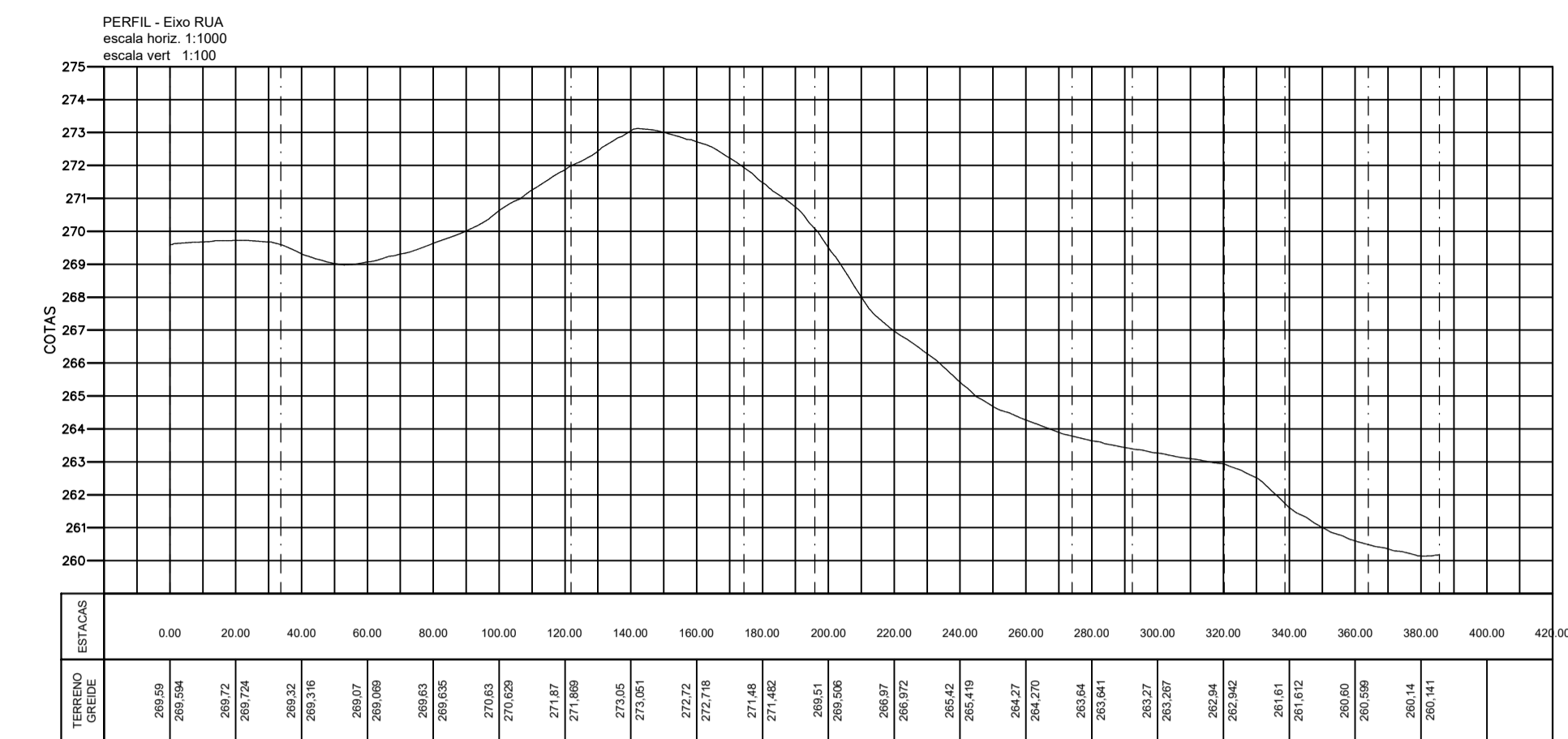
PERFIL TOPOGRÁFICO SEM ESCALA
