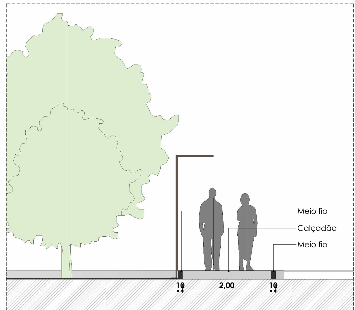
2 CORTE A 1 : 50
