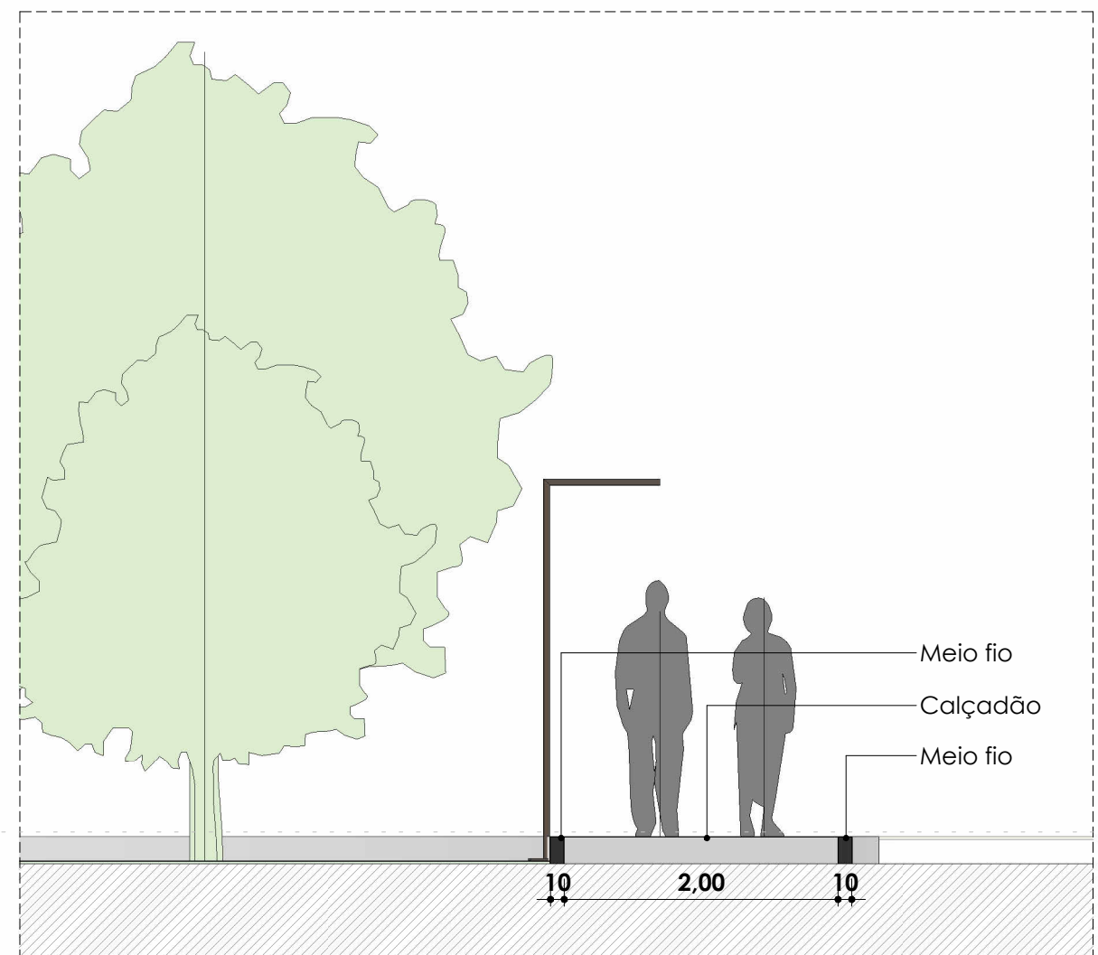
2 CORTE A 1 : 50
