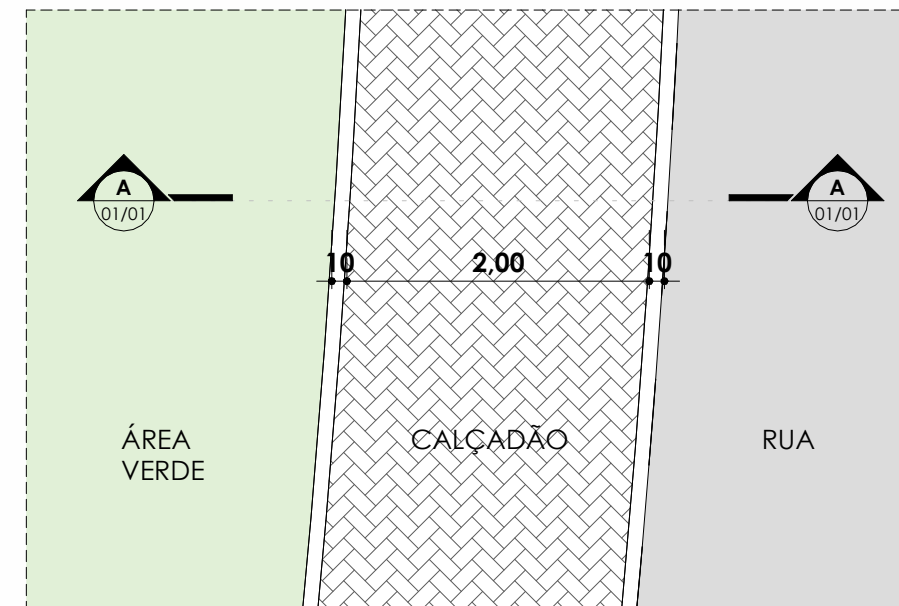
3 PLANTA BAIXA - PERCURSO 1 : 50
