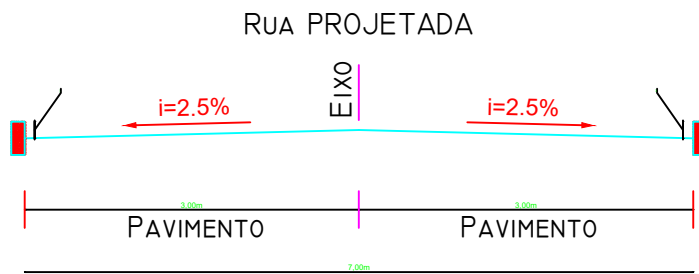
SEÇÃO TRANSVERSAL TIPO 5 / ESCALA
