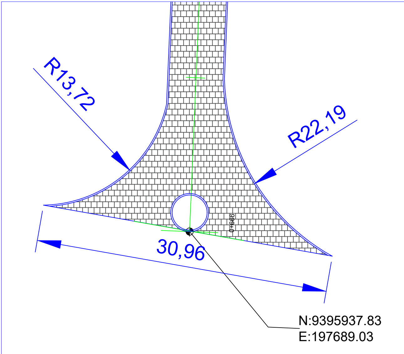
DETALHE 01 Escala 1:250
