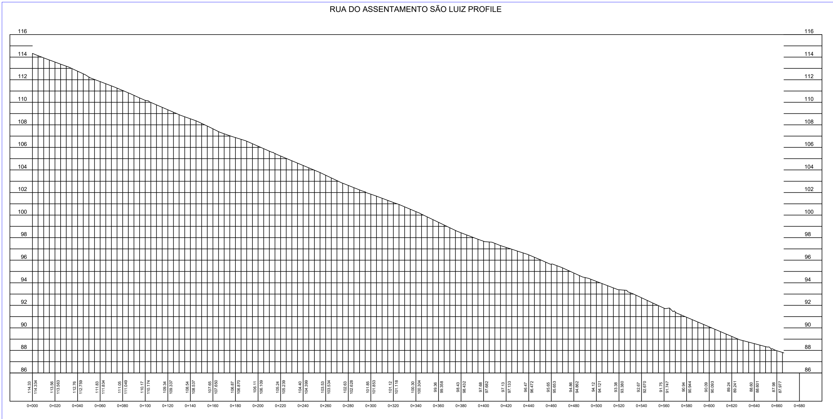
PERFIL DO TERRENO DA RUA DO ASSENTAMENTO SÃO LUIZ Escala 1:2000
