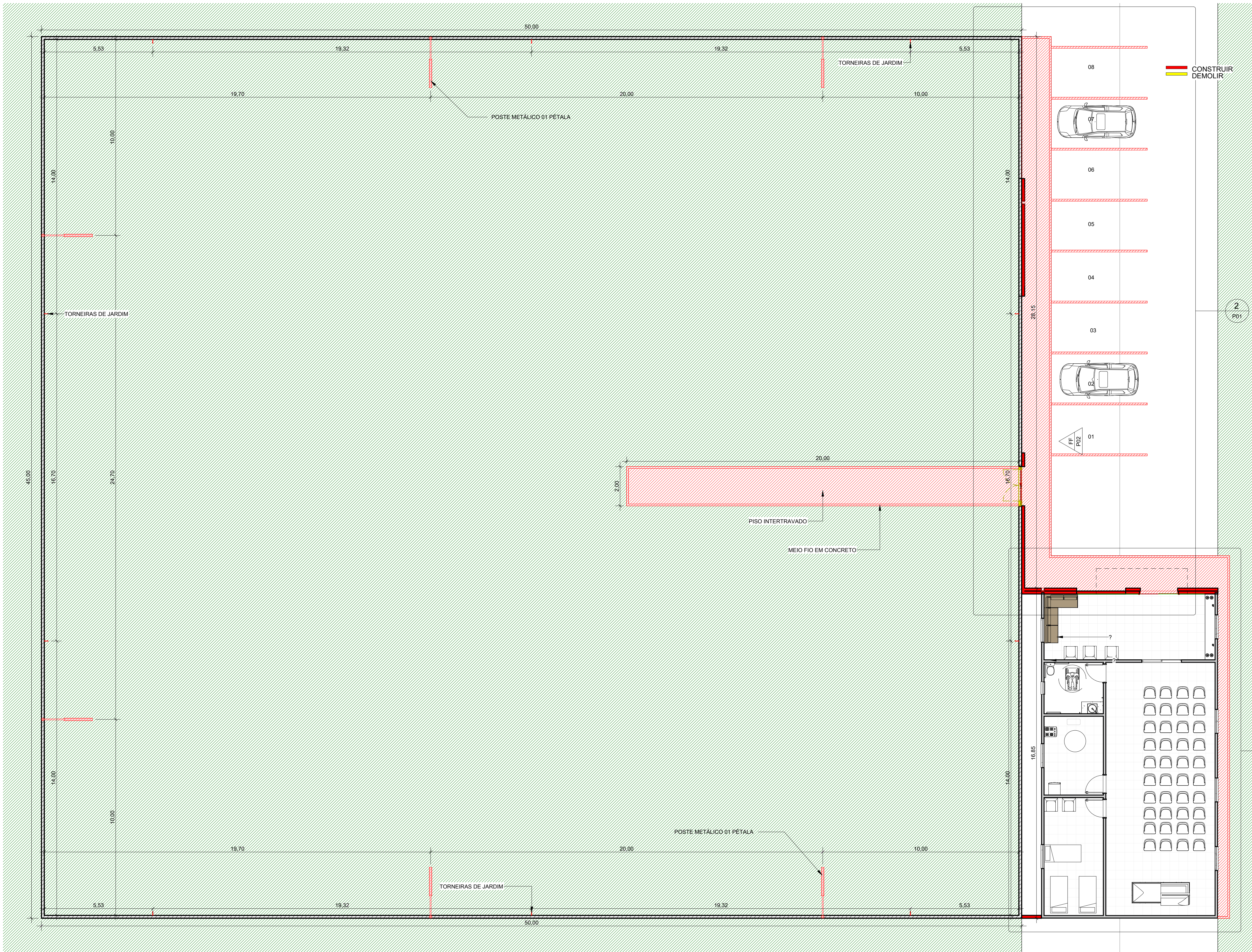
1 PLANTA BAIXA DE REFORMA 1 : 100
