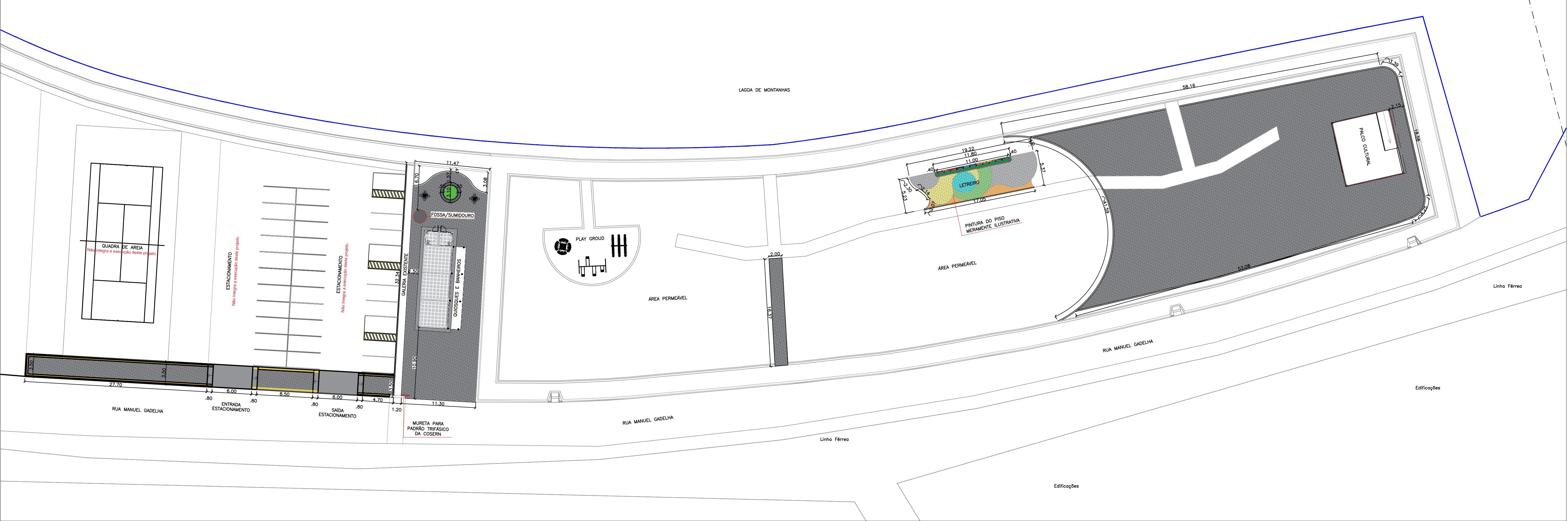
PLANTA BAIXA GERAL URBANIZAÇÃO DA LAGOA DE MONTANHAS esc. 1:300
