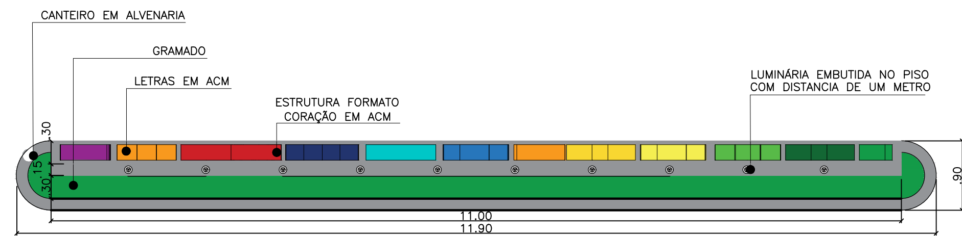
PLANTA BAIXA LETREIRO esc. 1:50
