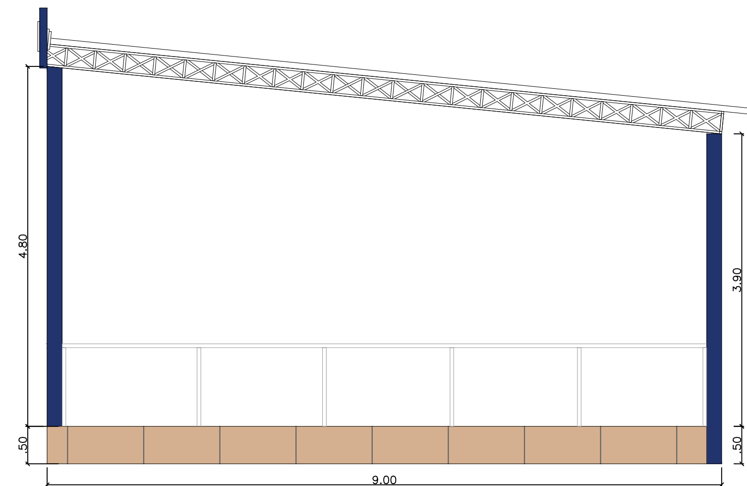
VISTA LATERAL 1 - PALCO CULTURAL esc 1:50
