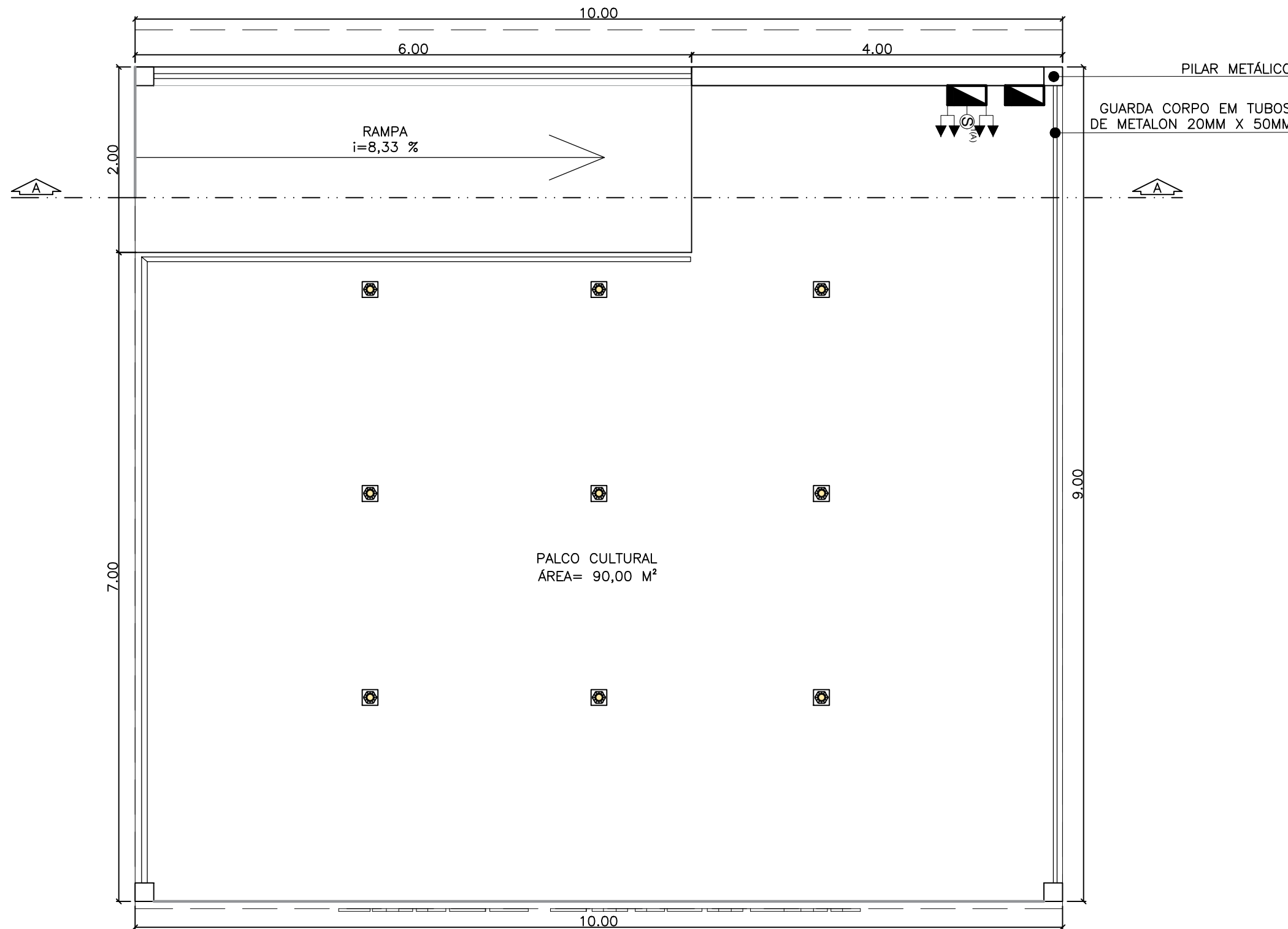
PLANTA BAIXA PALCO CULTURAL esc 1:50
