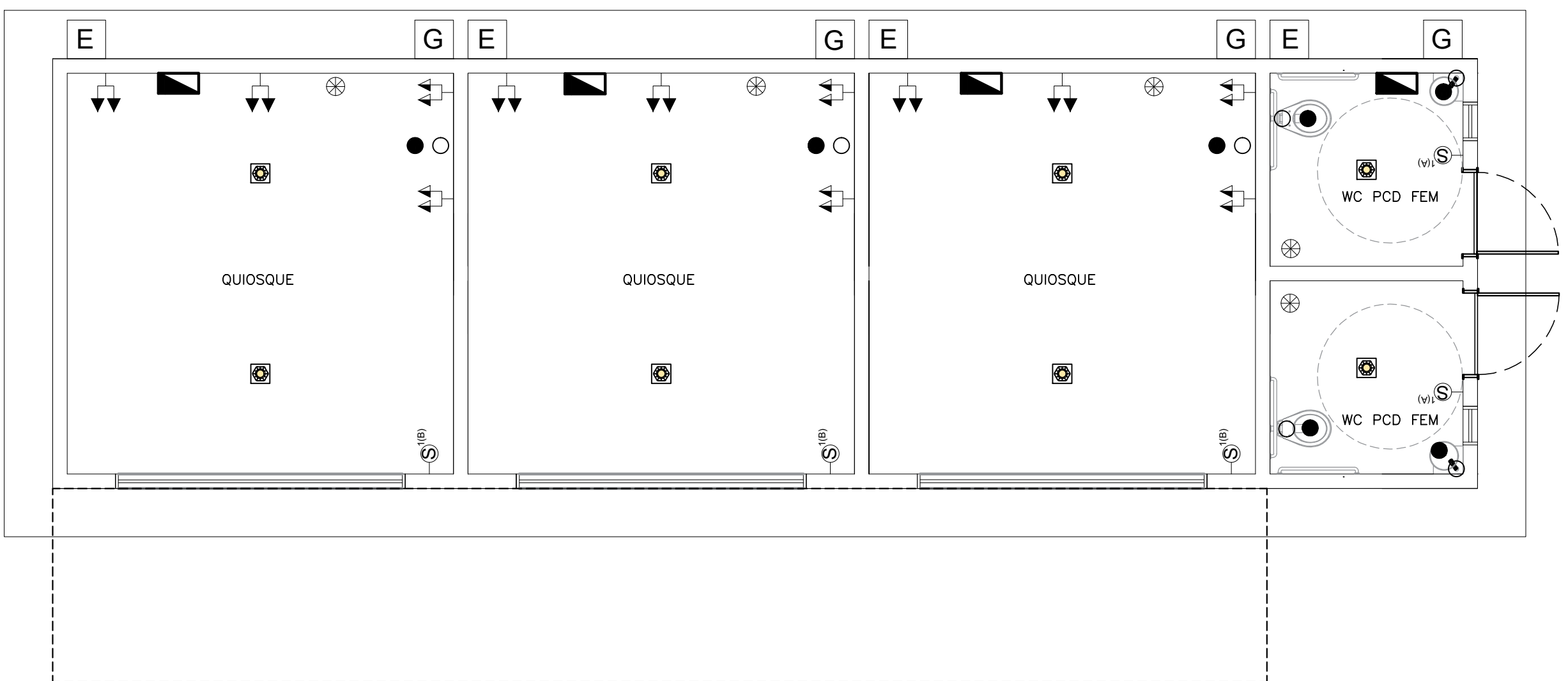
PLANTA DE PONTOS ELÉTRICOS E HIDRÁULICOS
