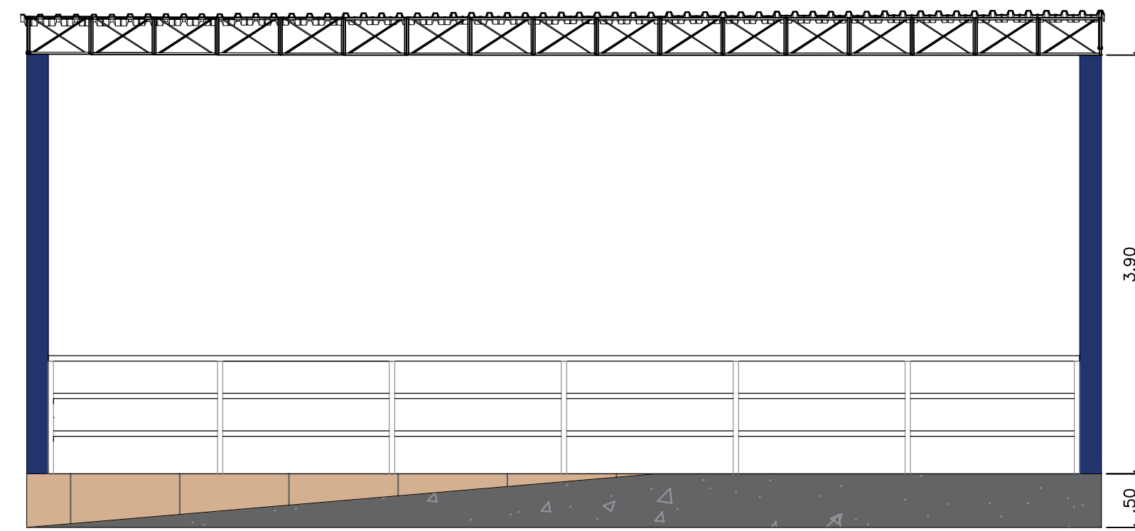
CORTE AA - PALCO CULTURAL esc 1:50
