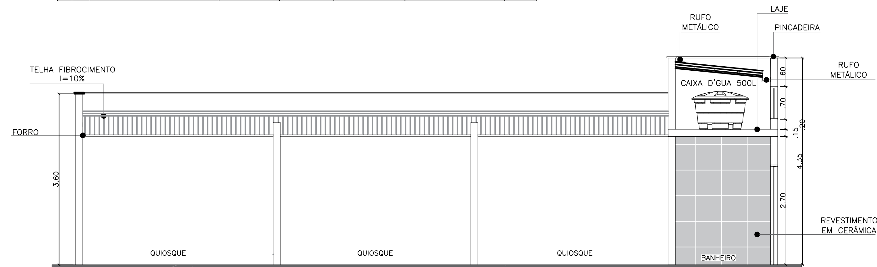
CORTE AA
