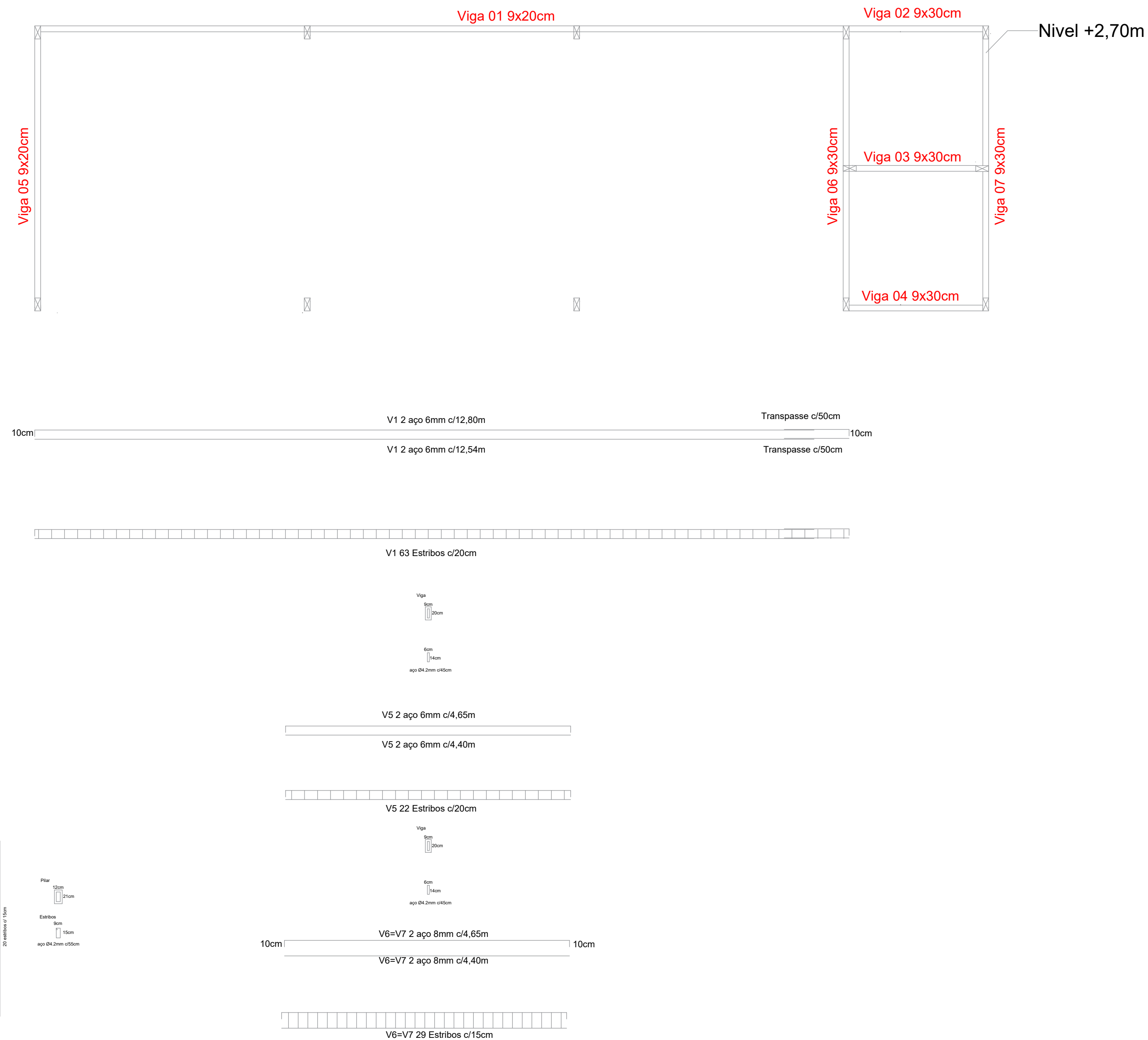
Planta de viga térreo
