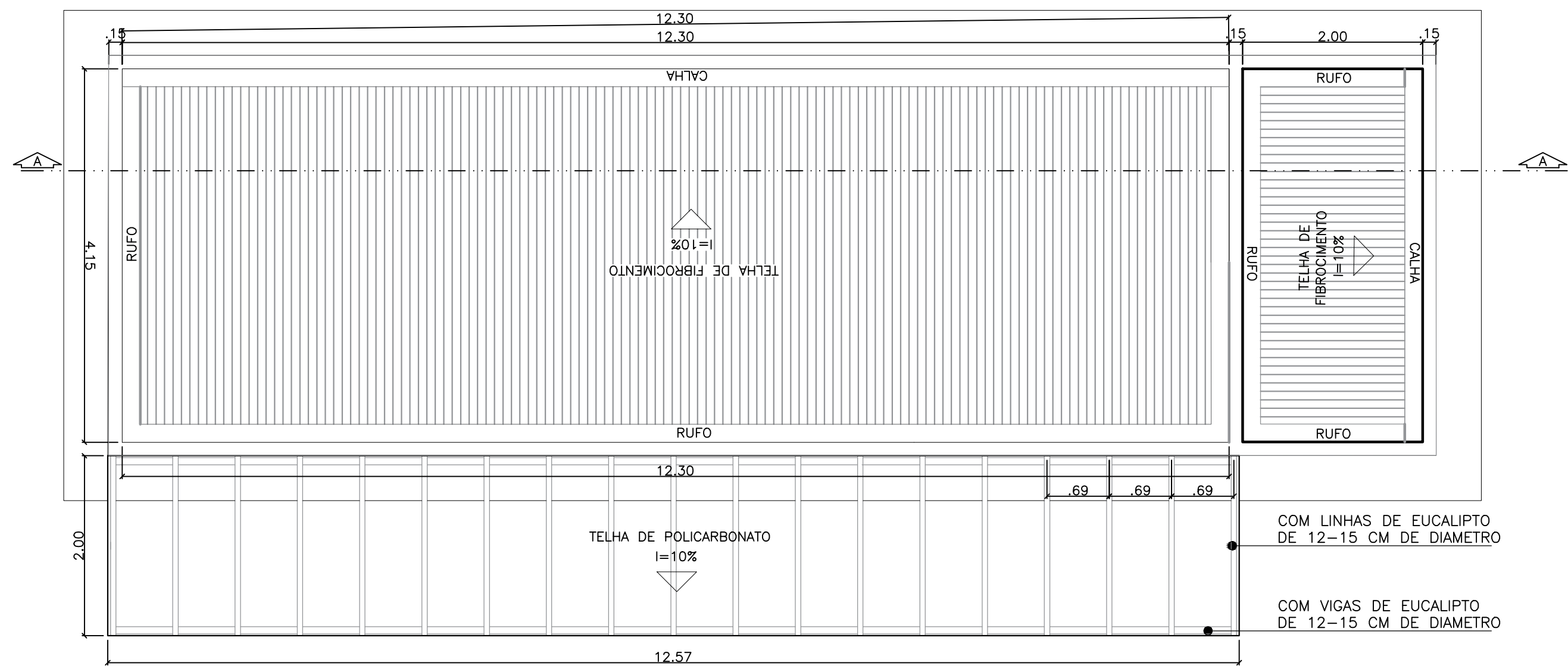
PLANTA DE COBERTA QUIOSQUE
