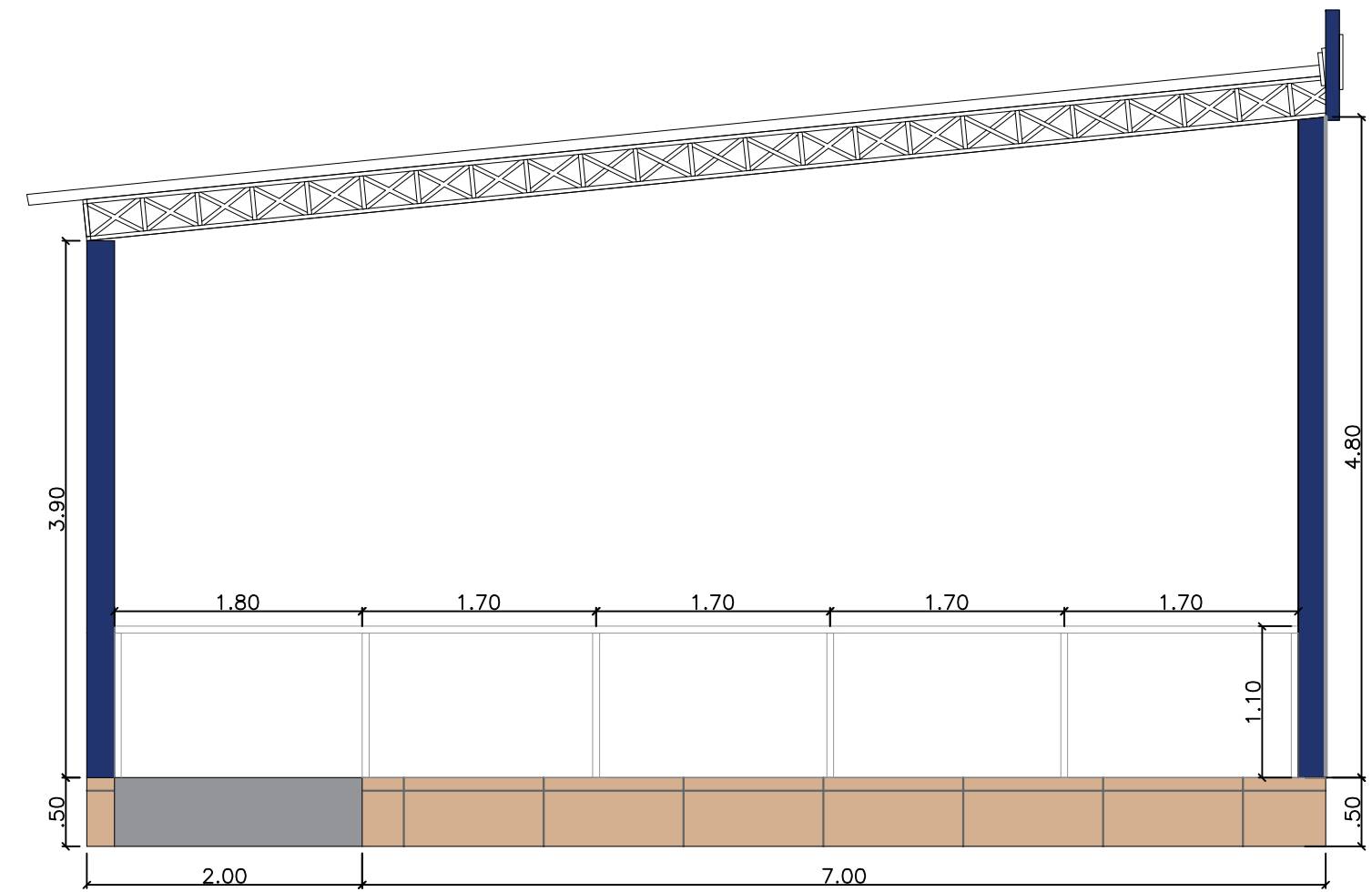
VISTA LATERAL 2 - PALCO CULTURAL esc 1:50
