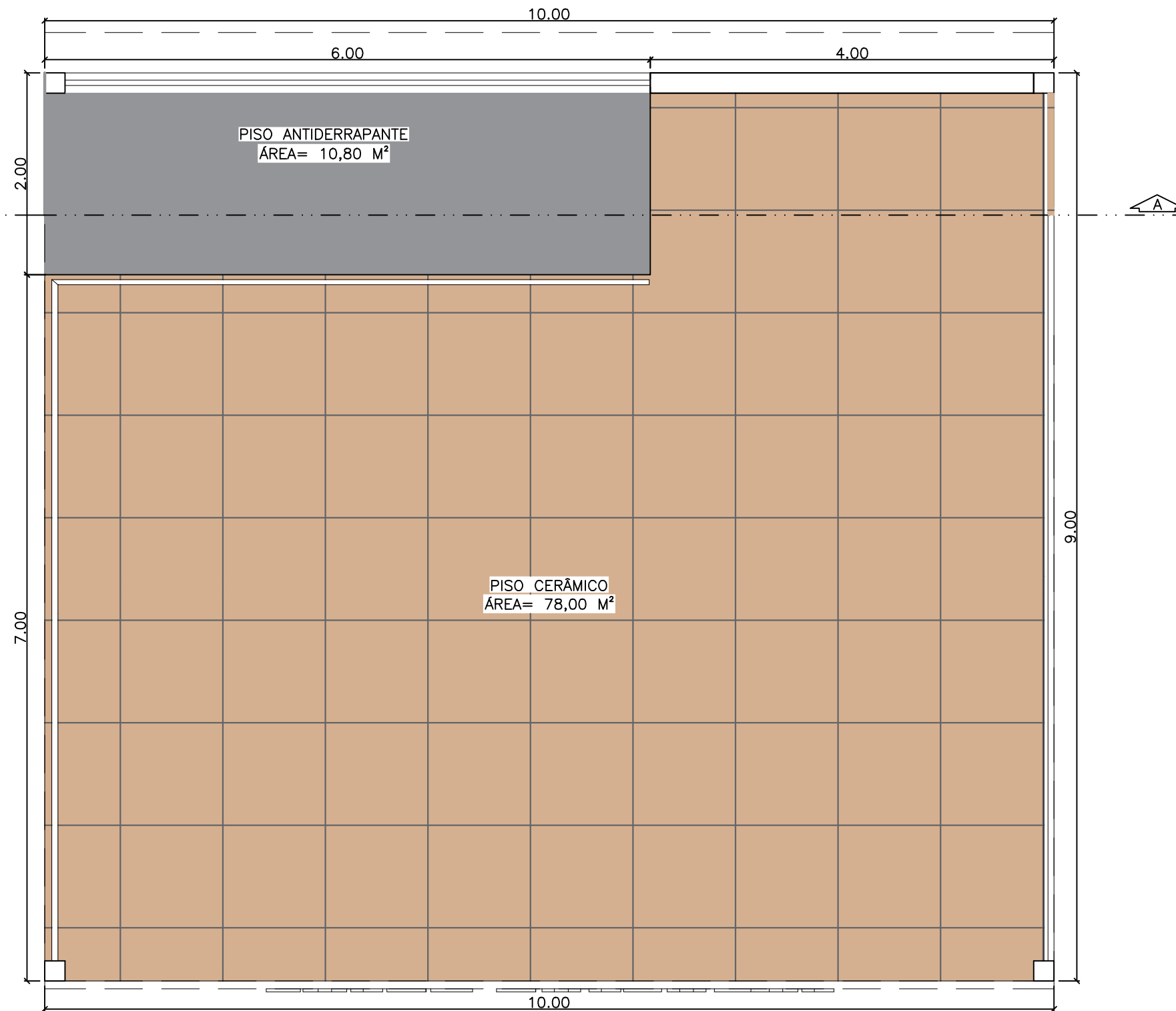
PLANTA DE PISO - PALCO CULTURAL esc 1:50
