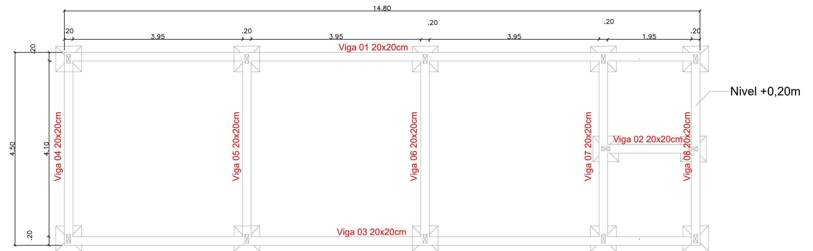
Planta de vigas baldrame dos quiosque
