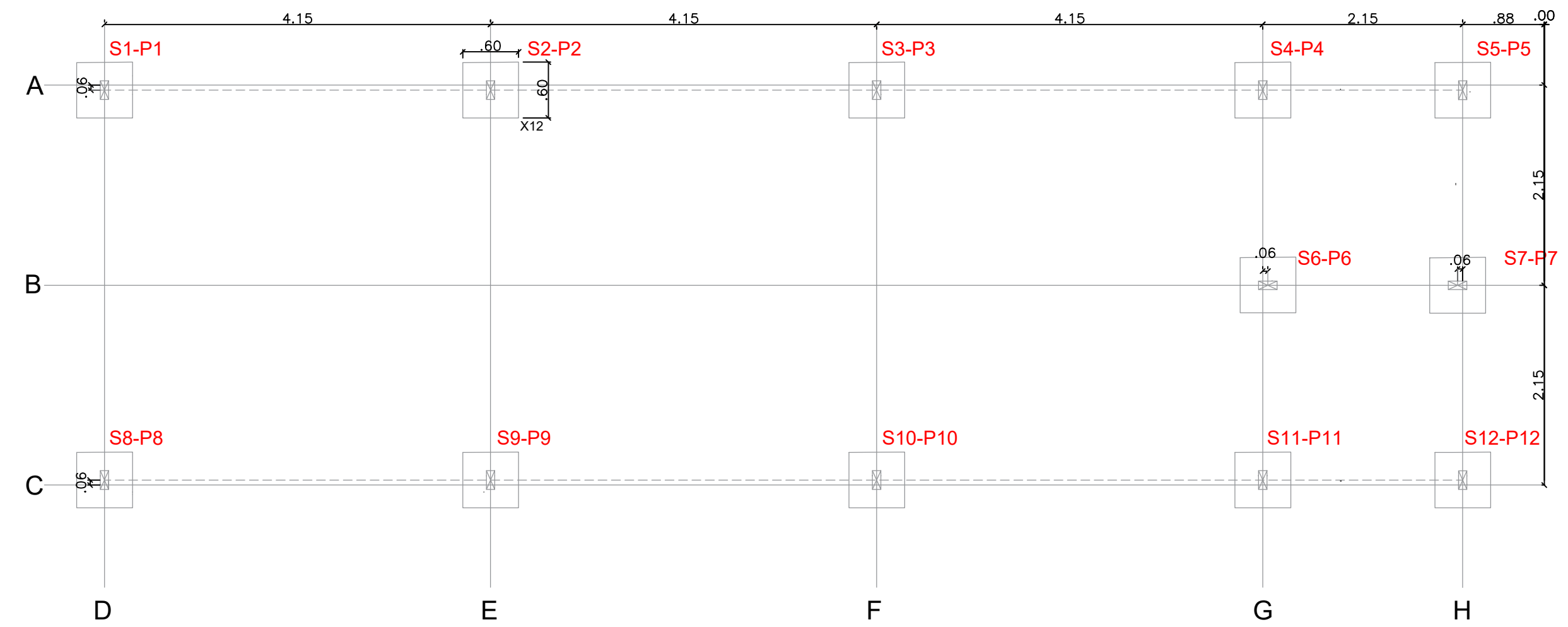
Planta de locação e pilares dos quiosque
