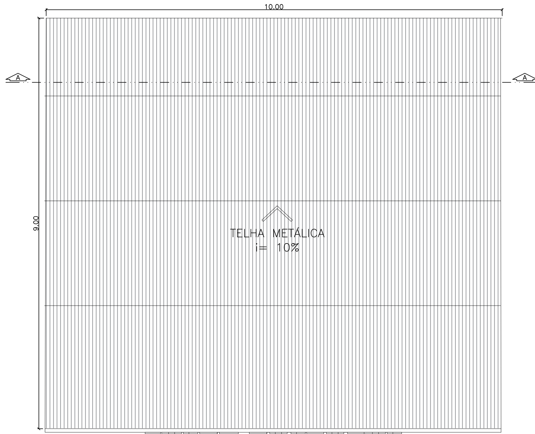
PLANTA DE COBERTA PALCO CULTURAL esc 1:50
