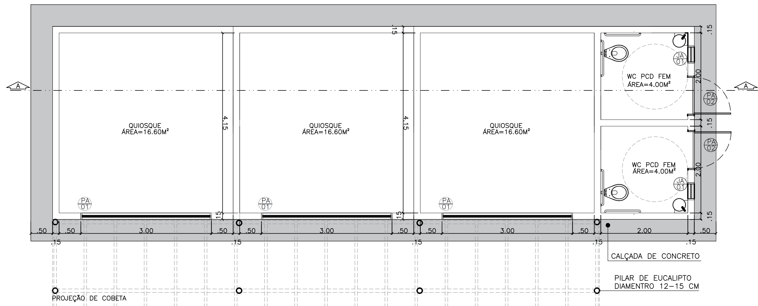
PLANTA BAIXA TÉCNICA QUIOSQUE
