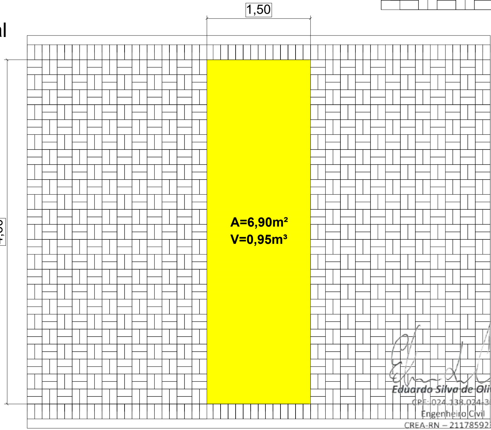
Detalhe lombada visto de cima
