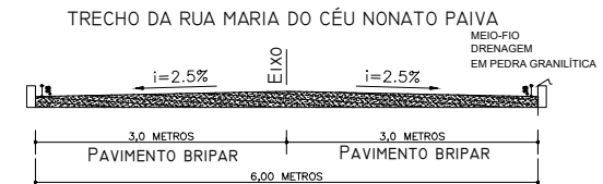
SEÇÃO TRANSVERSAL TIPO
