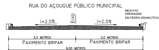
SEÇÃO TRANSVERSAL TIPO
