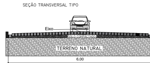
SEÇÃO TRANSVERSAL TIPO
